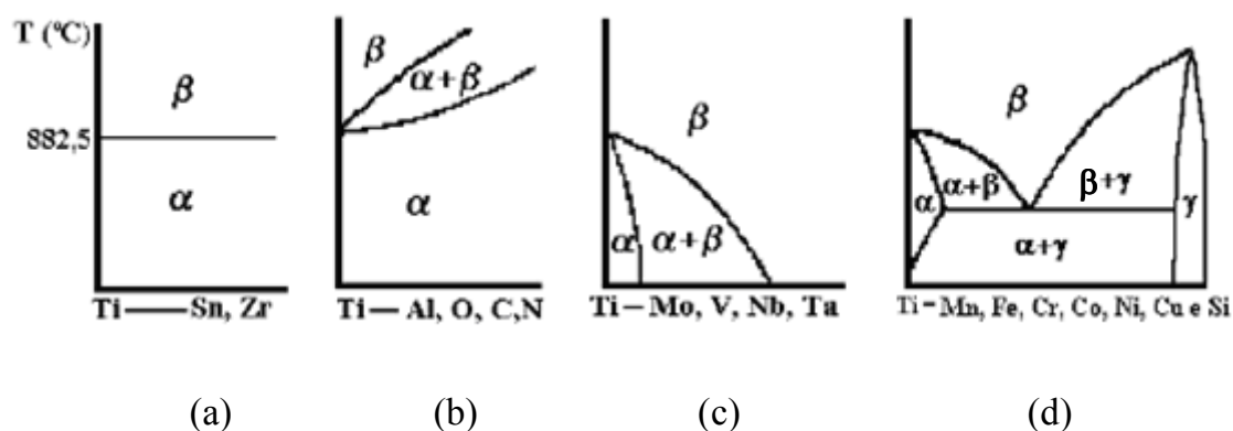
Figura 12 – Diagramas de fase binários das ligas de titânio: (a) elementos neutros, (b) elementos alifagênicos, (c) elementos \beta -isomorfos, (d) elementos \beta -eutetóides (SANTOS, 2006).
