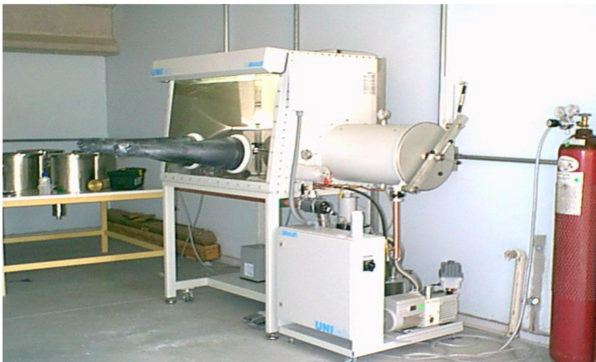
Figura 23 – Fotografia. Vista geral da câmara de gás inerte (glove box) utilizada para a manipulação dos materiais.
