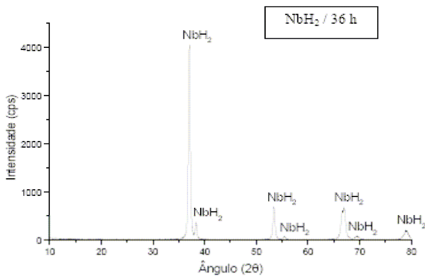
Figura 16 – Difratoograma de raios X dos pós de NbH 2 , moídos por 36h (SANTOS, 2006).
