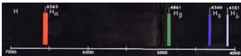
Figura 4 – Faixas luminosas que correspondem ao espectro visível do átomo de hidrogênio ( www.google.com.br/imagens ).
