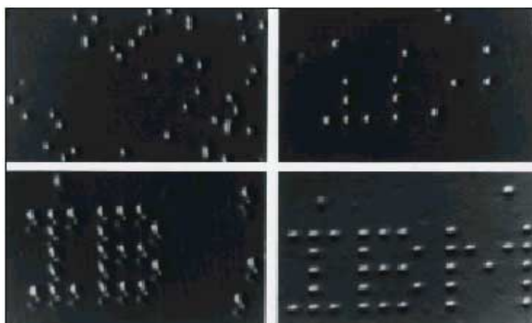
Figura 2 – Logotipo da IBM formado por 35 átomos de xenônio posicionados sobre uma superfície de níquel (CHAVES, 2002).
