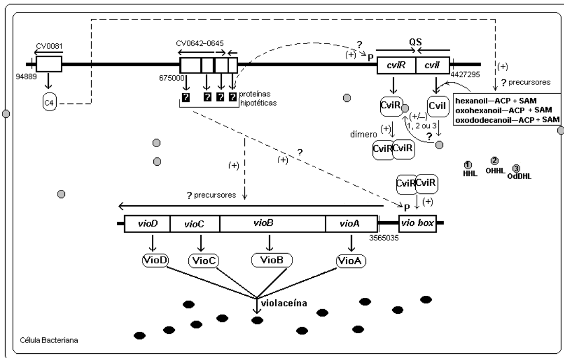
Figura 5.34. Modelo hipotético para o controle positivo da produção de violaceína em ATCC 12472. Os números 1, 2 e 3 indicam os três tipos de AHL identificados na linhagem selvagem de C. violaceum . Assume-se que CviI seja capaz de sintetizar os três tipos de moléculas. QS: Quorum sensing . P: região promotora. As linhas tracejadas representam algumas das possíveis formas de regulação. A representação da posição dos genes não está em escala, mas os números indicam a posição e a distância entre os genes no genoma de C. violaceum .
