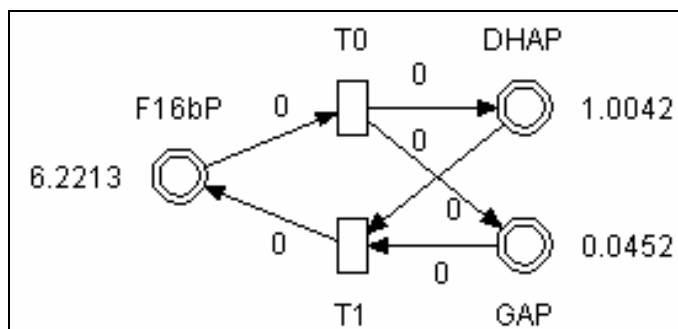
Figura 3.11 Estrutura da rede de Petri híbrida para a reação catalisada pela enzima frutose-1,6-bisfosfato aldolase.
