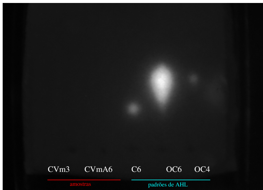
Figura 5.18. Identificação de AHL de cadeia curta a partir da extração do sobrenadante das culturas mutantes de C. violaceum (CVm3 e CVmA6). Padrões: C6: HHL; OC6: OHHL; OC4: OBHL. Biossensor: pSB401.
