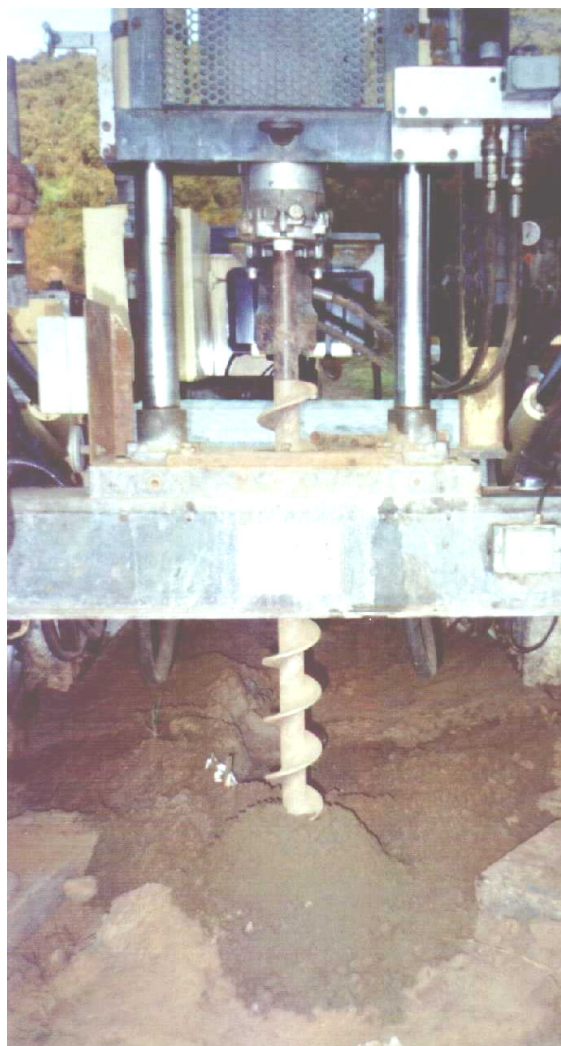
Figura 4.15 – Execução do pré-furo na bermas de alteamento da Barragem de Gongo Soco
