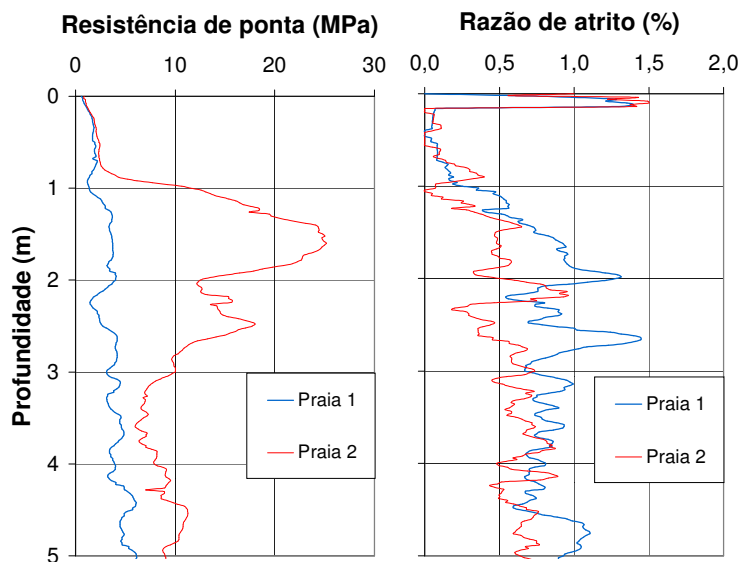
Figura 5.25 – Perfil integrado da resistência de ponta corrigida e da razão de atrito dos ensaios PraiaCG1 e PraiaCG2 (1)
