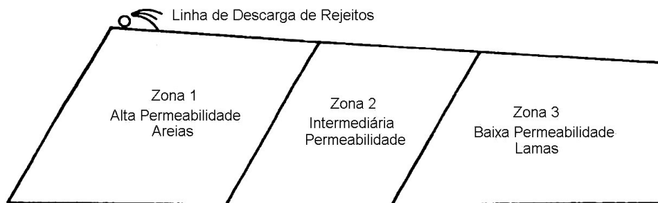
Figura 7.1 – Variação da condutividade hidráulica em um depósito de rejeitos (SANTOS, 2004)
