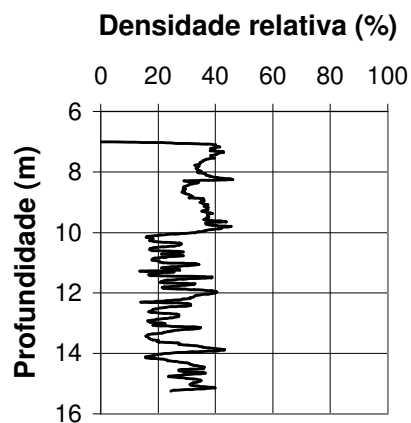
Figura 6.7 – Perfil da densidade relativa do ensaio CristaGS1 Proposta de KULHAWY & MAYNE (1990)
