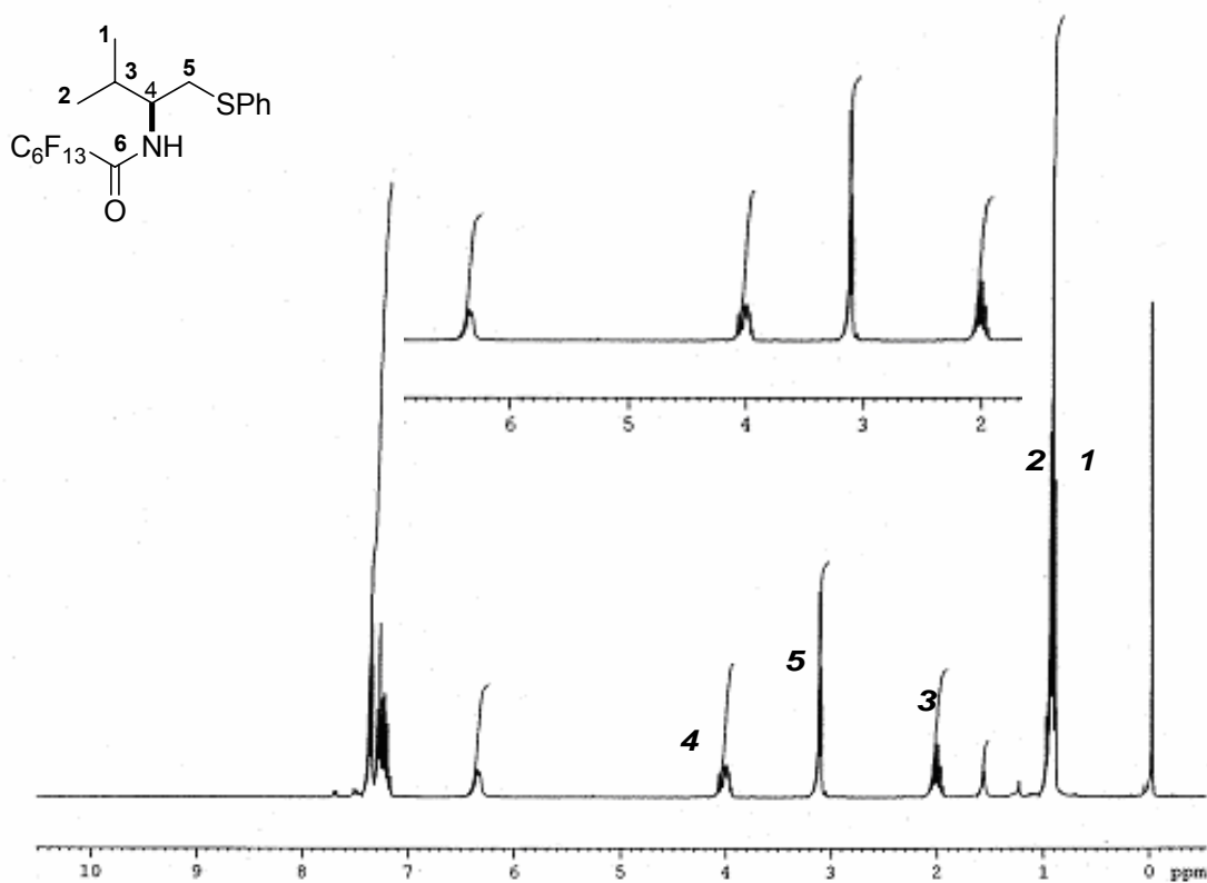
Figura 20. Espectro de RMN a 300 MHz, em CDCl 3 , do composto 22 .
