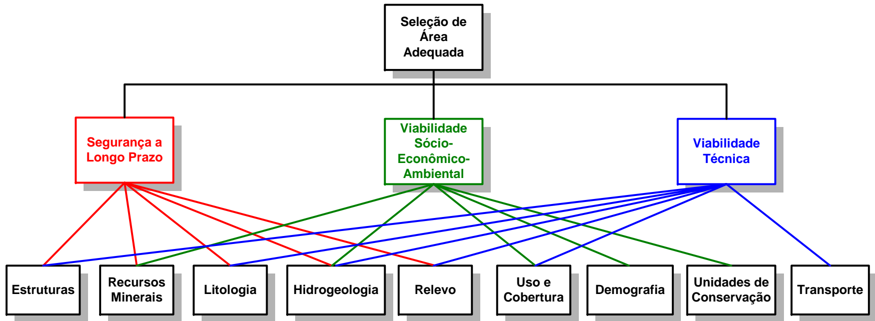
Figura 4.1 – Estrutura Hierárquica
