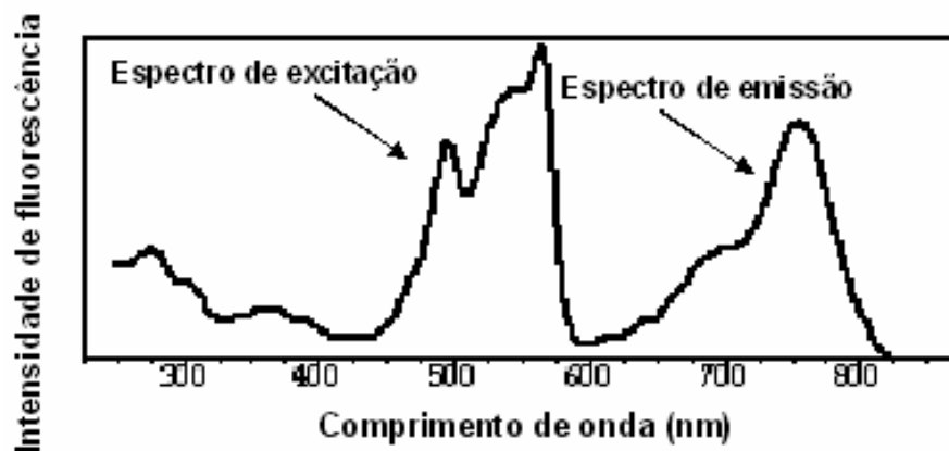
Figura 1.13: Espectro de excitação e emissão do fluorocromo R-PECy7. Fonte: Adaptado do site http://www.drmr.com/abcon/C7Paspec.html .
