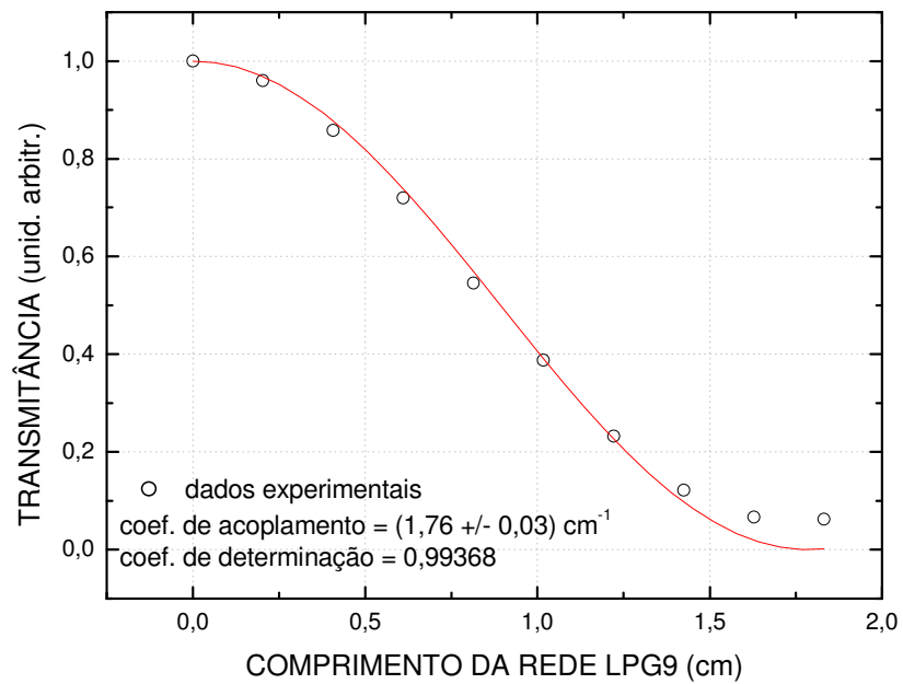
Determinação do coeficiente de acoplamento da LPG9
