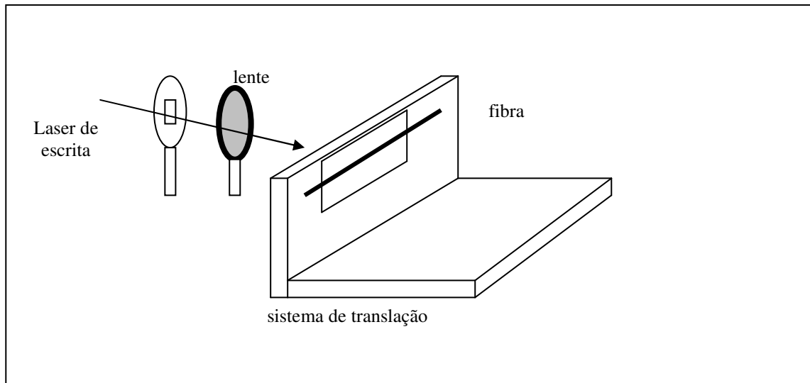
Figura 9: Técnica de escrita ponto-a-ponto (MALO, HILL, BILODEAU et al , 1993).
