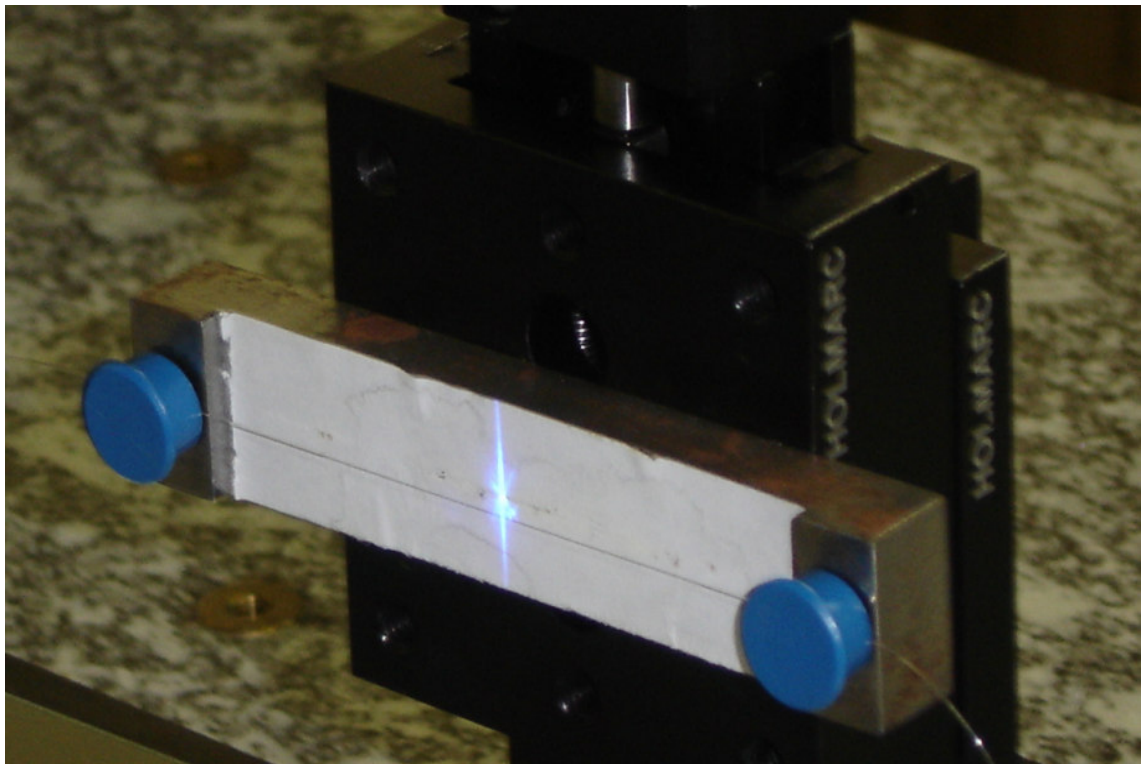
Figura 46: Foto do suporte de gravação das LPGs, observando-se a figura de iluminação resultante da difração formada pela incidência do feixe UV sobre a fibra ótica desencapada.
