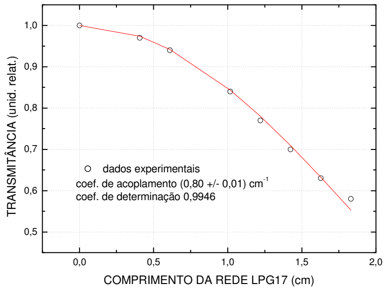
Determinação do coeficiente de acoplamento da LPG17
