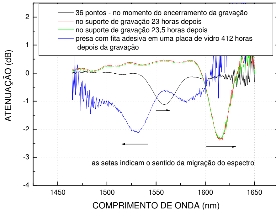
Figura 49: Evolução espectral da LPG13 (gravada em fibra “Nuferr”) depois da gravação.
