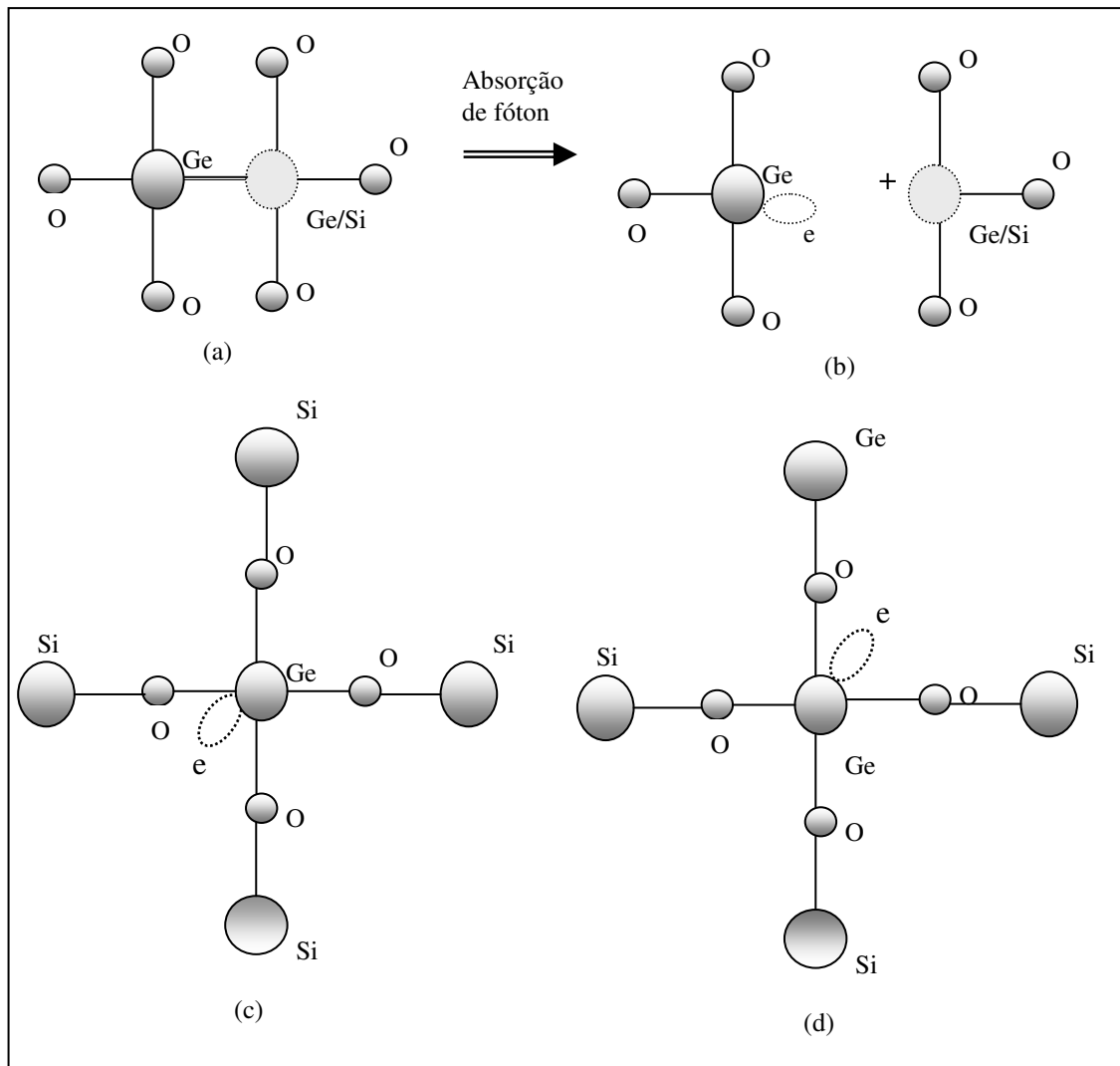
Figura 2: Defeitos associados à dopagem com Ge: (a) Centro \text{GeO} ou \text{GODC} , (b) defeito ionizado \text{GeE}' , (c) \text{Ge}(1) e (d) \text{Ge}(2) (KASHYAP, 1999).
