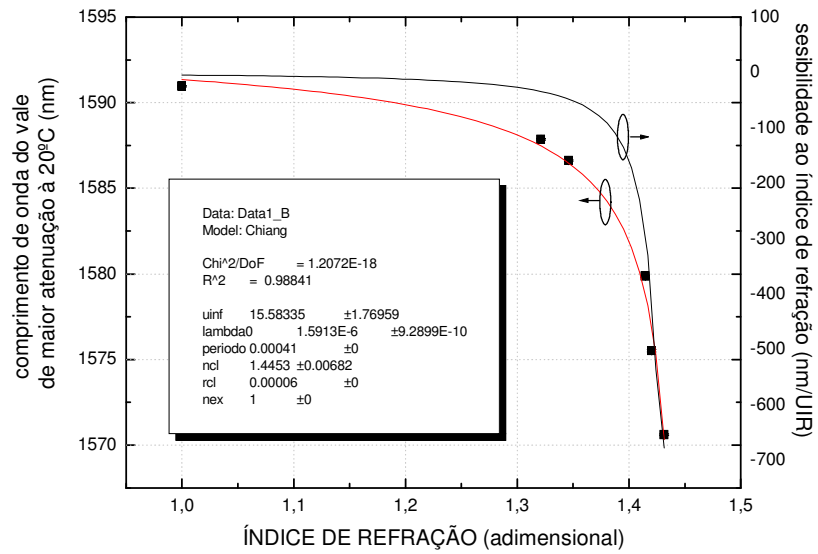
Ajuste da Equação de Chiang na LPG2
