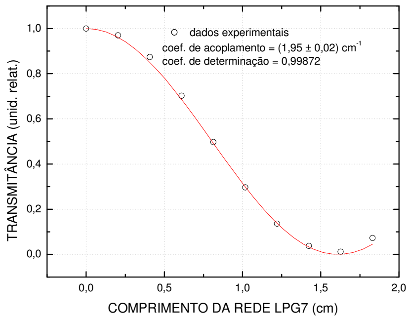
Determinação do coeficiente de acoplamento da LPG7
