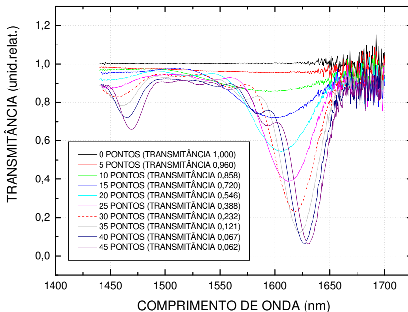
Razão espectral entre os sinais transmitidos pela LPG9 (fibra “Centaurus”), durante a gravação, e o sinal emitido pela fonte ótica LED.
