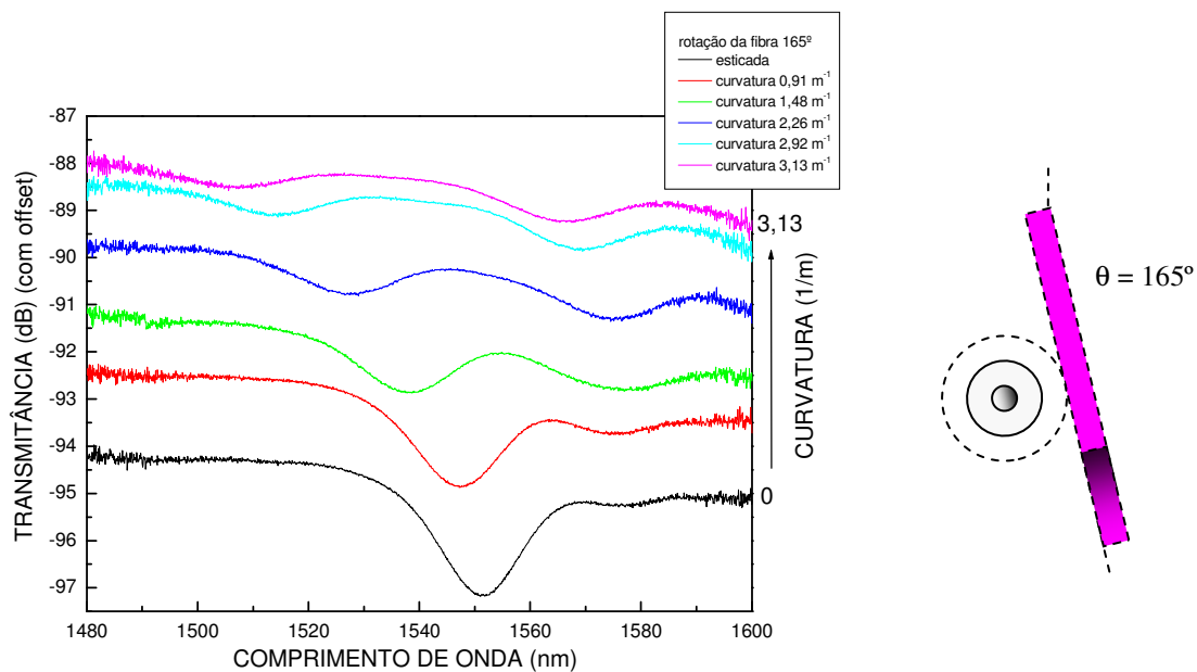
Resposta espectral da LPG20 submetida à curvaturas quando rotacionada de 165°.
