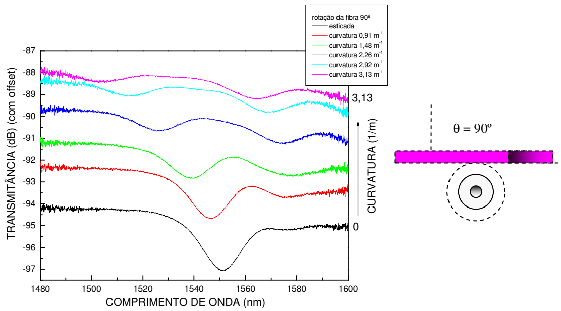
Resposta espectral da LPG20 submetida à curvaturas quando rotacionada de 90°.
