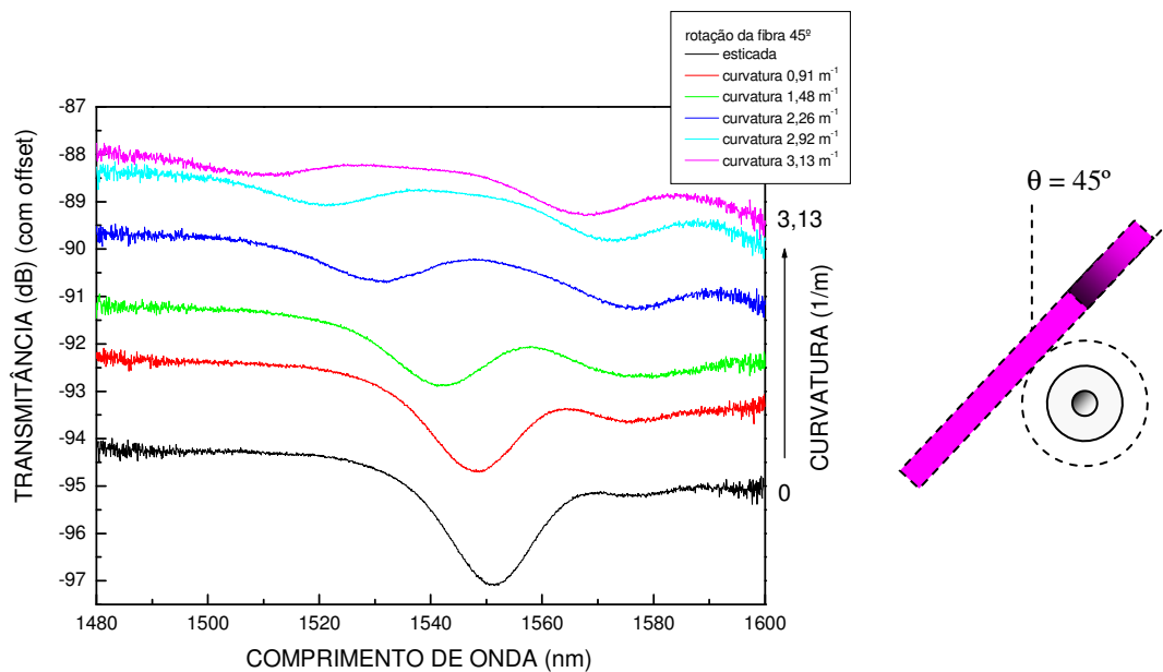
Resposta espectral da LPG20 submetida à curvaturas quando rotacionada de 45°.
