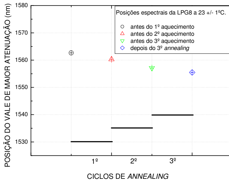
Figura 70: Deslocamentos espectrais do maior vale de atenuação da LPG8 ao longo dos três ciclos de “ annealing ”.
