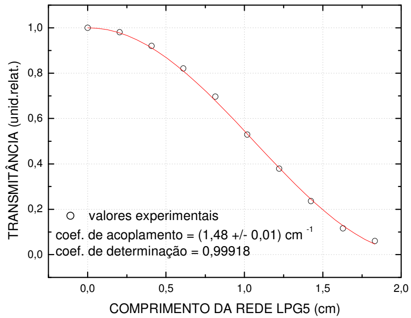
Determinação do coeficiente de acoplamento da LPG5
