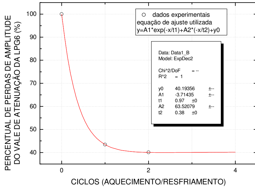
Figura 76: Ajuste exponencial da evolução das perdas percentuais de amplitude da LPG6 em função dos ciclos de “ quenching ”.
