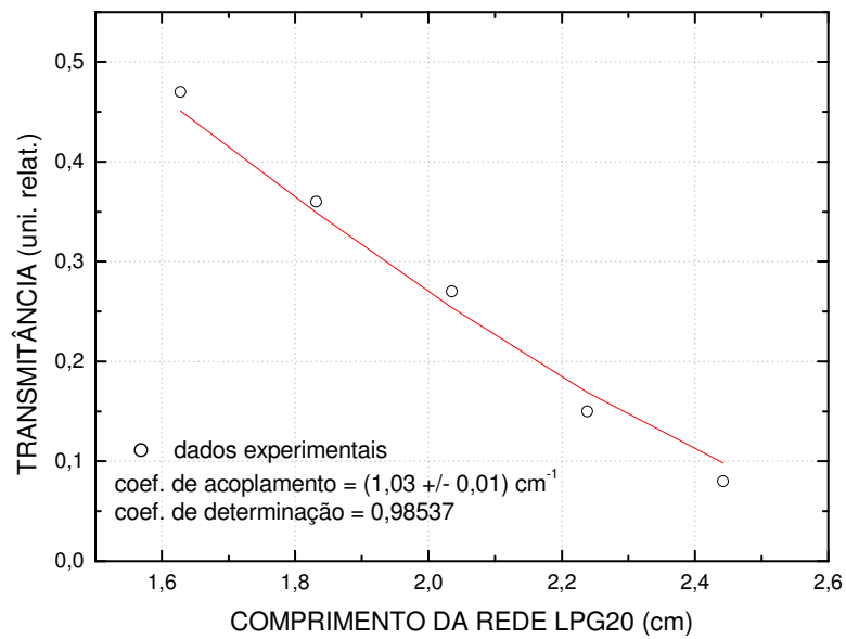
Determinação do coeficiente de acoplamento da LPG20
