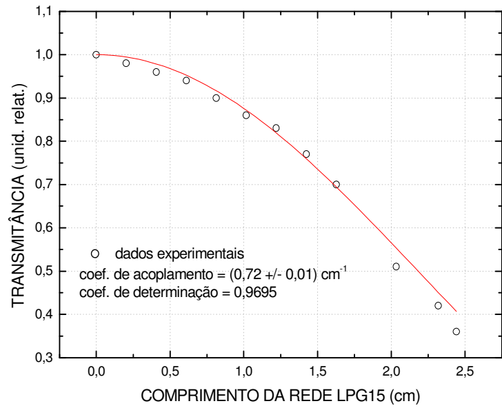
Determinação do coeficiente de acoplamento da LPG15
