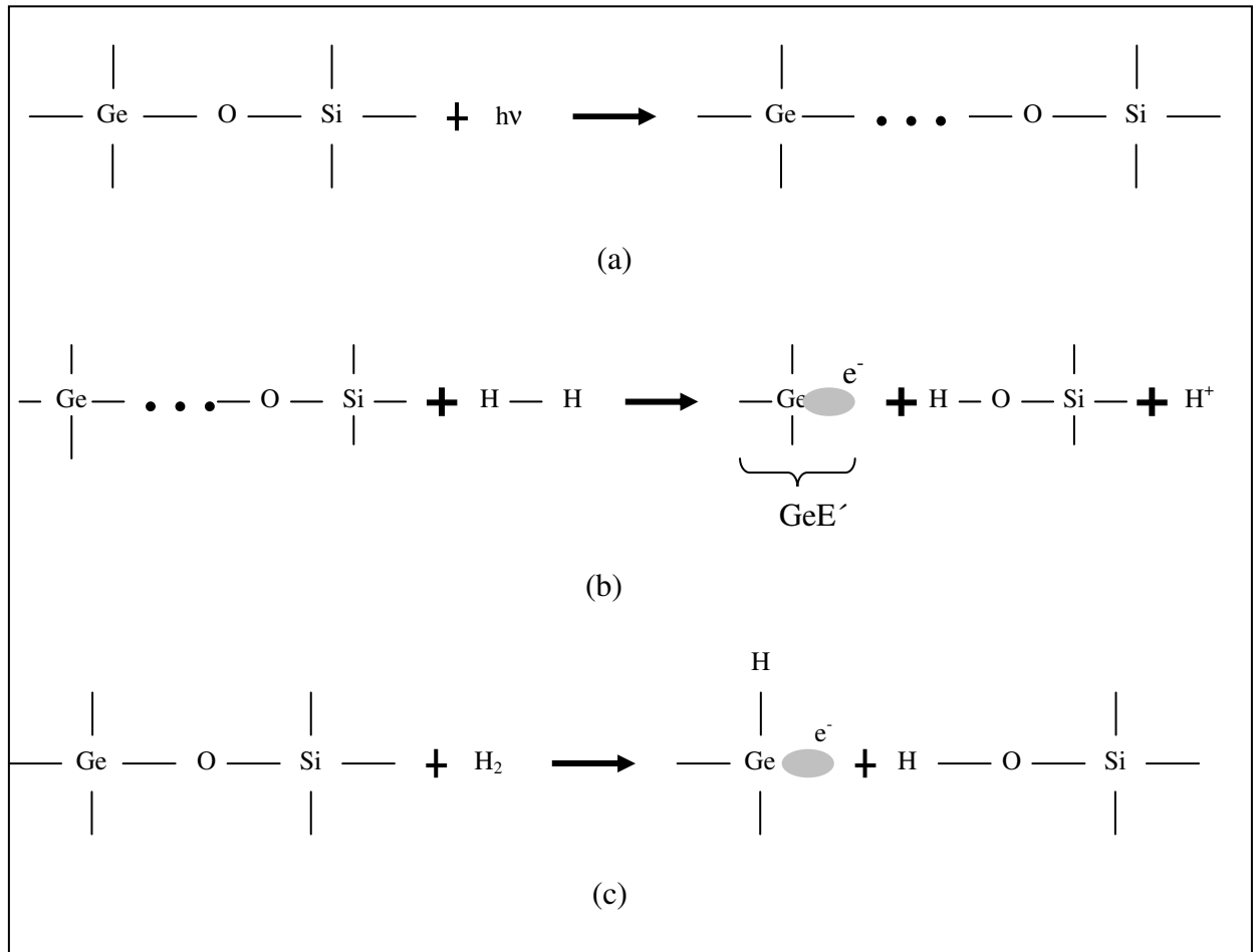
Figura 3: Reação química para a formação dos íons GeH e OH em fibras hidrogenadas (GRUBSKY, STARODUBOV e FEINBERG, 1999).
