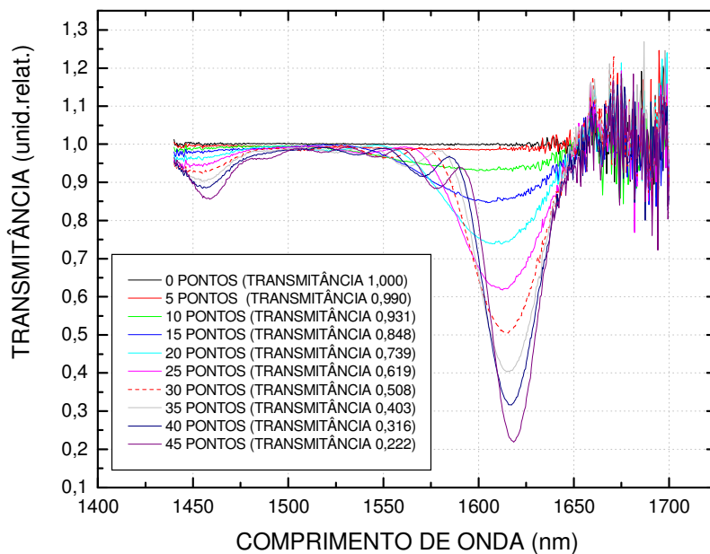
Razão espectral entre os sinais transmitidos pela LPG8 (fibra “Centaurus”), durante a gravação, e o sinal emitido pela fonte ótica LED.
