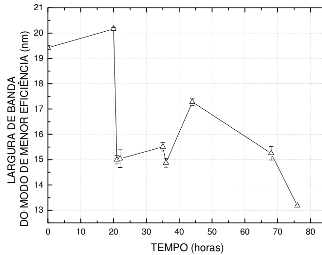
Figura 53: Acompanhamento da largura de banda da banda de menor eficiência da LPG9 após a gravação.
