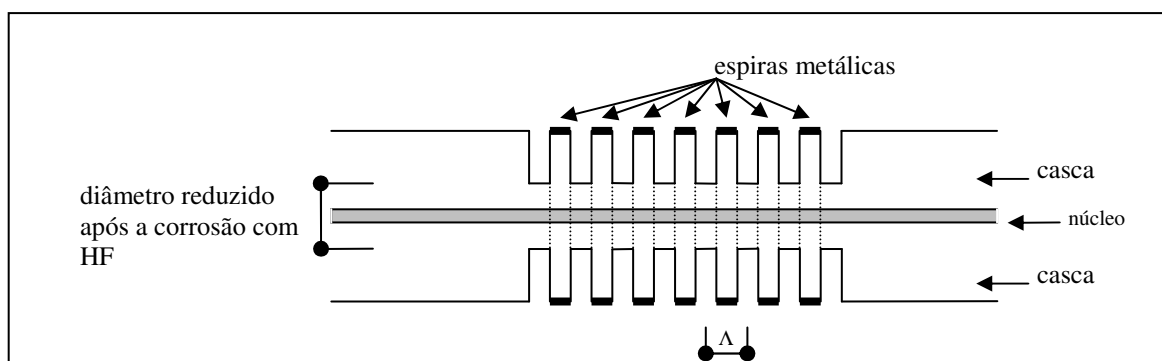
Figura 13: Corte longitudinal de uma LPG gravada através da corrosão periódica da casca da fibra óptica com HF (LIN E WANG, 1999).
