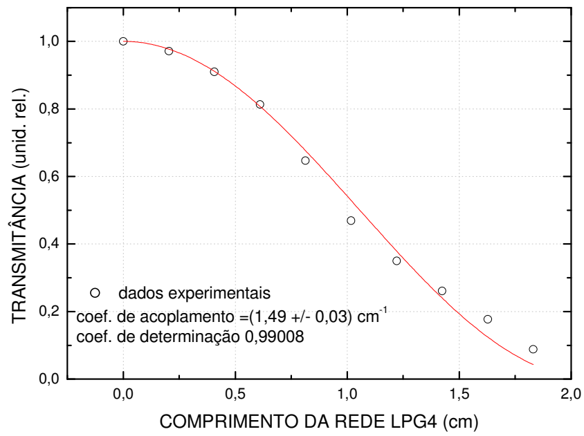
Determinação do coeficiente de acoplamento da LPG4
