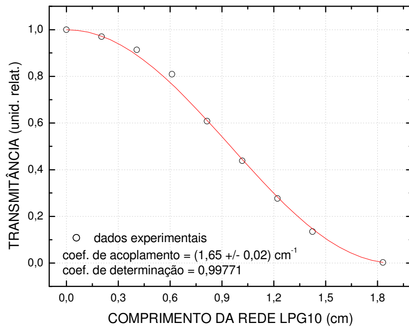
Determinação do coeficiente de acoplamento da LPG10
