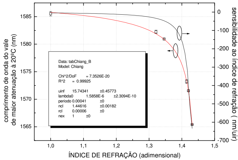
Ajuste da Equação de Chiang na LPG9
