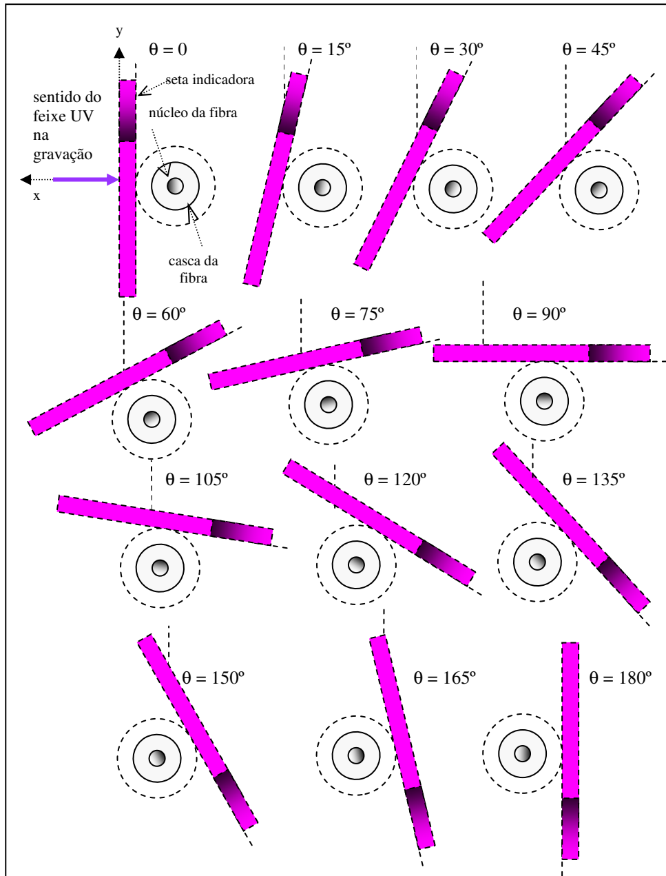
Figura 35: Ilustração fora de escala da secção transversal da LPG20, segundo o plano xy indicado na Figura 34, sendo rotacionada de 0 a 180°.
