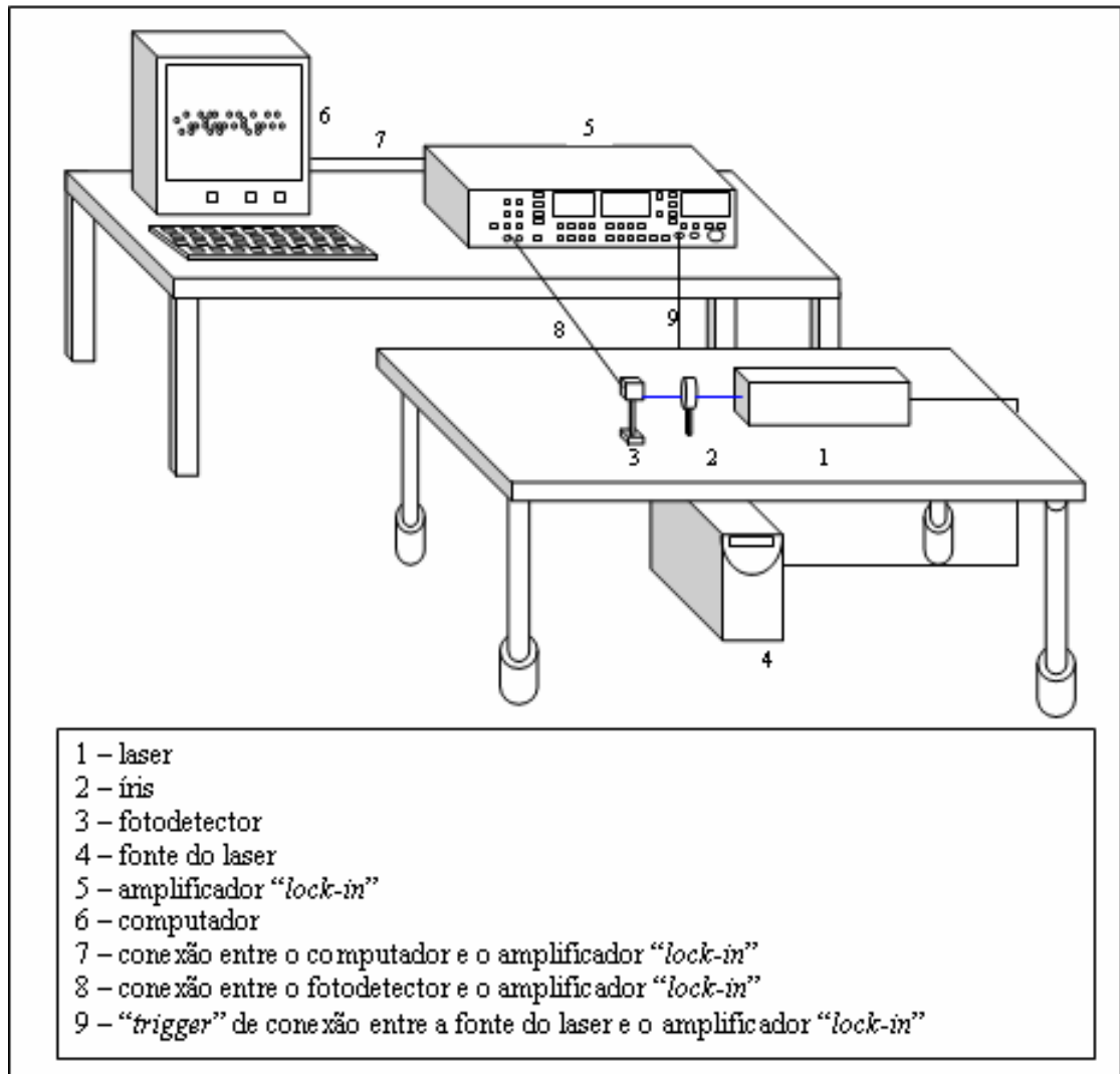
Figura 18: Esquema de montagem para a aquisição temporal da fluência do laser.
