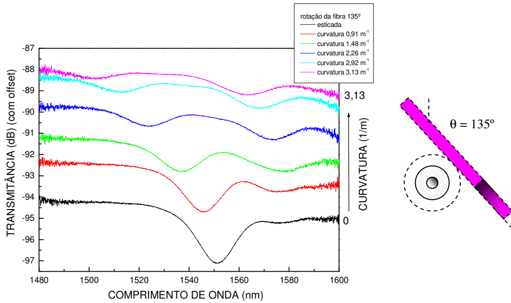
Resposta espectral da LPG20 submetida à curvaturas quando rotacionada de 135°.
