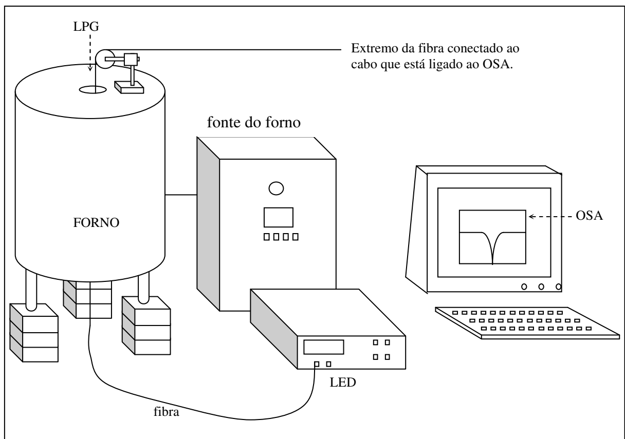
Figura 27: Arranjo experimental para o aquecimento das redes num forno de laboratório.
