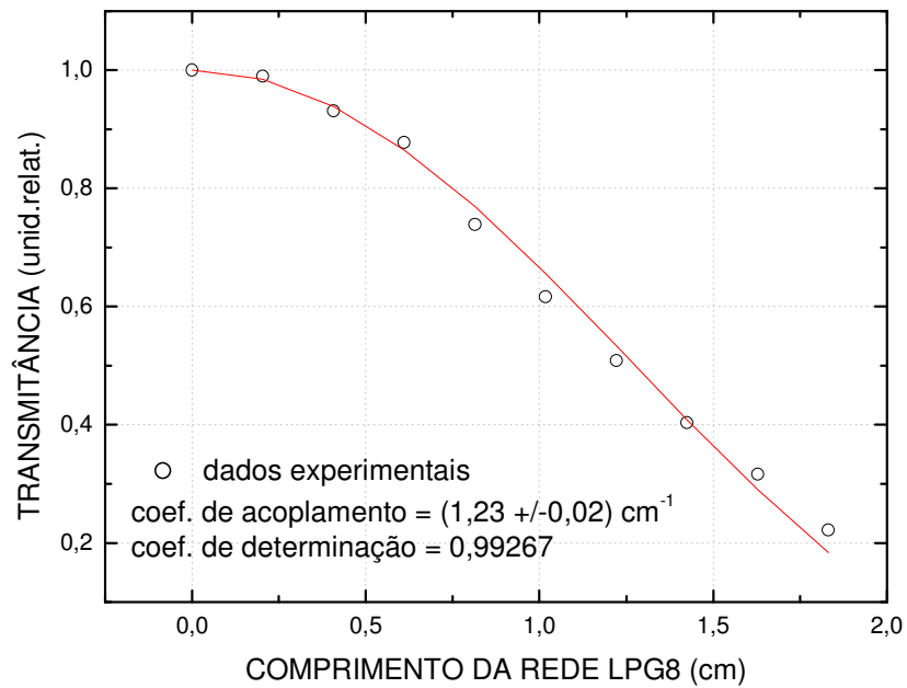
Determinação do coeficiente de acoplamento da LPG8
