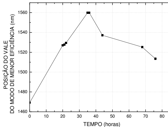
Figura 54: Acompanhamento da posição do vale da banda de menor eficiência da LPG9 após a gravação.
