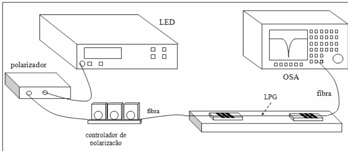
Figura 32: Arranjo experimental para testar a sensibilidade da LPG12 à mudanças no estado de polarização da luz por ela transmitida.
