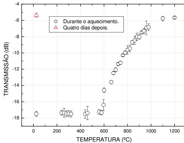
Figura 68: Medidas da atenuação da LPG3 nas temperaturas de 25°C a 1200°C e quatro dias depois do aquecimento a 24,7°C (COSTA, KAMIKAWACHI, MULLER et al , 2009).
