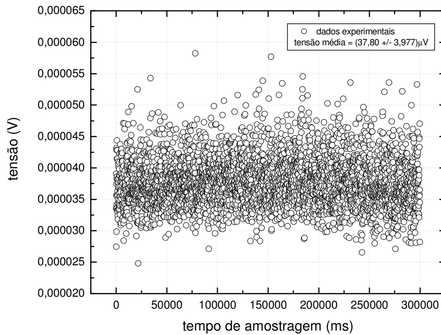
Figura 20: Segunda aquisição temporal do fotodetector com auxílio do amplificador “lock-in”.
