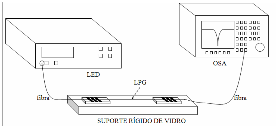
Figura 21: Esquema de como as redes LPG 9, LPG10, LPG11 e LPG13 ficaram fixadas durante os períodos de monitoramento dos seus espectros.
