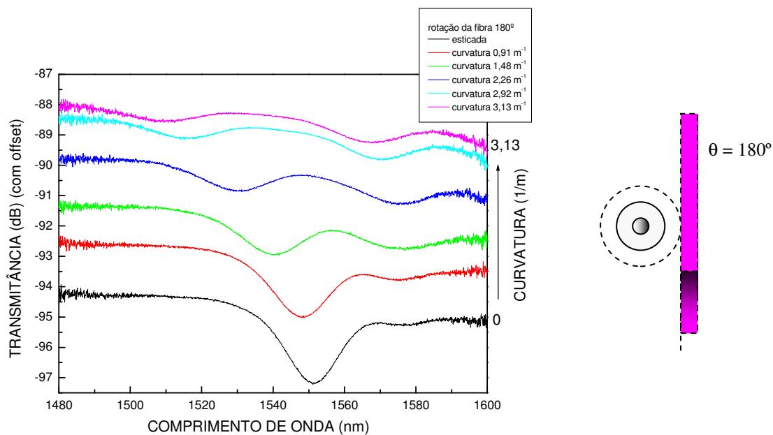
Resposta espectral da LPG20 submetida à curvaturas quando rotacionada de 180°.
