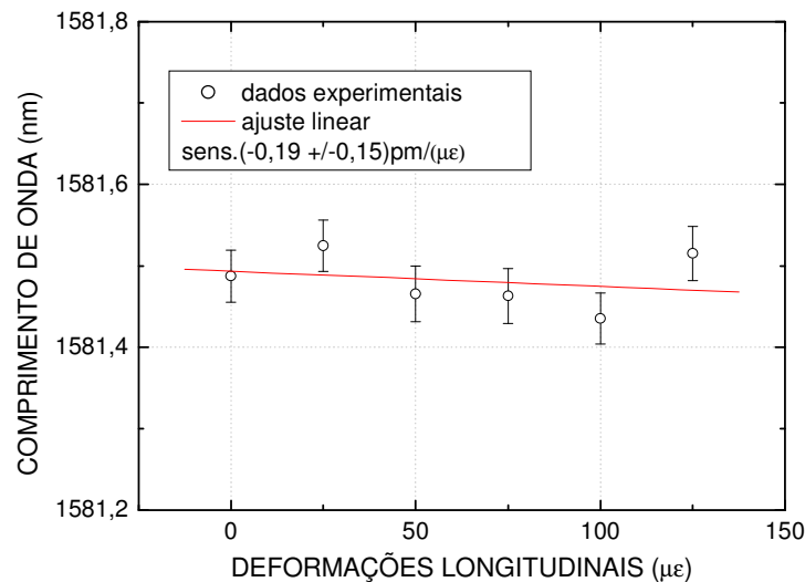
Figura 66: Sensibilidade da LPG9 à deformações longitudinais.
