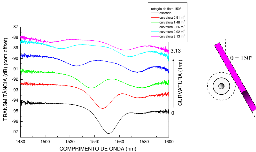
Resposta espectral da LPG20 submetida à curvaturas quando rotacionada de 150°.
