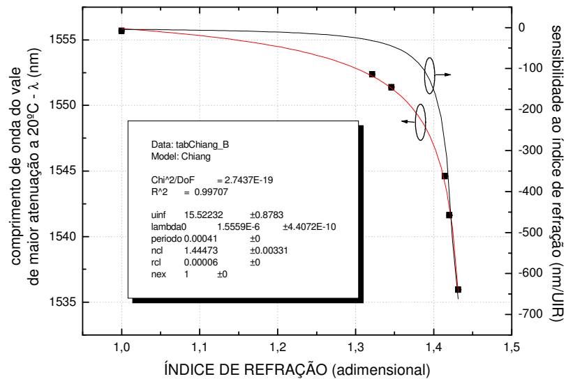
Ajuste da Equação de Chiang na LPG10
