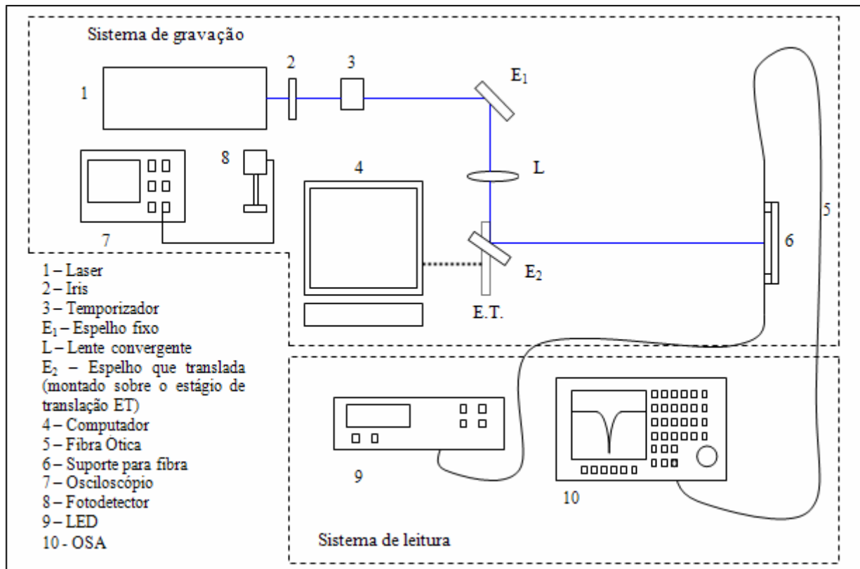
Figura 15: Diagrama esquemático do sistema de gravação ponto-a-ponto com laser UV e leitura de LPG
