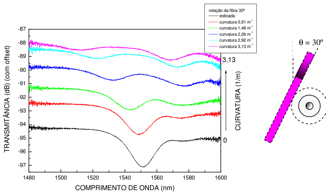
Resposta espectral da LPG20 submetida à curvaturas quando rotacionada de 30°.
