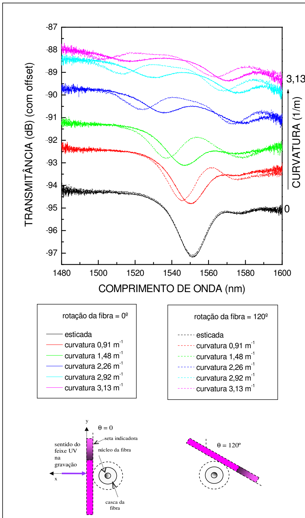
Figura 84: Respostas espectrais da LPG20 à curvatura quando rotacionada de 0° e de 120°.
