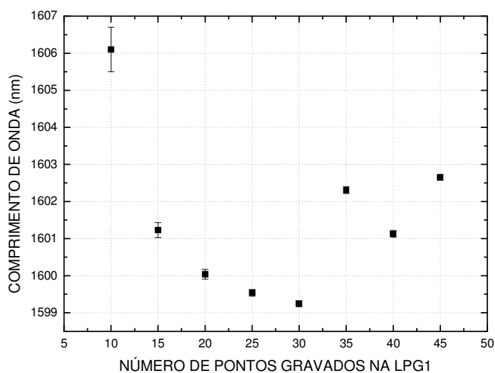
Figura 38: Evolução da posição do vale de maior atenuação da LPG1 (gravada com fluência de 278,65 \pm 30,65 \text{ mJ/cm}^2 ) à medida que os pontos iam sendo gravados nessa rede.
