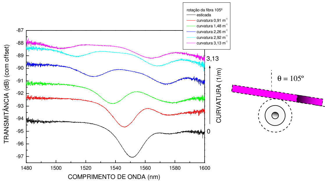
Resposta espectral da LPG20 submetida à curvaturas quando rotacionada de 105°.
