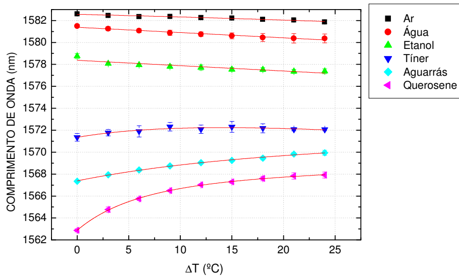
Figura 64: Resposta térmica da LPG9 na presença de diferentes ambientes com o ajuste fornecido pela Equação 49 (COSTA, KAMIKAWACHI, POSSETI et al , 2007).
