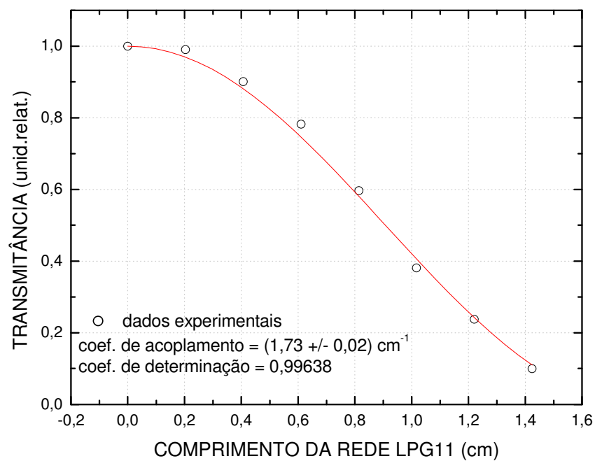
Determinação do coeficiente de acoplamento da LPG11
