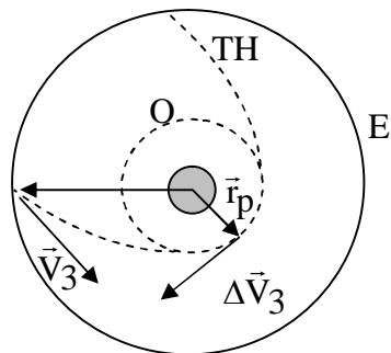
Figura 17 – Trajetória dentro da esfera de influência Lunar
