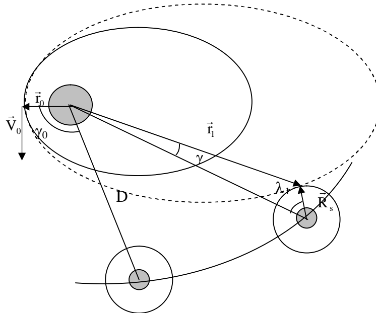
Figura 26 – Transferência da Terra para Lua
