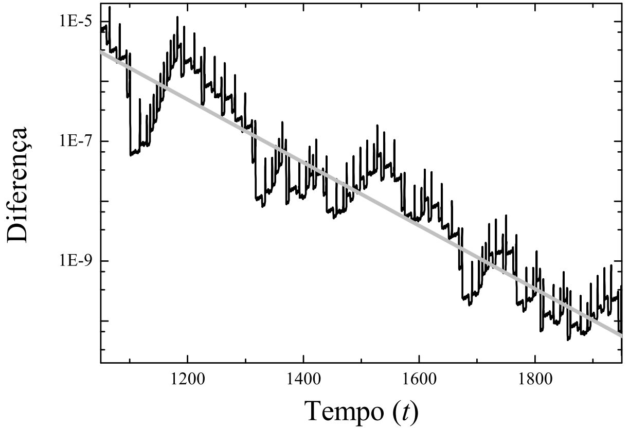
Figura 11: Evolução do módulo de uma diferença pequena entre as variáveis dos dois osciladores da figura 10. Percebe-se que o módulo segue uma lei exponencial. O coeficiente angular da reta ajustada vale aproximadamente 0,01/\ln 10 .
