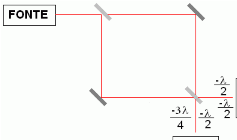
Figura4.4.2 - Superposição dos componentes do feixe emitido após o espelho semi-refletor S_2
