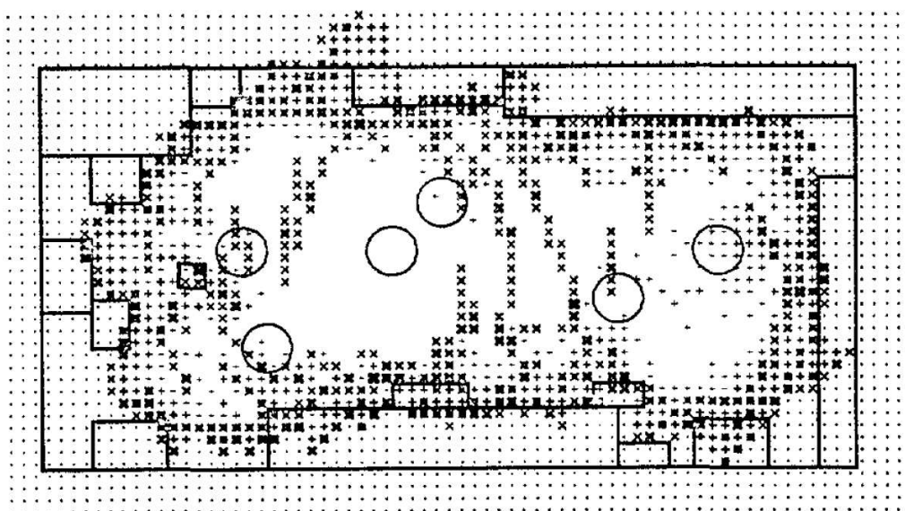
Figura 1: Mapa 2D gerado com o método Certainty Grid [5].
