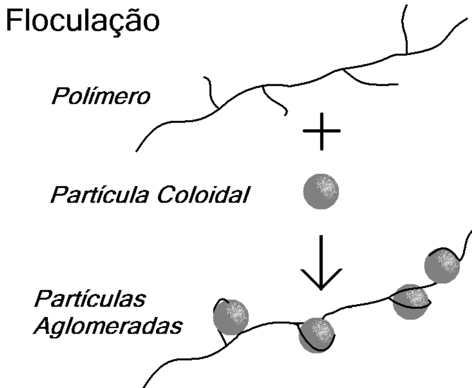
Figura 3.7: Aglomeração de partículas pelo polímero dando origem aos grandes flocos.
