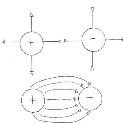
Na representação das linhas de campo, elas saem das cargas positivas e entram nas negativas.
