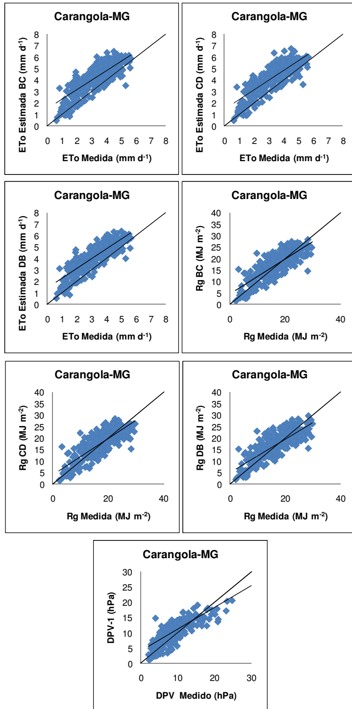
Figura 1A - Regressão linear dos valores diários para o ano de 2007 para a Evapotranspiração (ETo), Radiação Solar (Rg) e Déficit de Pressão de Vapor (DPV).
