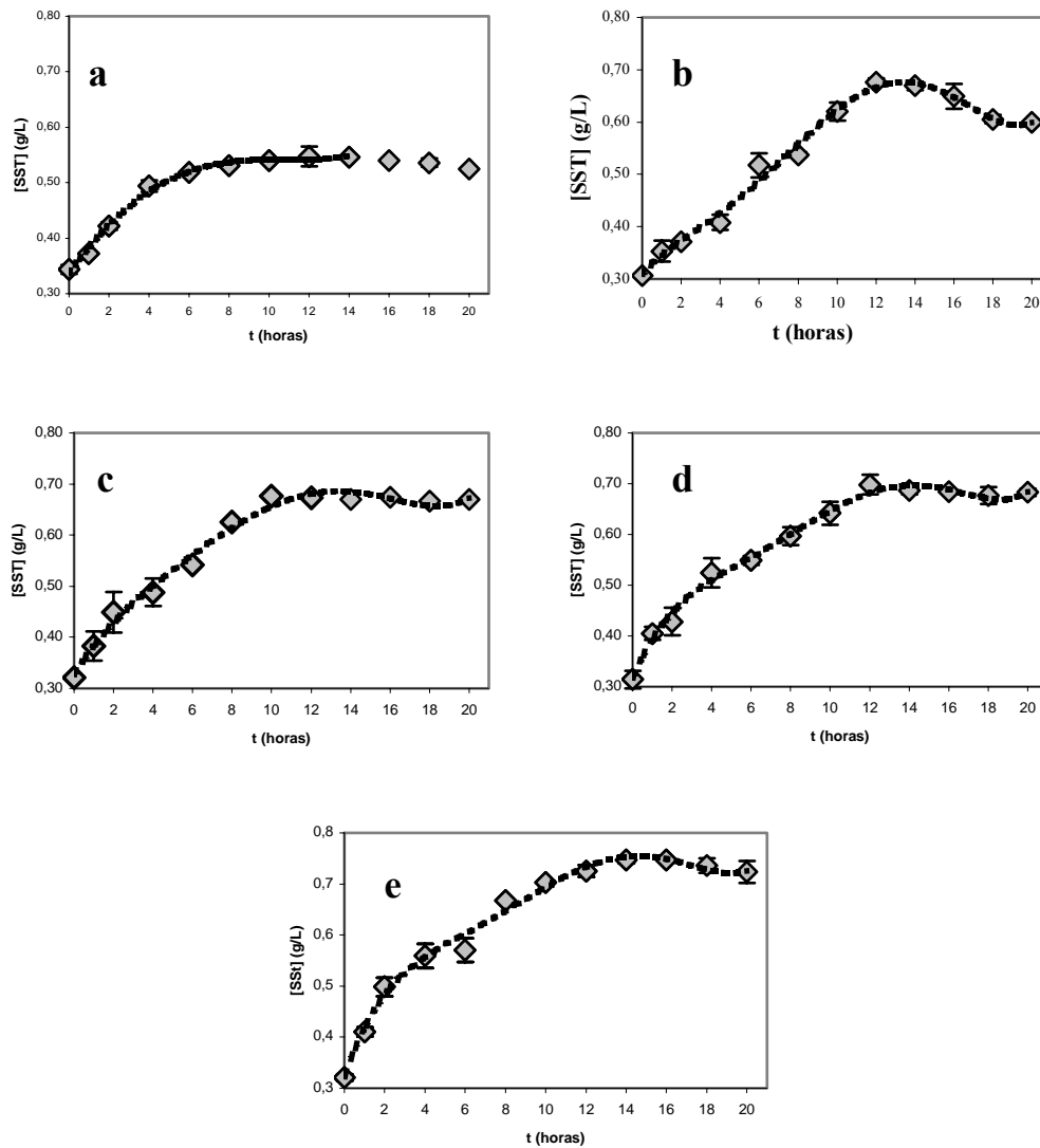
Figura 5.13: Crescimento celular em diferentes concentrações de S_0 . a) 103 mgN-NO 3 - /L, b) 227 mgN-NO 3 - /L, c) 315 mgN-NO 3 - /L, d) 415 mgN-NO 3 - /L, e) 512 mgN-NO 3 - /L.
