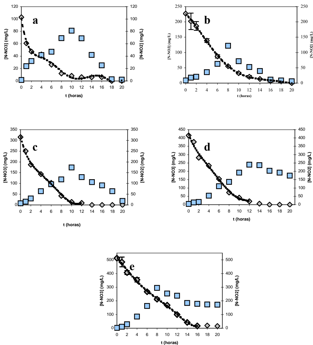
Figura 5.15: Concentração dos compostos nitrogenados ao longo do tempo em diferentes concentrações S_0 . a) 103 mgN-NO 3 - /L, b) 227 mgN-NO 3 - /L, c) 315 mgN-NO 3 - /L, d) 415 mgN-NO 3 - /L, e) 512 mgN-NO 3 - /L.
