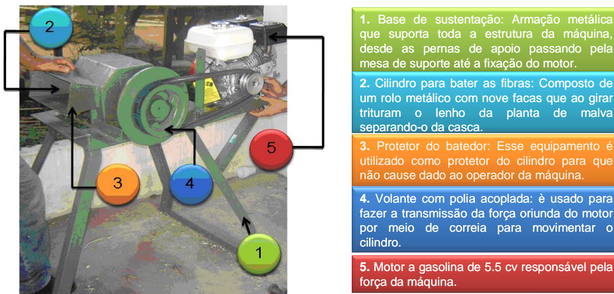
Figura 31 – Protótipo da máquina descortçadora de malva e/ou juta.
