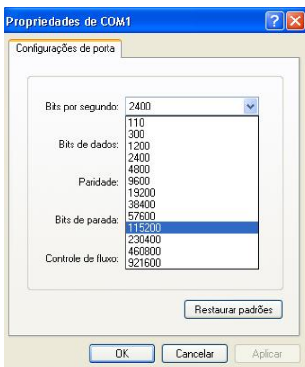
FIGURA 2.6 – Configuração de velocidade de transmissão da porta serial do Windows® FONTE: O autor (2007)
