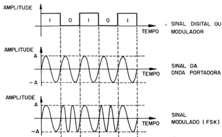
FIGURA 2.4 - Modulação FSK FONTE: AGHAZARM E MIRANDA (1988)
