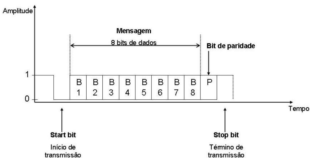
FIGURA 2.15 - Transmissão Assíncrona FONTE: AGHAZARM E MIRANDA (1988)
