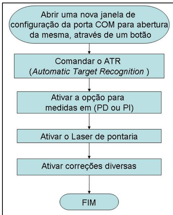
FIGURA 3.22 – Fluxograma de configuração da estação pelo programa. FONTE: O autor (2007)
