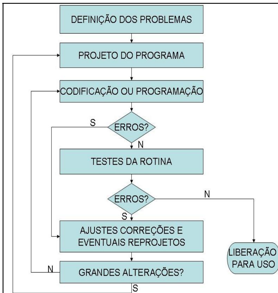
FIGURA 3.20 – Fluxograma das etapas de desenvolvimento de um programa. FONTE: CARVALHO (2001).
