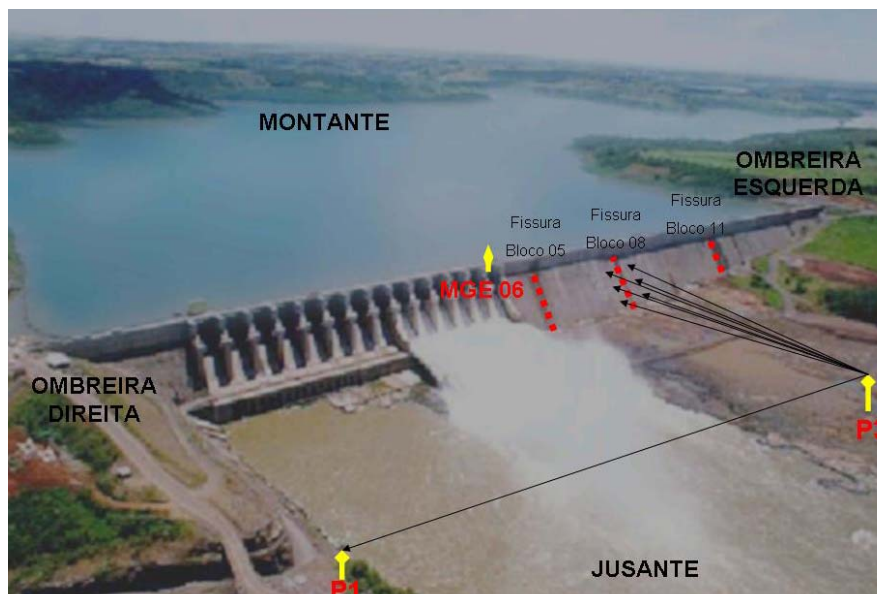
FIGURA 3.12 – Monitoramento das fissuras da barragem a partir dos pilares P1 e P3. FONTE: GRANEMANN (2004) – adaptado pelo autor
