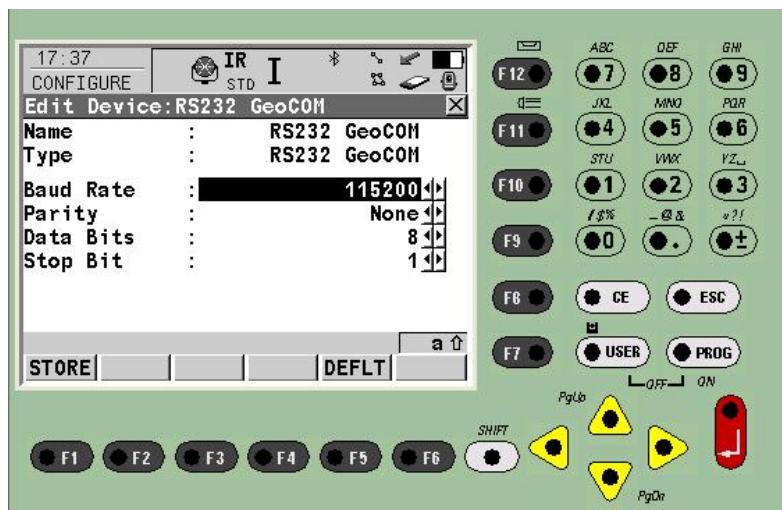
FIGURA 4.21 – Configuração de comunicação da TCRA1205 FONTE: LEICA (2006)
