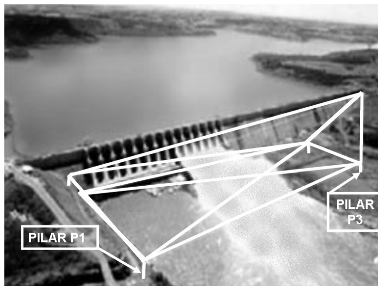
FIGURA 1.1 - Rede externa de monitoramento geodésico UHE Salto Caxias
