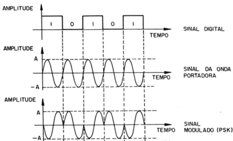
FIGURA 2.5 - Modulação PSK FONTE: AGHAZARM E MIRANDA (1988)
