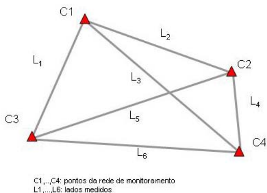
FIGURA 3.6 – Trilateração FONTE: VEIGA et al. (2006):
