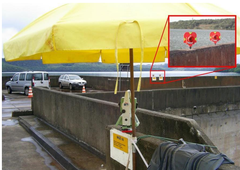
FIGURA 3.14 – Prismas posicionados em pontos a montante. FONTE: O autor (2007)
