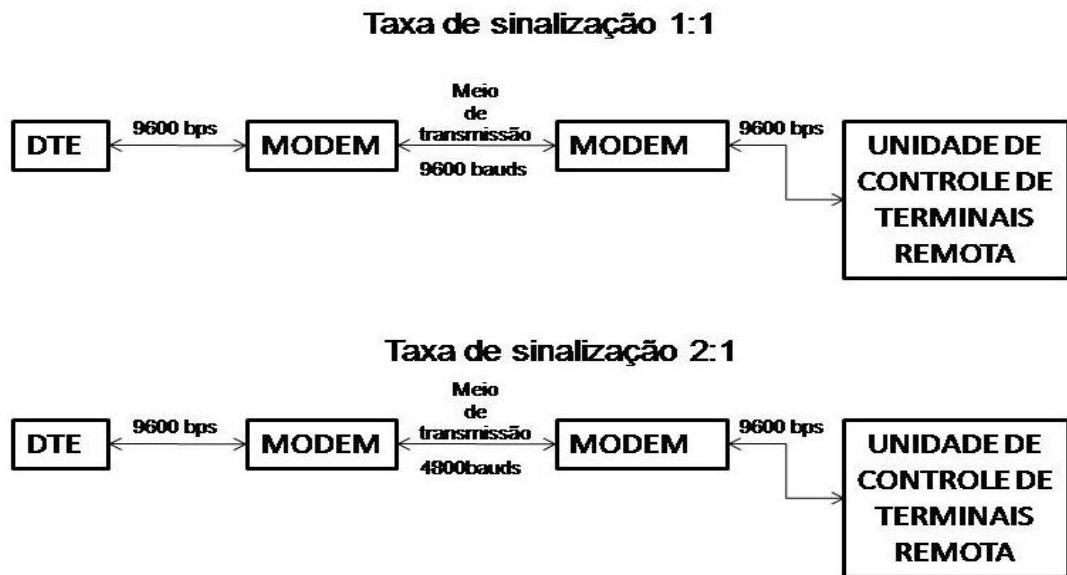
FIGURA 2.7 - Taxas de sinalização FONTE: AGHAZARM E MIRANDA (1988) – Adaptado pelo AUTOR.
