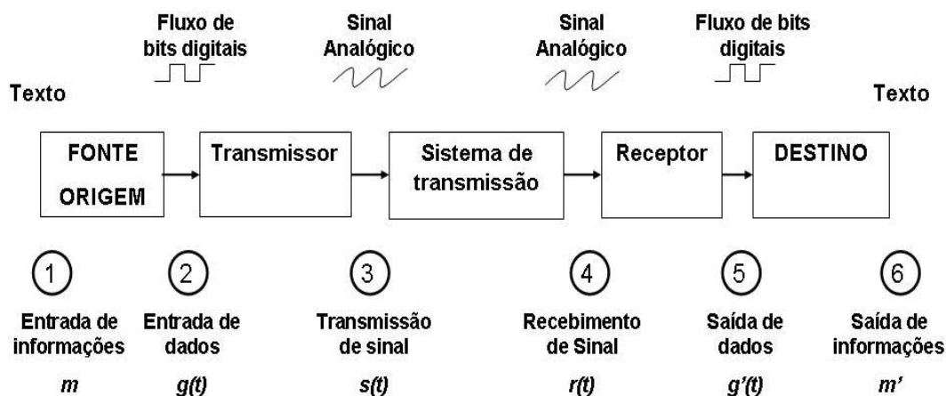
FIGURA 2.9 - Modelo simplificado de comunicação de dados FONTE: STALLINGS (2004)-Adaptado pelo autor.
