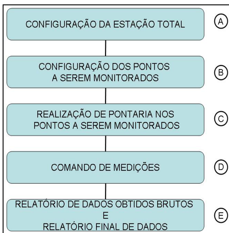
FIGURA 3.21 – Fluxograma de módulos que o programa de controle deve cumprir. FONTE: O autor (2007)
