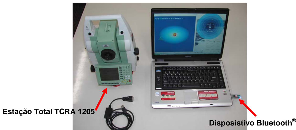
FIGURA 4.16 – Emparelhamento da TCRA1205 com o Notebook através do dispositivo Bluetooth ® FONTE: O autor (2007)
