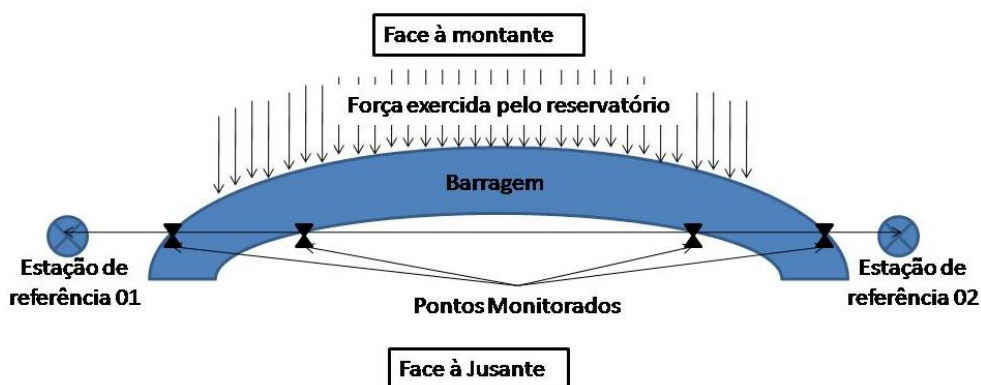
FIGURA 2.1 - Método dos alinhamentos FONTE: O autor (2007)
