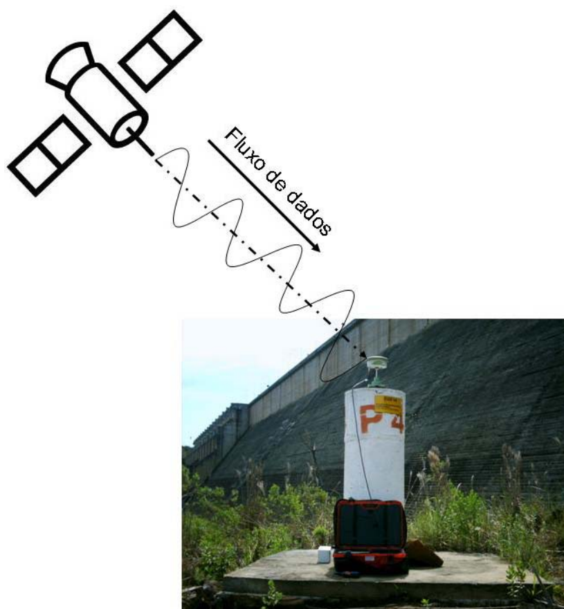
FIGURA 2.10 - Modo de operação simplex FONTE: O autor (2007).
