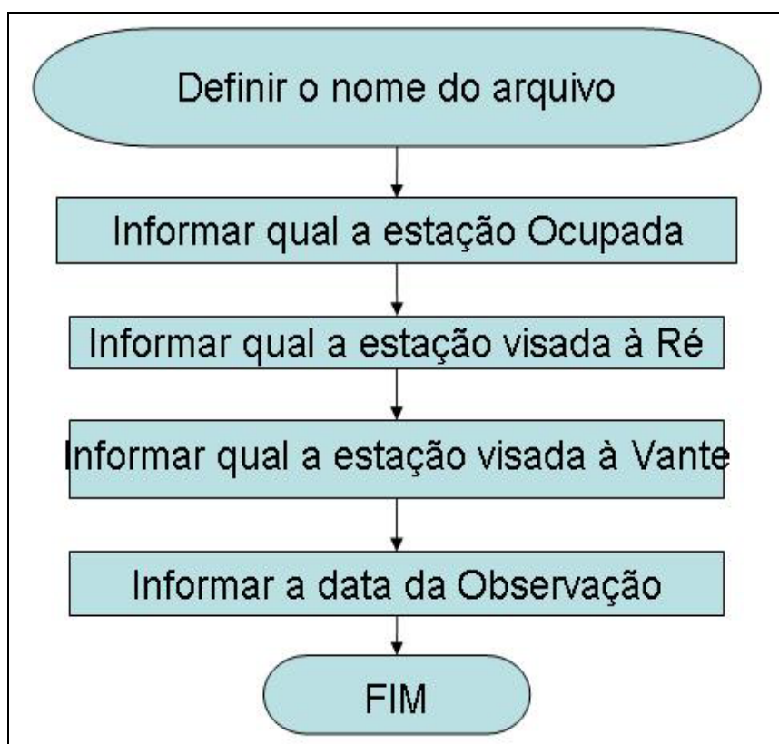
FIGURA 3.23 – Fluxograma de configuração dos pontos medidos FONTE: O autor (2007)
