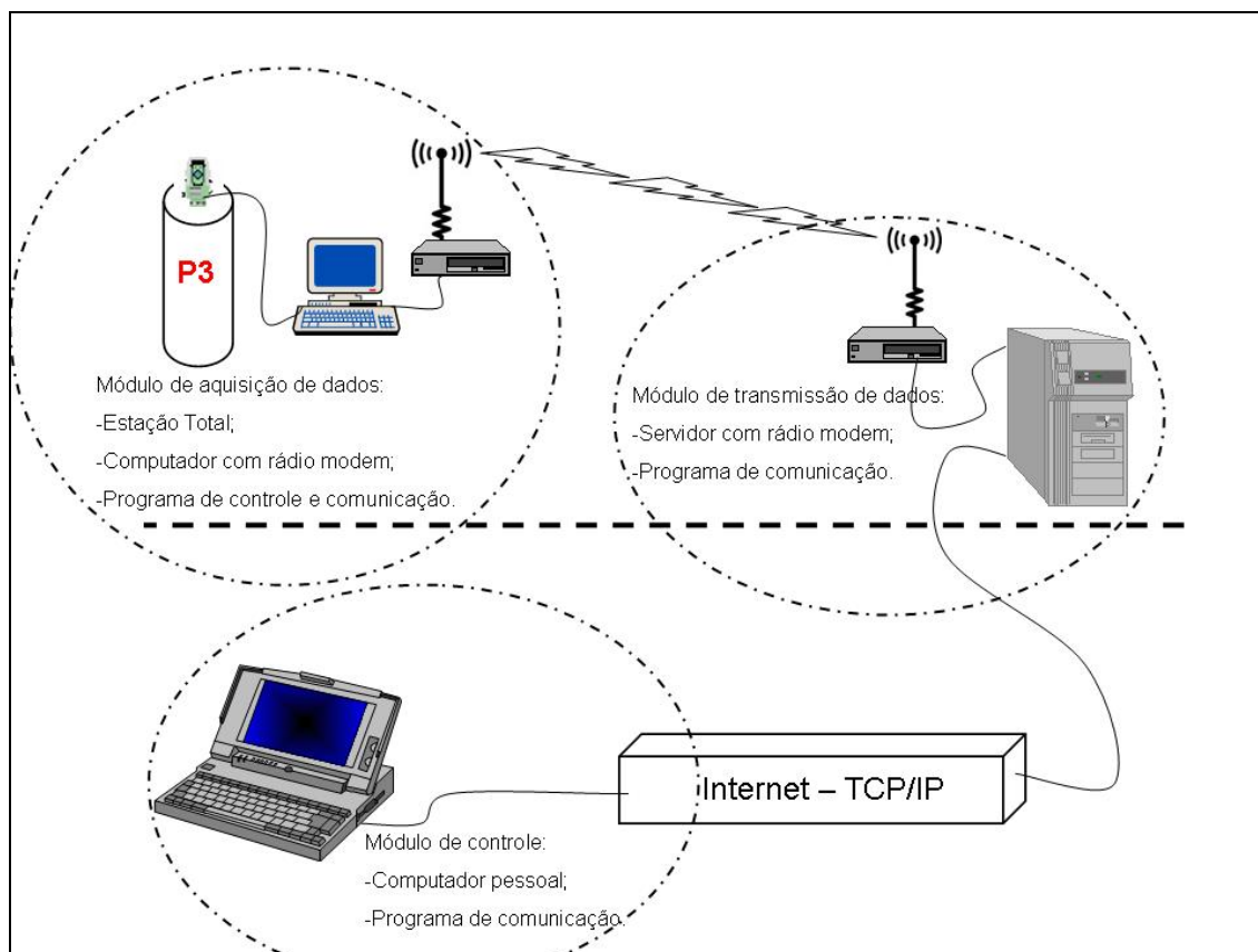
FIGURA 3.16 – Esquema do sistema de automação do Levantamento Geodésico: FONTE: O autor (2007)
