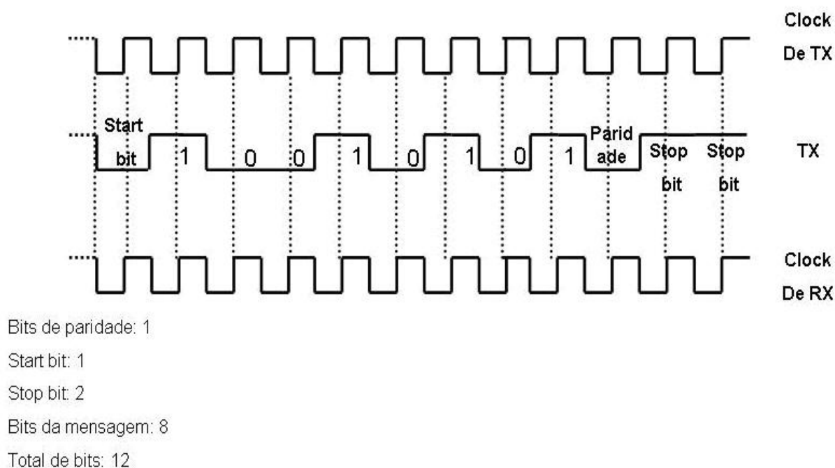
FIGURA 2.16 - Típica mensagem de transmissão assíncrona. FONTE: AGHAZARM E MIRANDA (1988)
