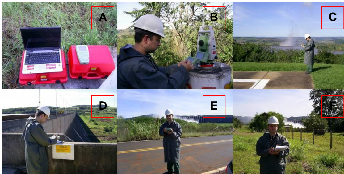
FIGURA 4.25 – Teste de alcance efetivo de rádio-modem. FONTE: O autor (2007)
