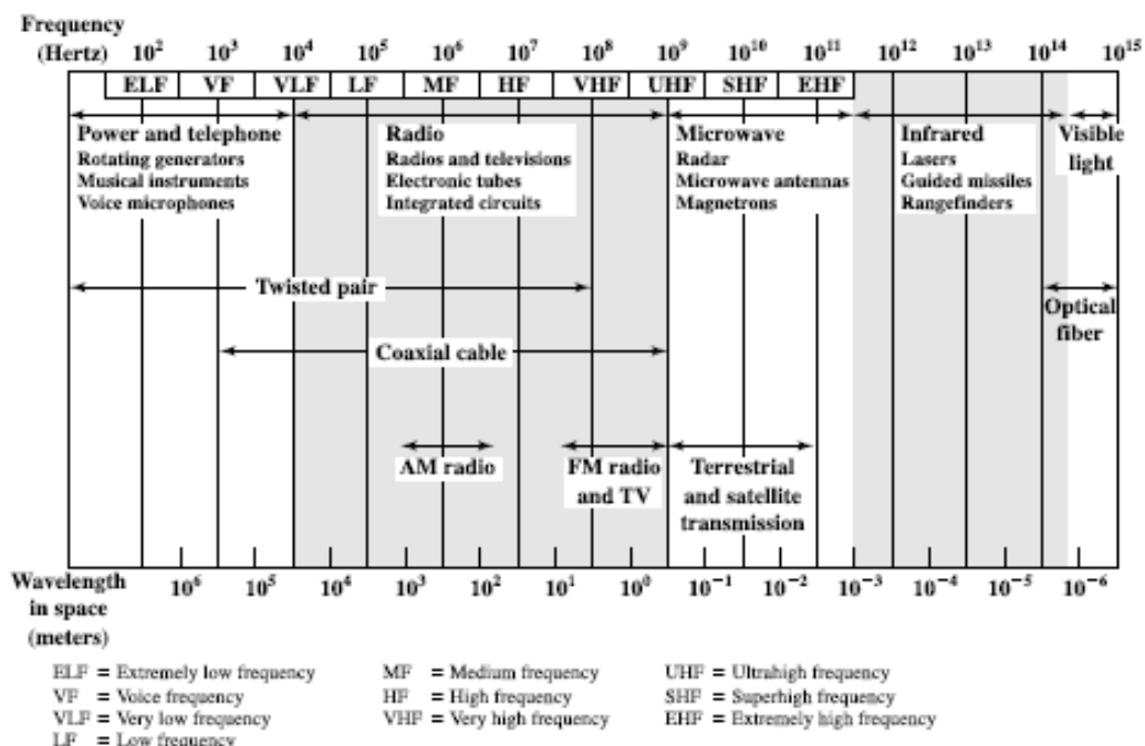
FIGURA 2.20 - Frequências no espectro FONTE: STALLINGS (2004, p.95)
