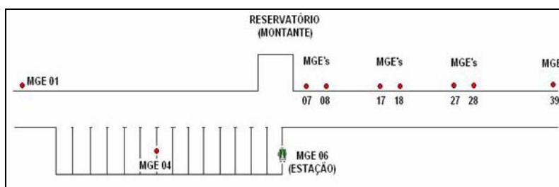
FIGURA 3.13 – Esquema dos pontos de monitoramento a montante. FONTE: VEIGA et al. (2006):
