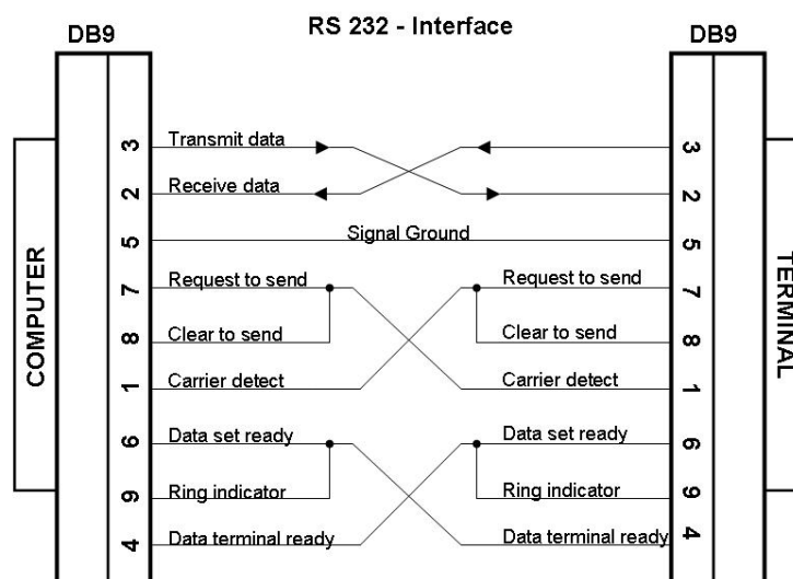
FIGURA 2.18 - Interface RS232C com o computador via DB9 FONTE: CAMPBELL (1986) adaptado pelo autor
