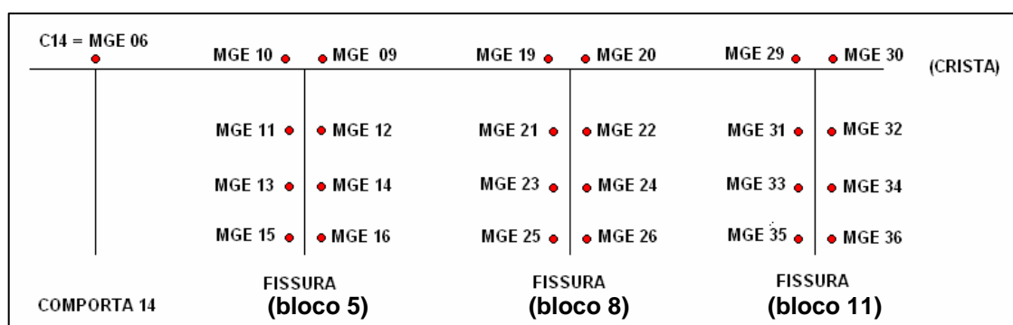
FIGURA 3.9 –Pontos a jusante observados a partir do pilar P3 (Rede Externa). FONTE: VEIGA et al. (2006) – adaptado pelo autor
