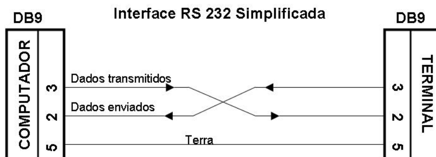
FIGURA 2.20 - Interface RS232 com o computador via DB9 simplificada FONTE: o autor
