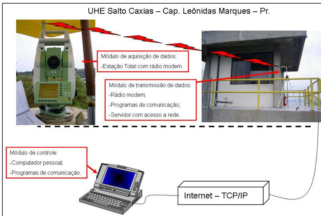
FIGURA 3.17 – Esquema do conjunto de monitoramento a distância FONTE: O autor (2007)
