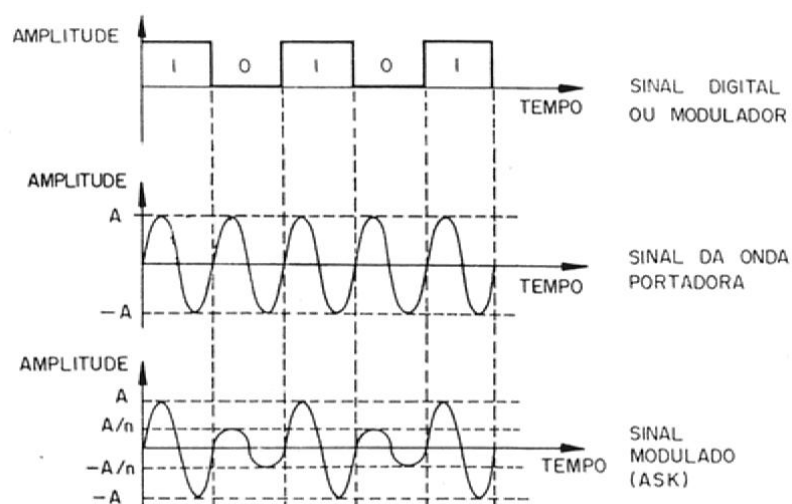
FIGURA 2.3 - Modulação ASK FONTE: AGHAZARM E MIRANDA (1988)
