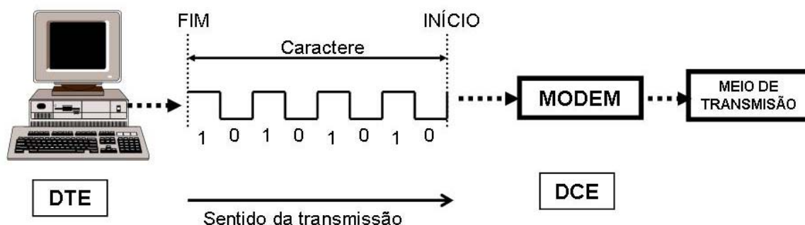
FIGURA 2.13 - Transmissão Serial FONTE: O autor (2007)
