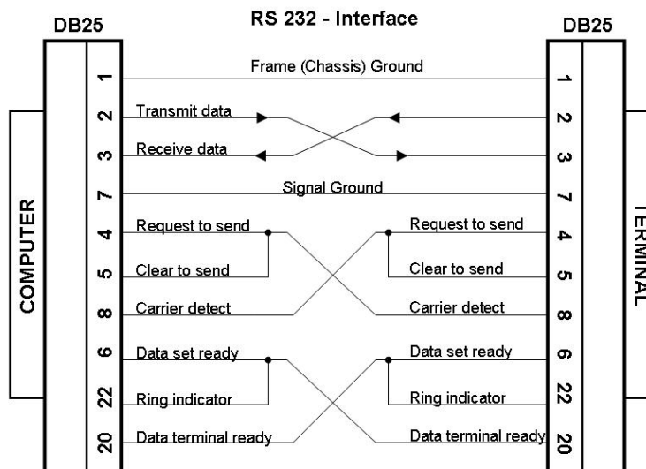
FIGURA 2.19 - Interface RS232C com o computador via DB25 FONTE: CAMPBELL (1986) adaptado pelo autor
