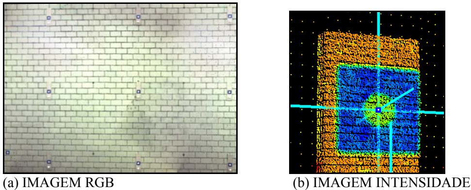
FIGURA 5.16: PAREDE VARRIDA PELO LASER SCANNER
