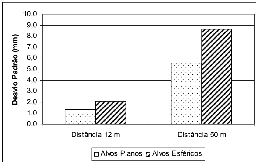
FIGURA 5.21: ALVOS PLANOS x ESFÉRICOS - DISTÂNCIAS VERTICAIS
