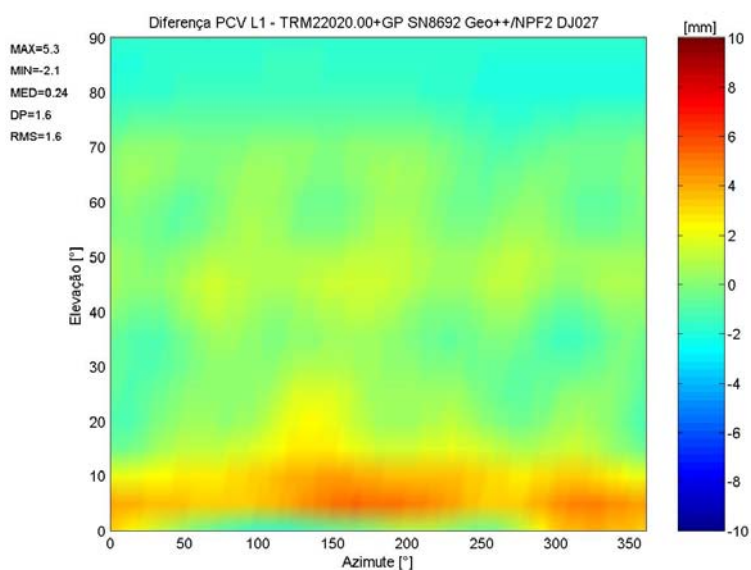
FIGURA 87–DIFERENÇAS DAS PCV DEPENDENTES DE AZIMUTE E ELEVAÇÃO ENTRE RESULTADOS GEO++ E GIK (PILAR NPF2) NA PORTADORA L1, TRM22020.00+GP SN8692
