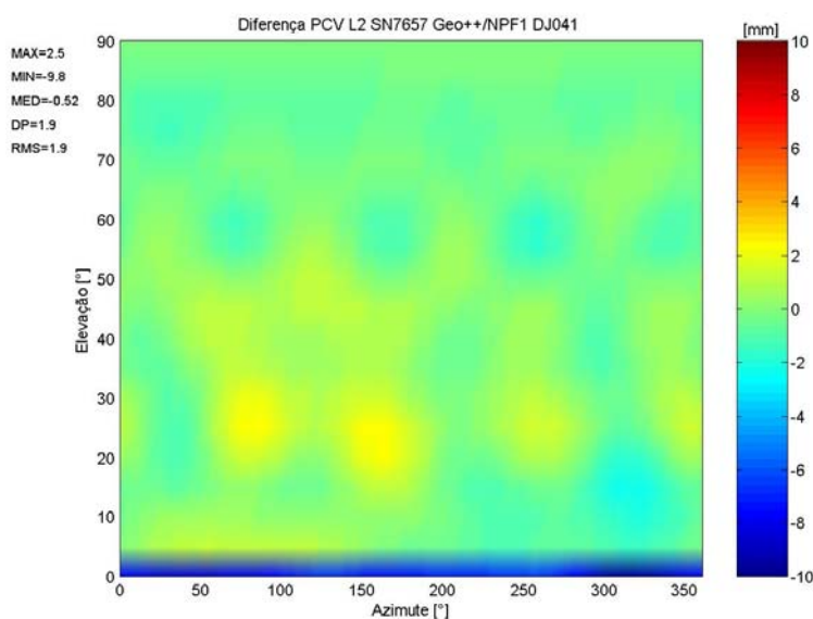
FIGURA 92–DIFERENÇAS DAS PCV DEPENDENTES DE AZIMUTE E ELEVAÇÃO ENTRE RESULTADOS GEO++ E GIK (PILAR NPF1) NA PORTADORA L2, TRM29659.00 SN7657
