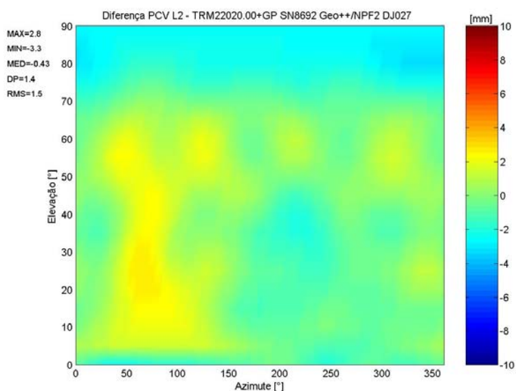
FIGURA 88–DIFERENÇAS DAS PCV DEPENDENTES DE AZIMUTE E ELEVAÇÃO ENTRE RESULTADOS GEO++ E GIK (PILAR NPF2) NA PORTADORA L2, TRM22020.00+GP SN8692
