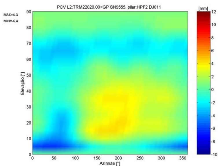
FIGURA 96—PCV DEPENDENTES DE AZIMUTE E ELEVAÇÃO NA PORTADORA L2, ANTENA TRM22020.00+GP SN9555, PILAR HPF2
