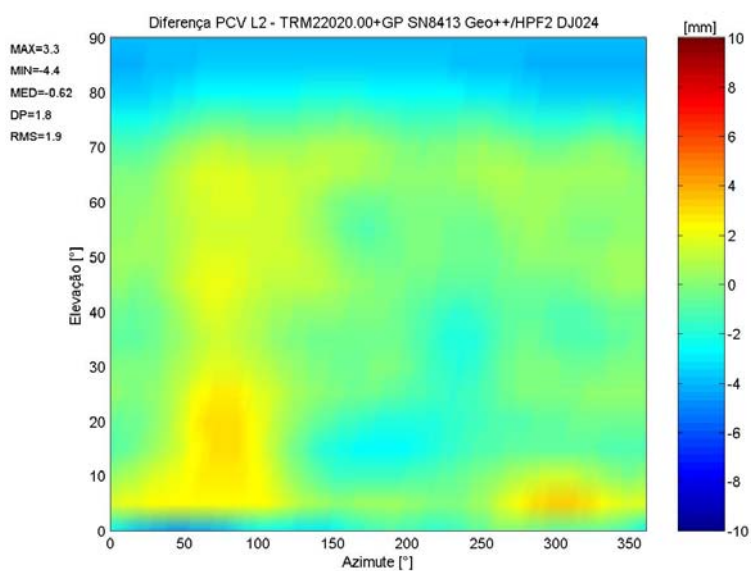
FIGURA 86–DIFERENÇAS DAS PCV DEPENDENTES DE AZIMUTE E ELEVAÇÃO ENTRE RESULTADOS GEO++ E GIK (PILAR HPF2) NA PORTADORA L2, TRM22020.00+GP SN8692
