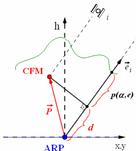
FIGURA 14–DEDUÇÃO DAS VARIAÇÕES DO CENTRO DE FASE
