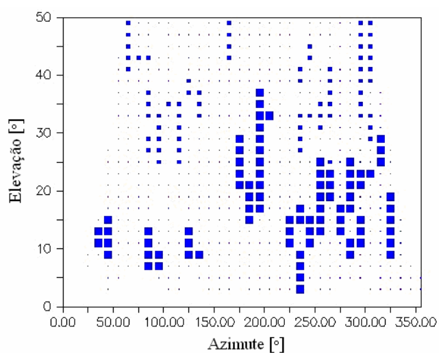
FIGURA 126–DETECCÃO E LOCALIZAÇÃO DO EFEITO DE MULTICAMINHO, ADAPTADOR LONGO, ANTENA TRM22020.00+GP SN8918, PILAR HPF1
