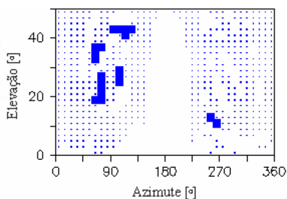
FIGURA 147–DETECCÃO E LOCALIZAÇÃO DO EFEITO DE MULTICAMINHO NO PILAR 1000 (OESTE), ANTENA LEIAT504 ( CHOKE RING )
