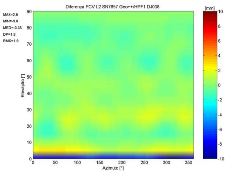
FIGURA 90–DIFERENÇAS DAS PCV DEPENDENTES DE AZIMUTE E ELEVAÇÃO ENTRE RESULTADOS GEO++ E GIK (PILAR HPF1) NA PORTADORA L2, TRM29659.00 SN7657
