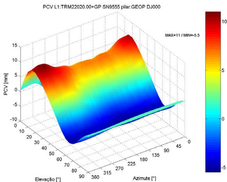
FIGURA 79–PCV DEPENDENTE DE AZIMUTE E ELEVÇÃO NA PORTADORA L_1 , ANTENA TRM22020.00+GP SN9555, CALIBRAÇÃO ABSOLUTA GEO++
