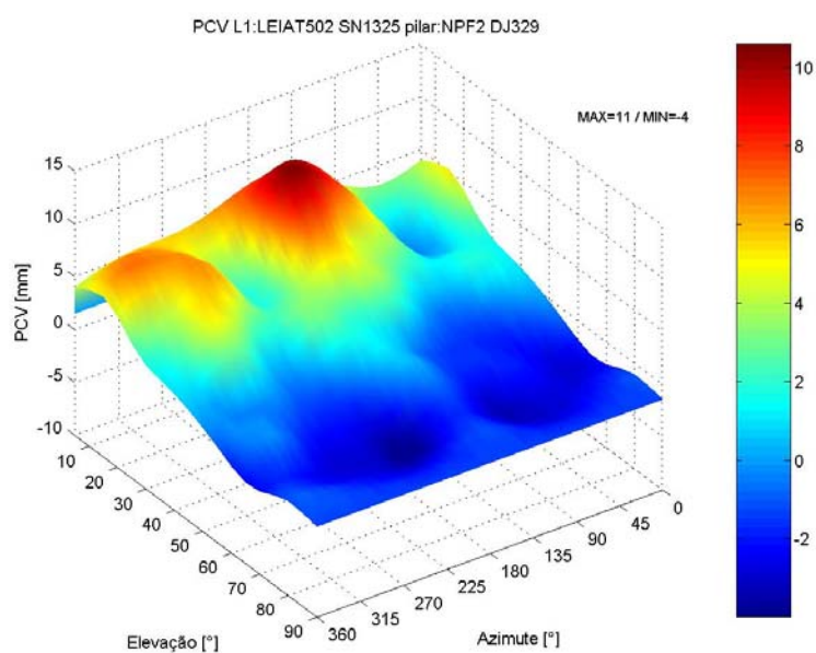
FIGURA 62–REPRESENTAÇÃO TRIDIMENSIONAL DAS PCV DEPENDENTES DE AZIMUTE E ELEVÇÃO NA PORTADORA L1, ANTENA LEIAT502, PILAR NPF2
