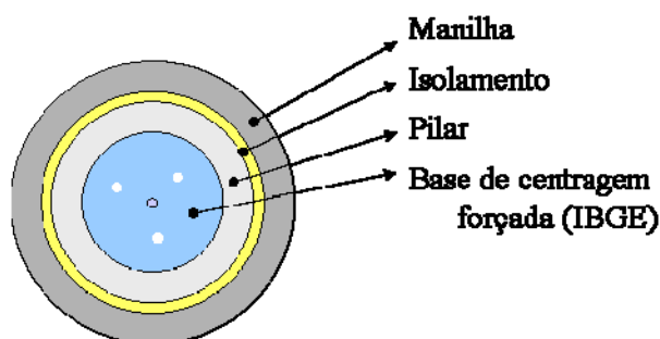
FIGURA 140–CORTE TRANSVERSAL DOS PILARES DE CALIBRAÇÃO
