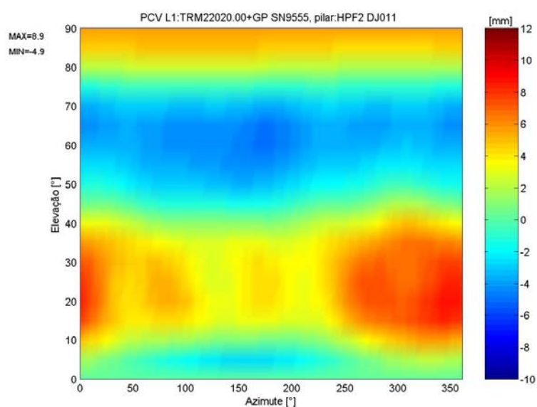
FIGURA 95—PCV DEPENDENTES DE AZIMUTE E ELEVAÇÃO NA PORTADORA L1, ANTENA TRM22020.00+GP SN9555, PILAR HPF2
