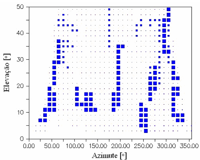
FIGURA 128–DETECCÃO E LOCALIZAÇÃO DO EFEITO DE MULTICAMINHO, ADAPTADOR LONGO, ANTENA TRM22020.00+GP SN8918, PILAR HPF2
