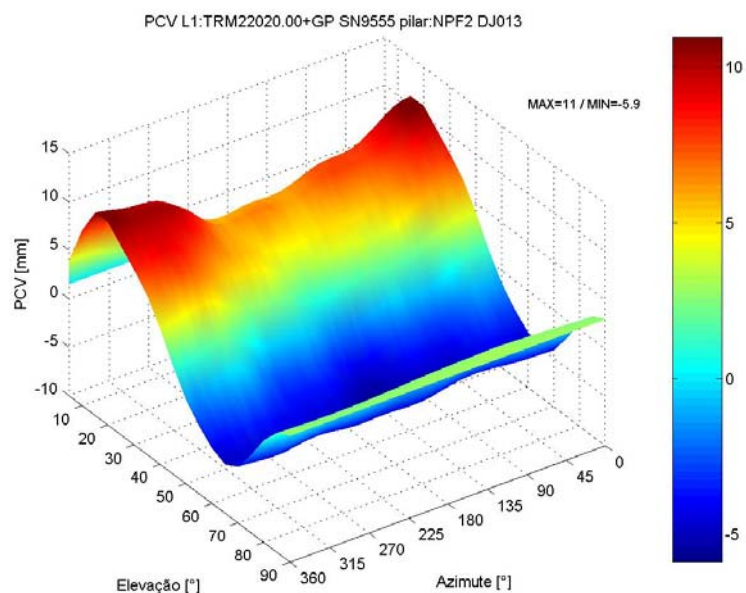
FIGURA 83–PCV DEPENDENTE DE AZIMUTE E ELEVAÇÃO NA PORTADORA L1, ANTENA TRM22020.00+GP SN9555, CALIBRAÇÃO NO PILAR NPF2
