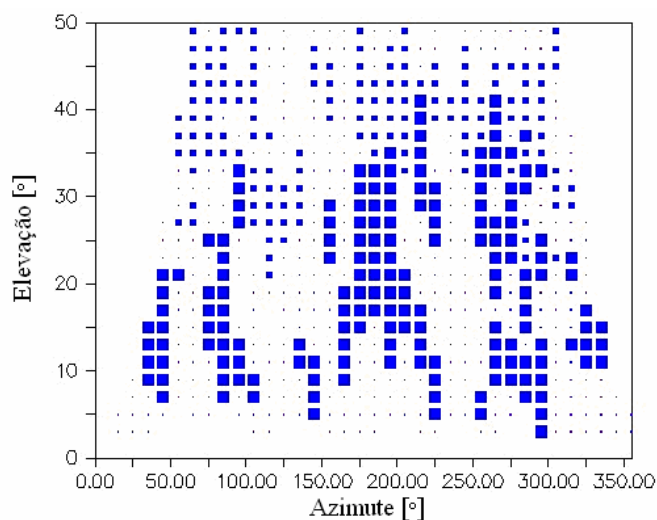
FIGURA 130–DETECCÃO E LOCALIZAÇÃO DO EFEITO DE MULTICAMINHO, ADAPTADOR LONGO, ANTENA TRM22020.00+GP SN8918, PILAR NPF2
