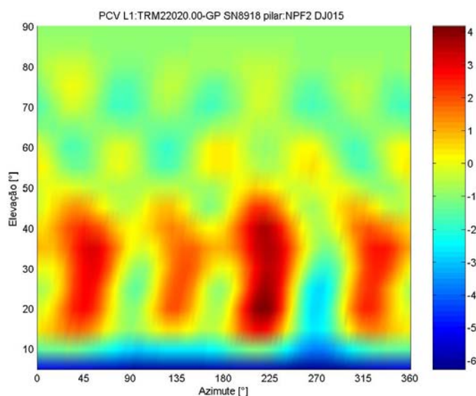
FIGURA 118–PCV DEPENDENTE DE ELEVAÇÃO E AZIMUTE NA FREQUÊNCIA L_1 (REPRESENTAÇÃO PLANA), ANTENA TRM22020.00-GP SN8918, PILAR NPF2
