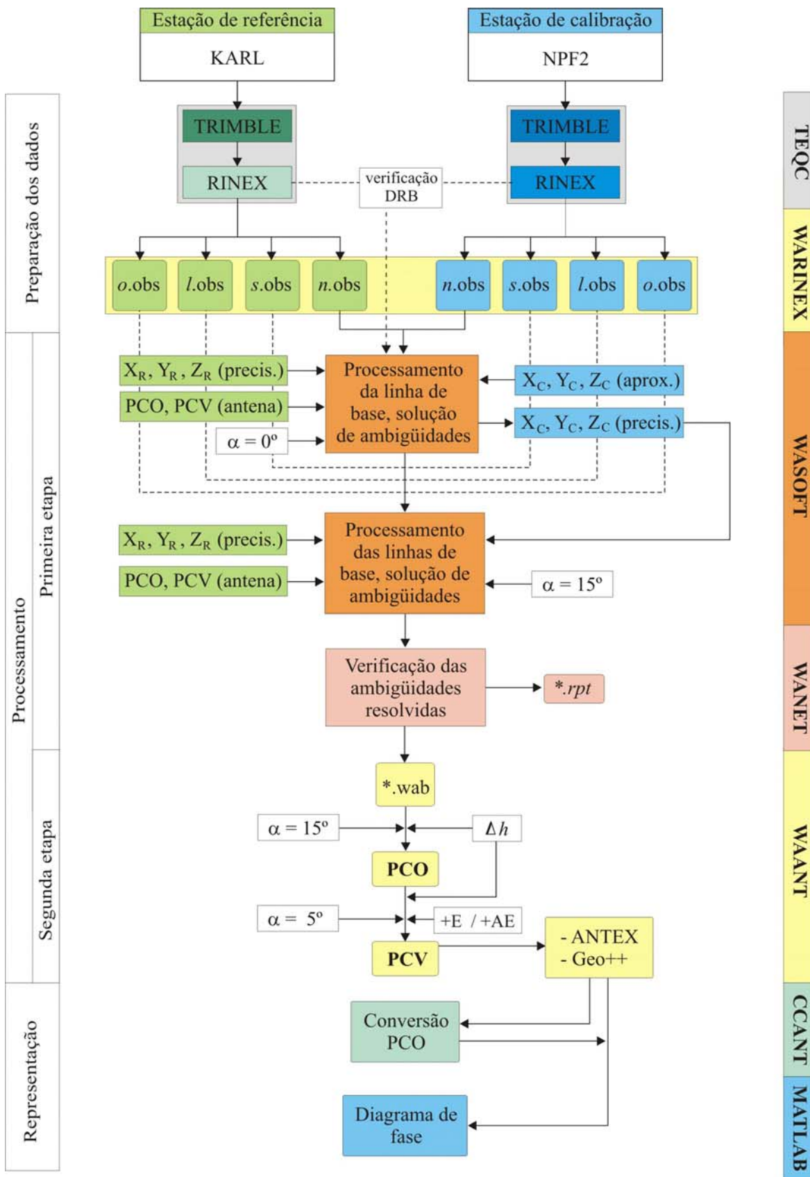
QUADRO 13 – FLUXOGRAMA DO PROCESSAMENTO DA CALIBRAÇÃO
