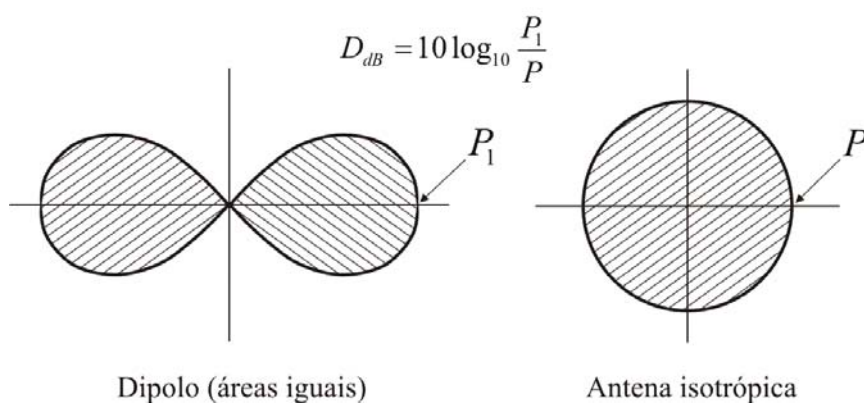
FIGURA 11—CONCEITO DE DIRETIVIDADE
