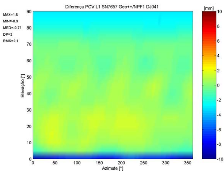
FIGURA 91–DIFERENÇAS DAS PCV DEPENDENTES DE AZIMUTE E ELEVAÇÃO ENTRE RESULTADOS GEO++ E GIK (PILAR NPF1) NA PORTADORA L1, TRM29659.00 SN7657
