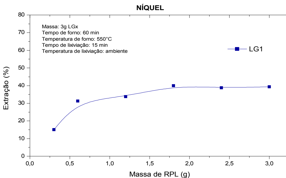
Figura 21: Influência da massa de RPL na extração de níquel.
