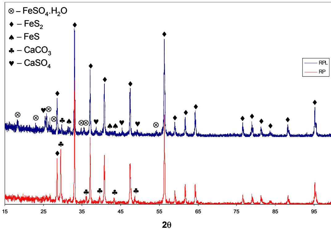
Figura 15: Difratogramas de RP e RPL, indicando as fases presentes antes e depois do ataque com ácido clorídrico.
