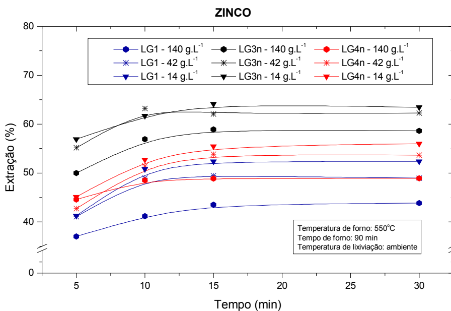
Figura 33: Influência do teor de sólidos em polpa e do tempo de lixiviação na extração de zinco.
