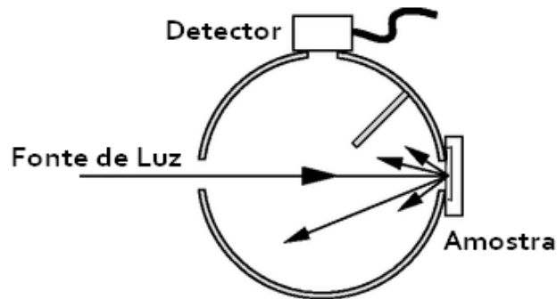
Figura 2.12: Estrutura básica de um sistema de ERD. A fonte de luz varre o espectro ultravioleta até o infravermelho próximo.
