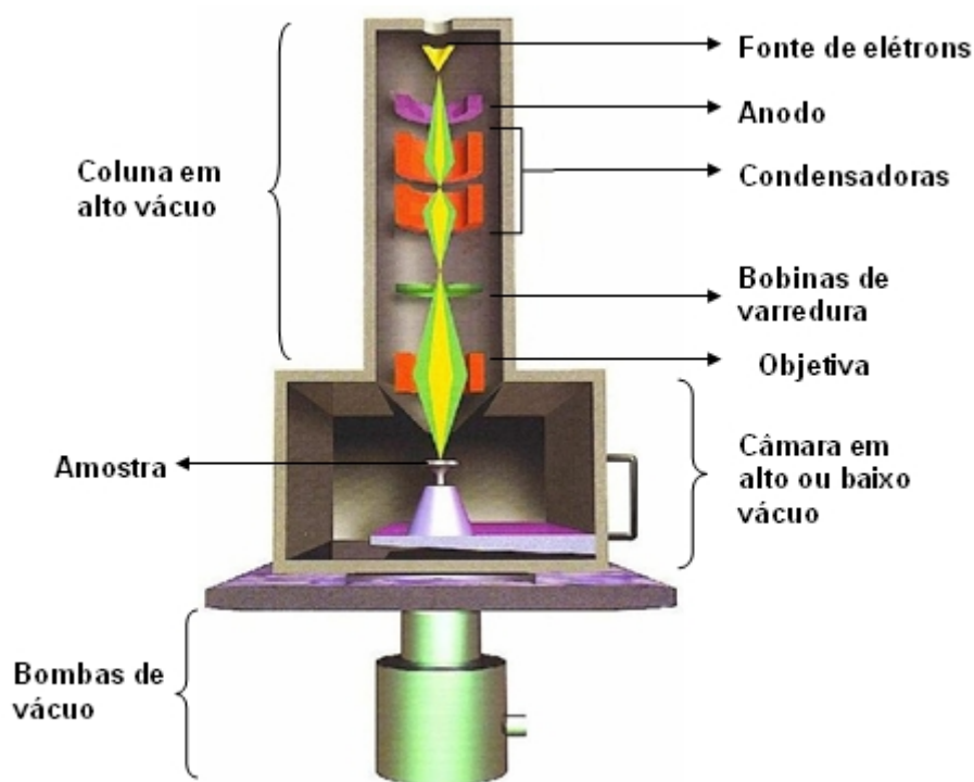
Figura 2.4: Estrutura de uma torre de microscopia eletrônica de varredura [68].
