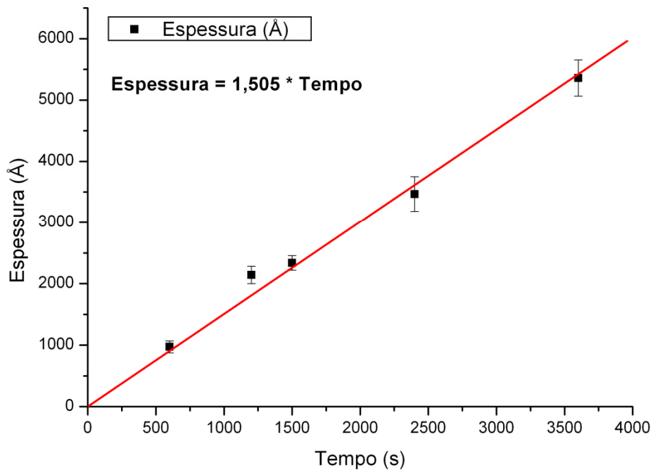
Figura 2.2: (a) Perfis obtidos através de perfilometria, de amostras de filmes finos de titânio sobre Si (111). (b) Aproximação linear da taxa de deposição do sistema de sputtering utilizado no LFF-UFRGS para amostras de Ti/Si.
