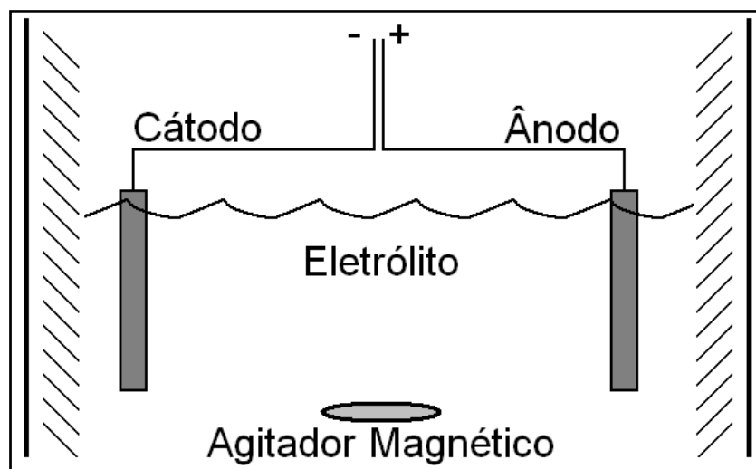
Figura 1.6: Esquemática de uma célula eletrolítica. A amostra de titânio é colocada como o ânodo, e um metal inerte à solução (e.g. platina) faz o papel do cátodo.
