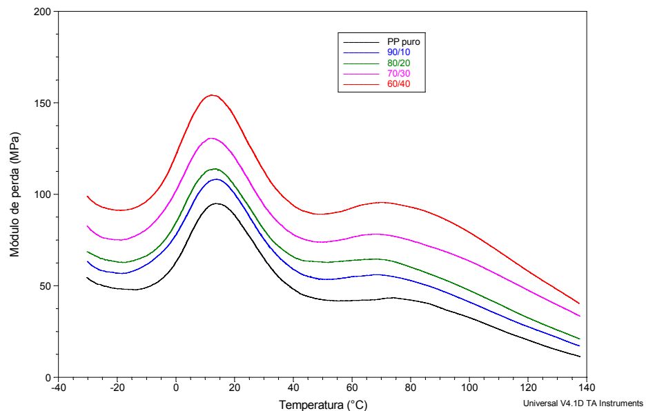
Figura 4.15 Módulo de perda do PP e dos compósitos com CA-A
