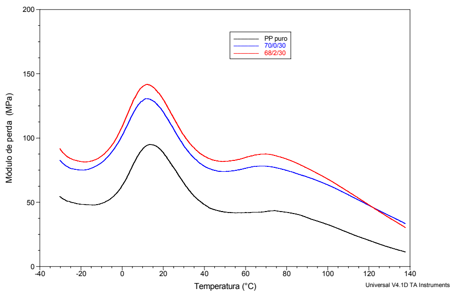
Figura 4.21 Efeito do PP-MA no módulo de perda dos compósitos com 30% de CA-A
