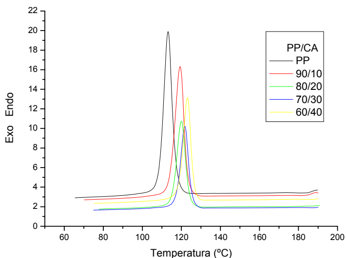
Figura 4.7 Termograma de resfriamento do PP e dos compósitos PP/CA-A
