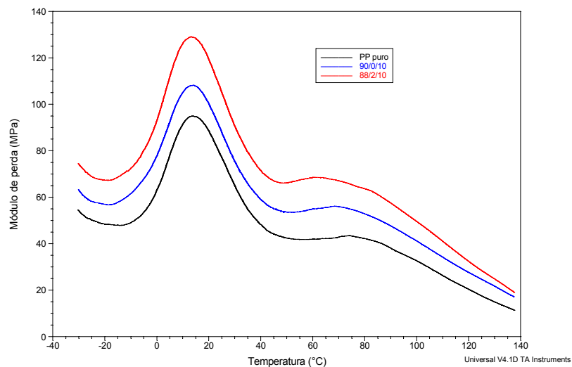
Figura 4.19 Efeito do PP-MA no módulo de perda dos compósitos com 10% de CA-A
