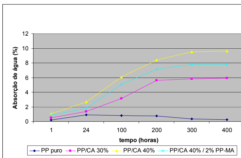
Figura 4.38 Absorção de água com a presença ou não de agente de compatibilização
