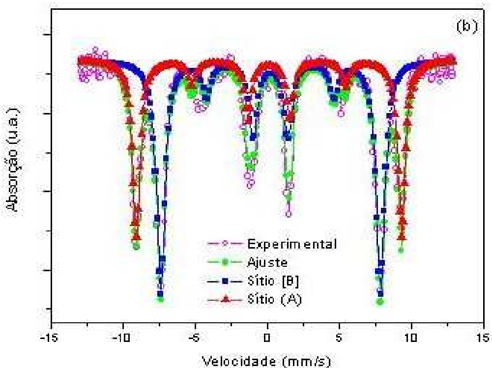
Figura 6.21 – Espectros Mössbauer a temperatura de 4,2 K da amostra de \text{MgFe}_2\text{O}_4 sintetizada a 650^\circ\text{C} (a) sem campo magnético externo e (b) campo magnético externo de 6T.
