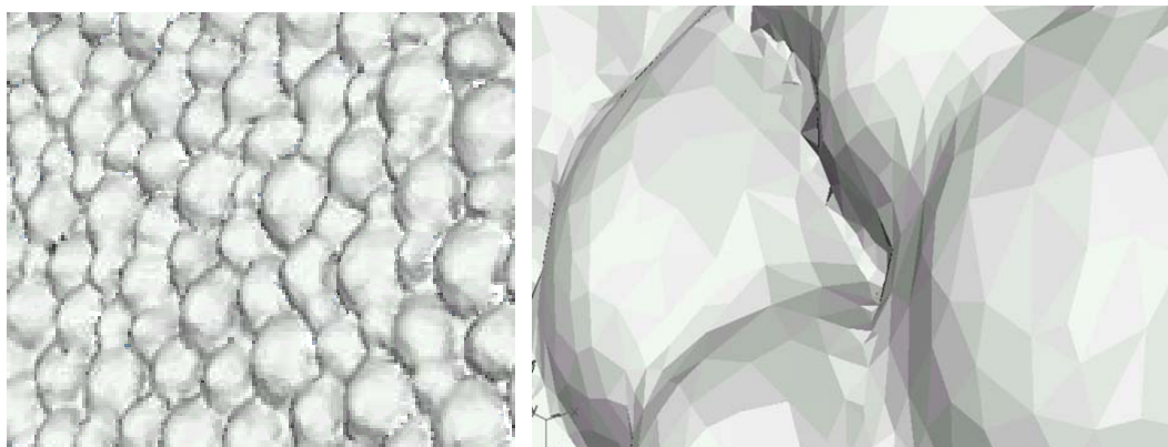
Figura 85 - Malha de triângulos obtidas a partir da nuvem de pontos.
