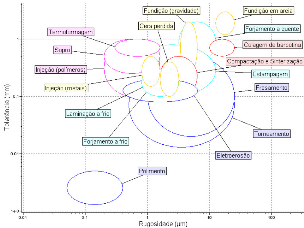
Figura 4 - Mapa de seleção de processos de fabricação: tolerância x rugosidade superficial. Fonte: realizado pelo autor com uso do software CES (2005).
