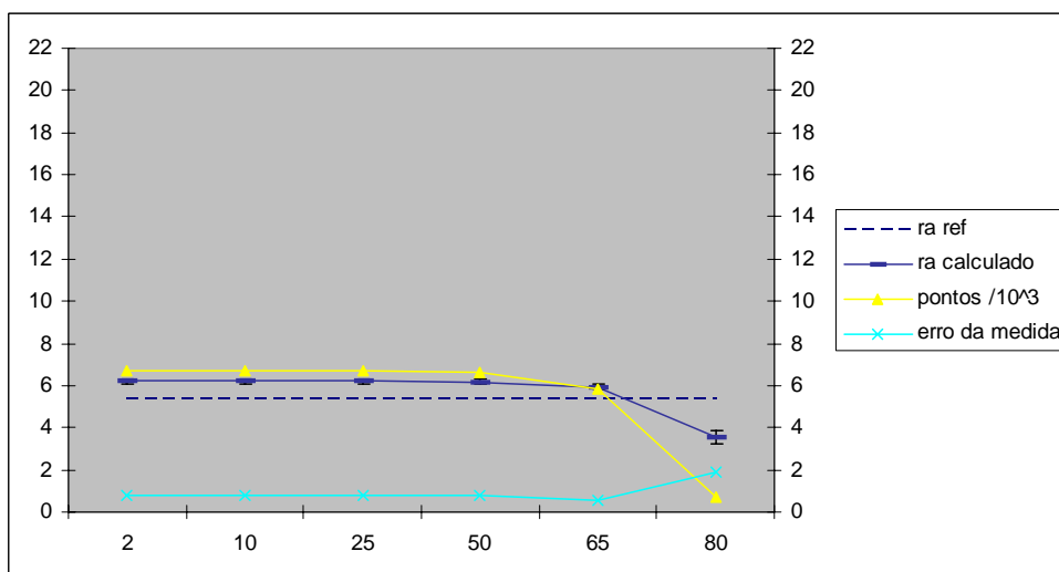
Figura 100 - Resultados para o padrão Rz 20 ( R_a = 5,4 \mu\text{m} ).
