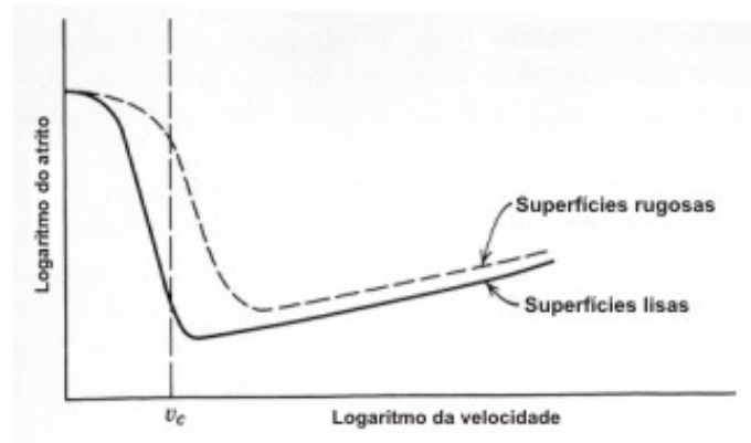
Figura 10 - Atrito em função da velocidade. Fonte: Rabinowicz (1965).
