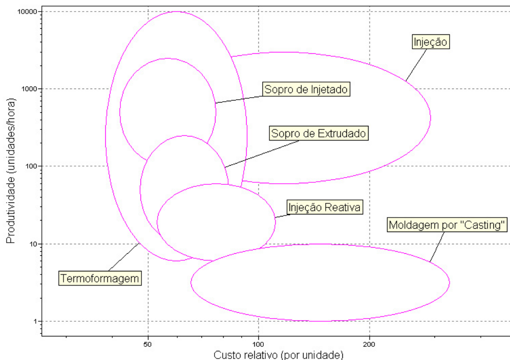
Figura 54 - Relação entre custo relativo por unidade fabricada e produtividade dos principais processos de fabricação de produtos poliméricos. Fonte: estudo realizado pelo autor através do software CES (2005).
