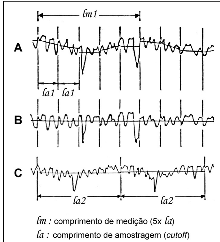
Figura 33 - Comprimentos de amostragem; (a) perfil primário, (b) perfil de rugosidade e (c) perfil de rugosidade com ondulação.
