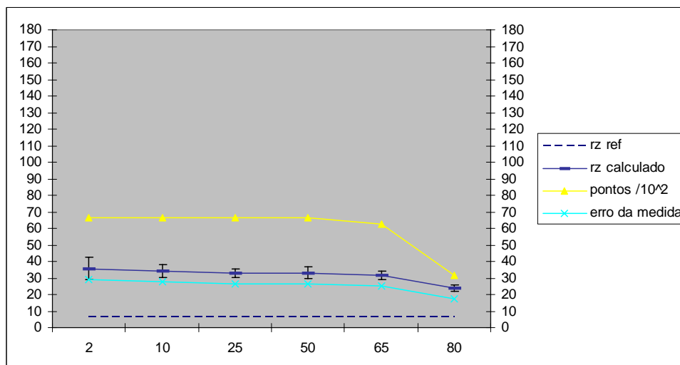
Figura 114 - Resultados para o padrão Rz 6,3 ( Rz = 6,5 \mu\text{m} ).
