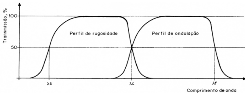
Figura 29 - Filtros para os perfis de rugosidade e ondulação. Fonte: NBR ISO 4287 (2002).
