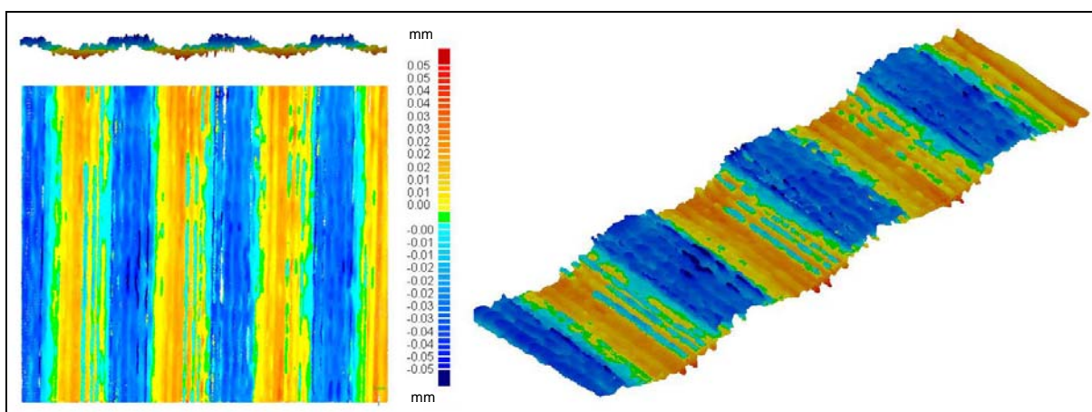
Figura 121 - Avaliação tridimensional da superfície do padrão Rz 80.
