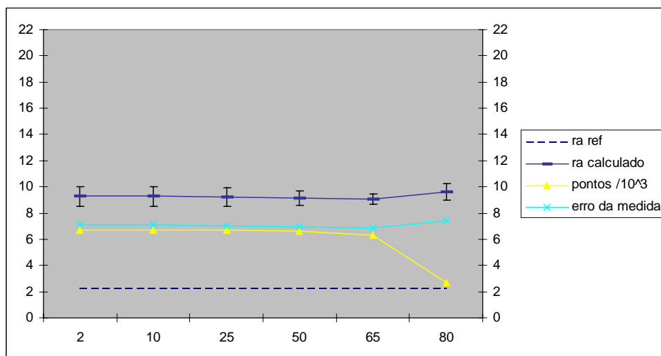
Figura 101 - Resultados para o padrão Rz 10 ( R_a = 2,2 \mu\text{m} ).
