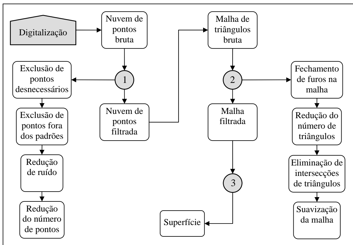
Figura 86 - Processamento da nuvem de pontos obtida através da digitalização 3D a Laser.
