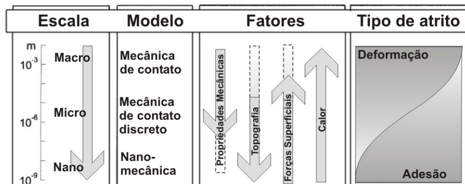
Figura 37 - Escalas de rugosidade e sua influência na fricção. Fonte: Myshkin (1998).
