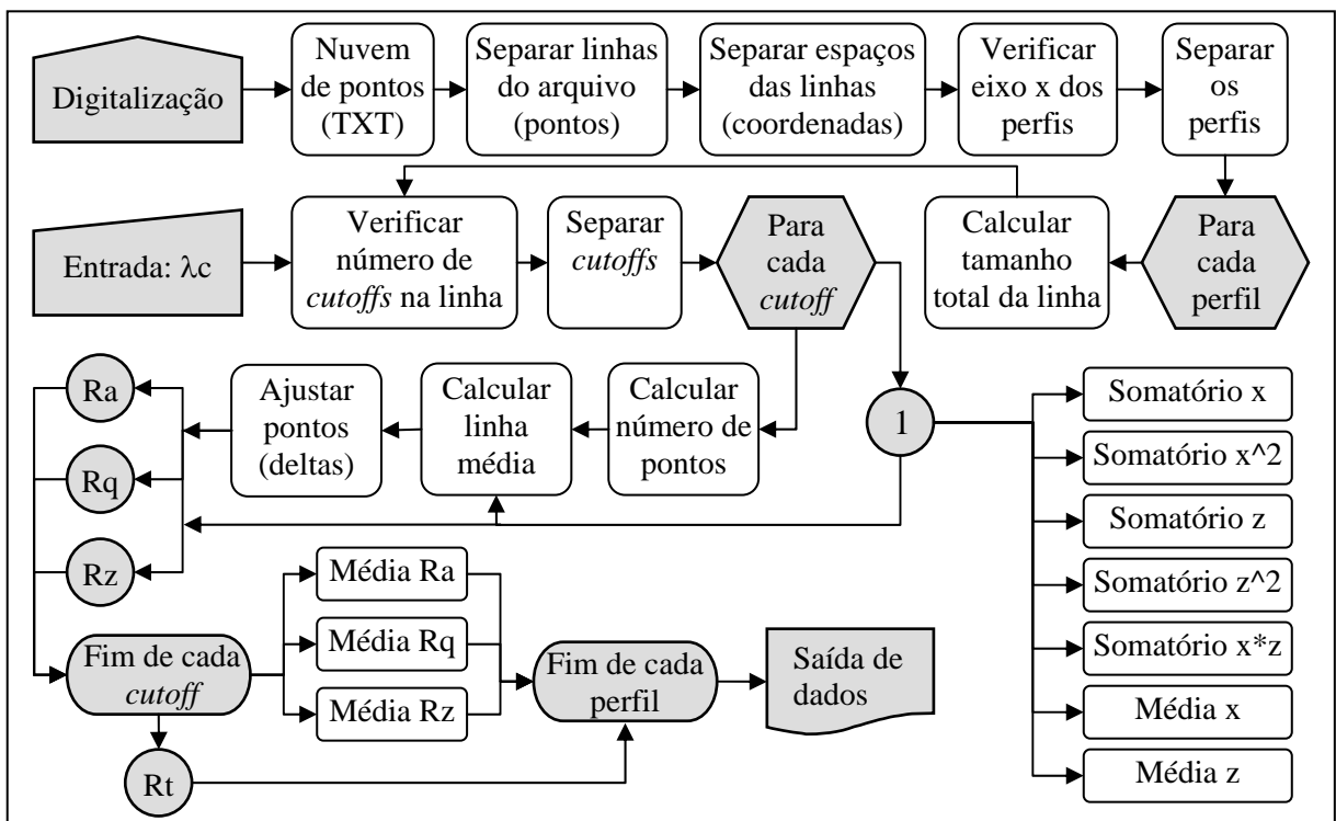
Figura 74 - Processamento da nuvem de pontos para cálculo de parâmetros de rugosidade.
