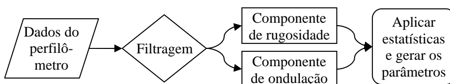
Figura 30 - Algoritmo para o procedimento de filtragem
