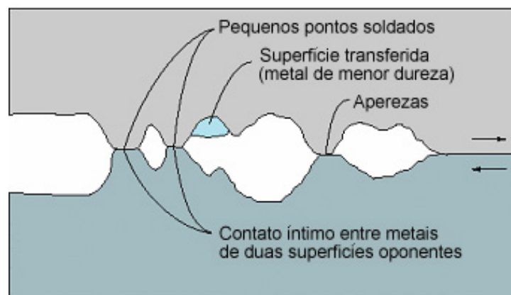
Figura 8 - Desgaste adesivo. Fonte: Mendes (2006).
