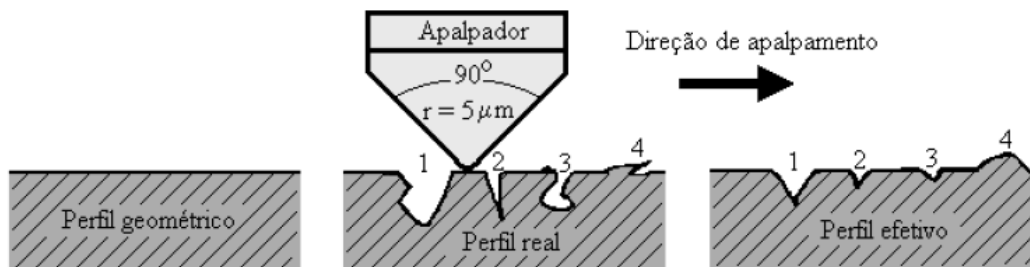
Figura 27 - Perfil geométrico, real e efetivo. Fonte: Silva (2002).
