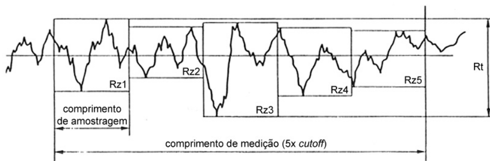
Figura 36 - Representação gráfica do perfil indicando o parâmetro R_t .
