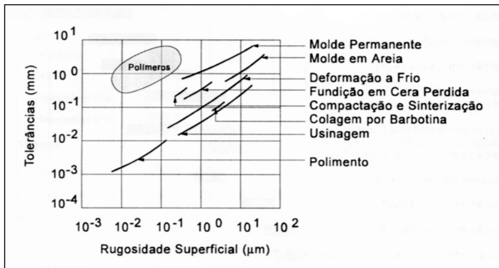
Figura 3 - Tolerâncias e Rugosidade Superficial. Fonte: Ferrante (1996).
