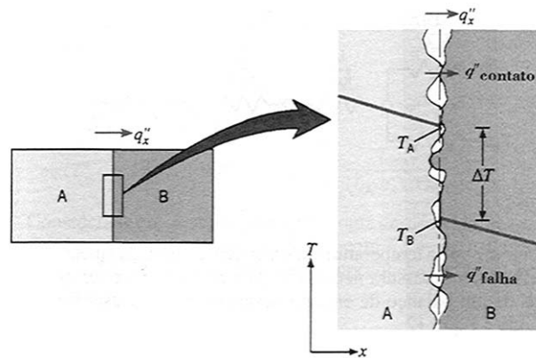
Figura 20 - Resistência térmica de contato. Fonte: Incropera & DeWitt (1998).
