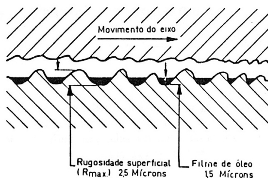
Figura 11 - Rugosidade e lubrificação. Fonte: González (1998).
