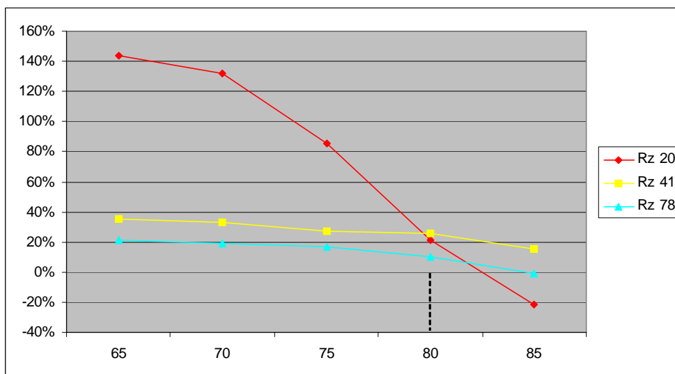
Figura 119 - Erro(%) x qualidade mínima admissível para nova análise do Rz.
