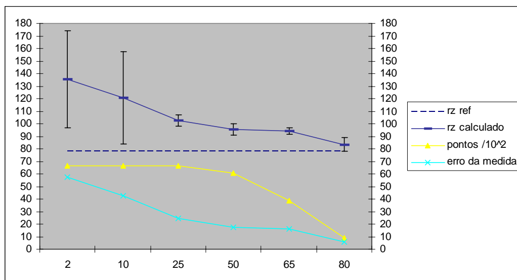
Figura 110 - Resultados para o padrão Rz 80 ( Rz = 78 \mu\text{m} ).
