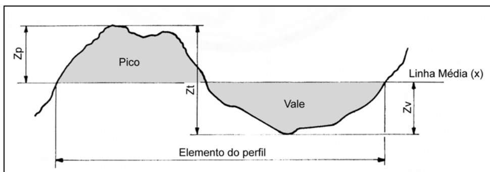
Figura 34 - Elemento do perfil.
