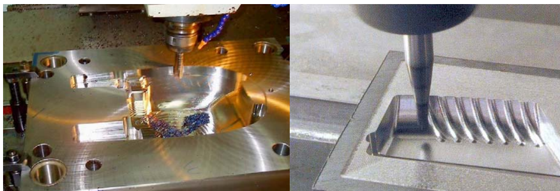
Figura 63 - Usinagem de moldes para injeção. Fonte: Ho-Yo (2006) e Fer-Plastic (2006), respectivamente.
