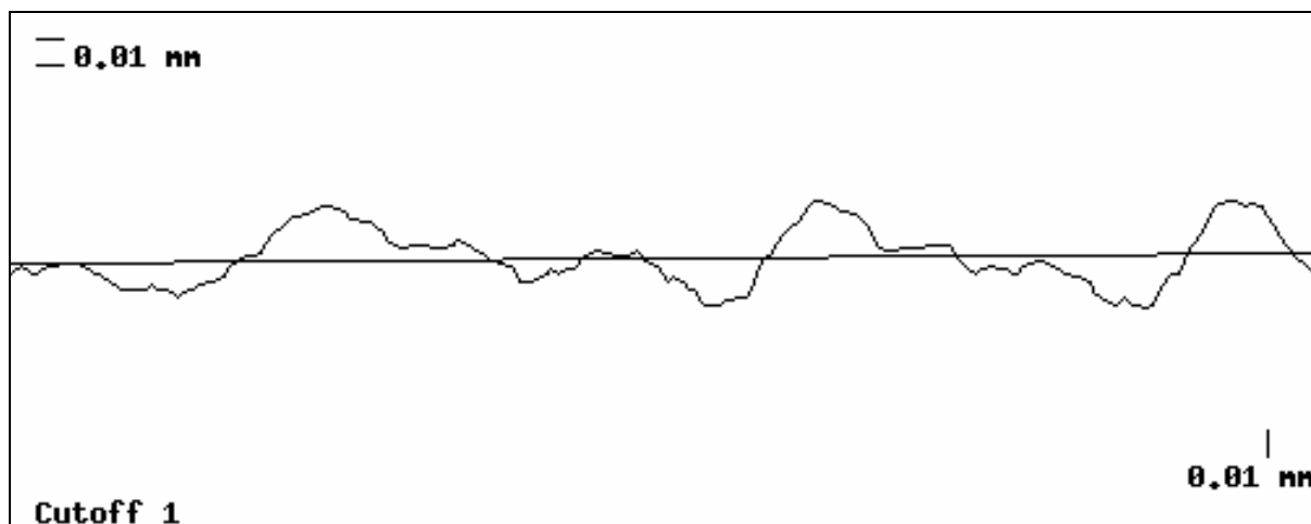
Figura 96 - Perfil obtido do padrão Rz 3,2µm, cutoff=0,25mm , escala x=2000X y=1000X .
