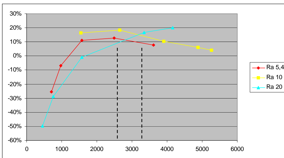
Figura 108 - Erro(%) x nº de pontos adquiridos na nova análise do Ra.
