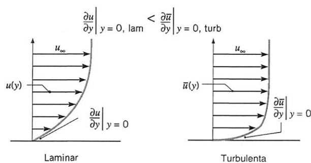
Figura 22 - Perfis de velocidade para escoamento laminar e turbulento. Fonte: Incropera & DeWitt (1998).
