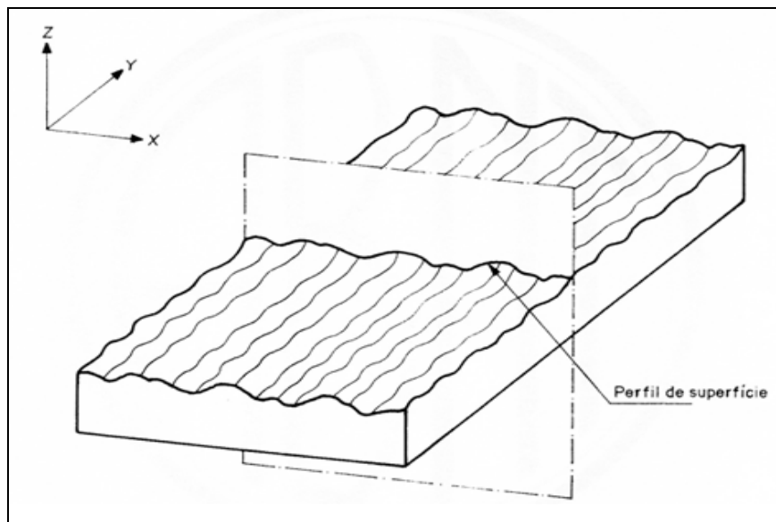
Figura 26 - Perfil de superfície. Fonte: NBR ISO 4287 (2002).
