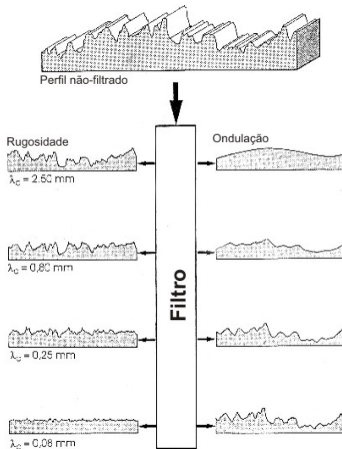
Figura 31 - Perfis de rugosidade e ondulação de acordo com o filtro \lambda_c utilizado. Fonte: Mummery (1992).
