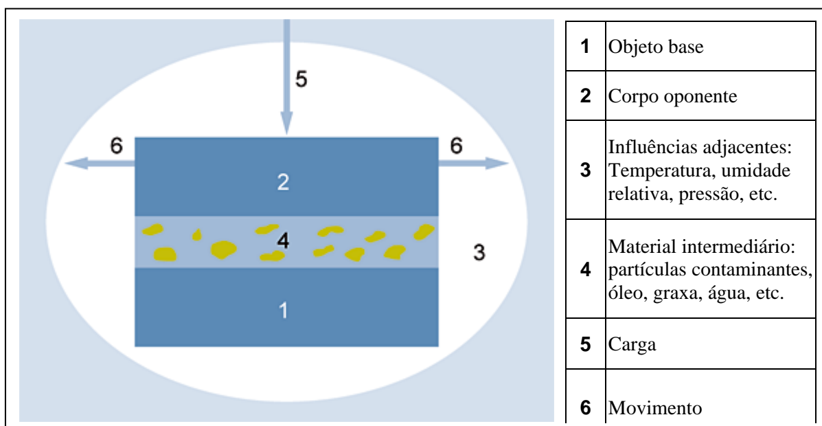
Figura 7 - Sistema Tribológico. Fonte: Balzers (2005).
