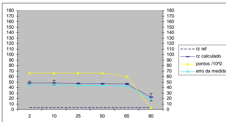
Figura 115 - Resultados para o padrão Rz 3,2 ( Rz = 3,5 \mu\text{m} ).
