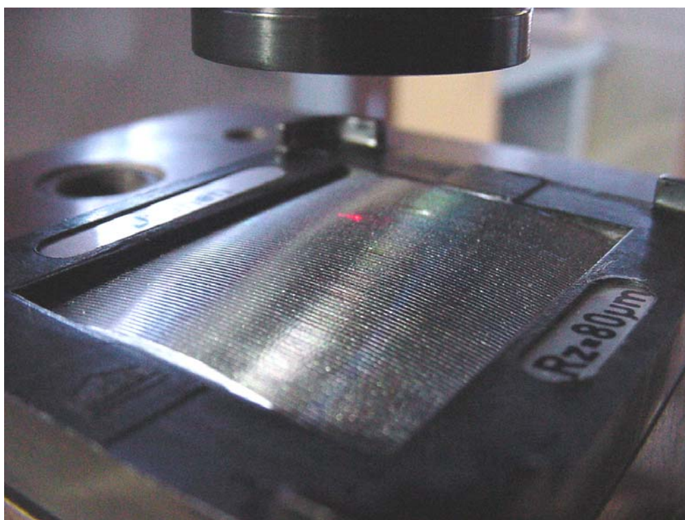
Figura 81 - Digitalização do Padrão Rz 80 \mu\text{m} .
