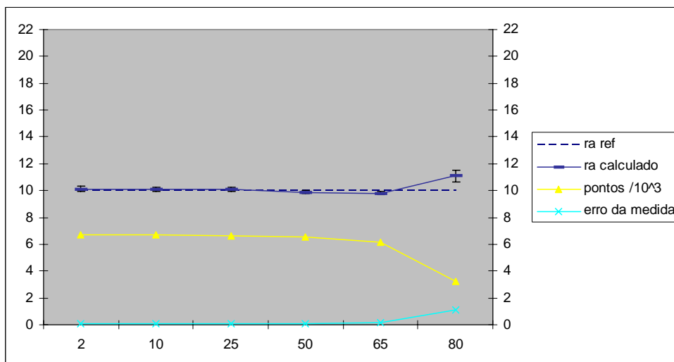
Figura 99 - Resultados para o padrão Rz 40 ( R_a = 10 \mu\text{m} ).
