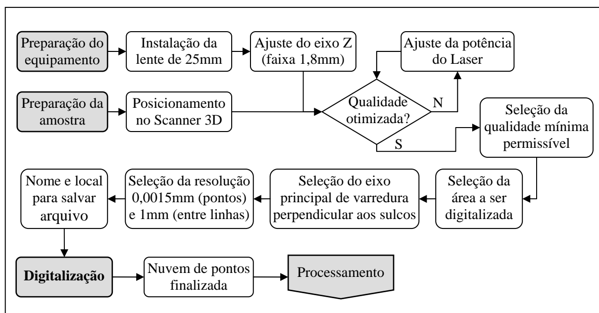
Figura 70 - Procedimentos para a digitalização dos padrões de rugosidade.
