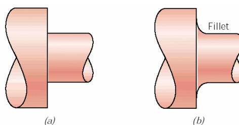
Figura 13 - Utilização de raios ao invés de entalhes para minimizar a fadiga.
