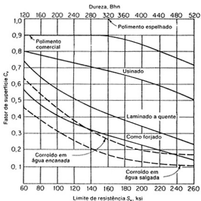
Figura 14 - Fator de redução do limite de fadiga devido a vários tratamentos superficiais. Fonte: Strohaecker (2003).
