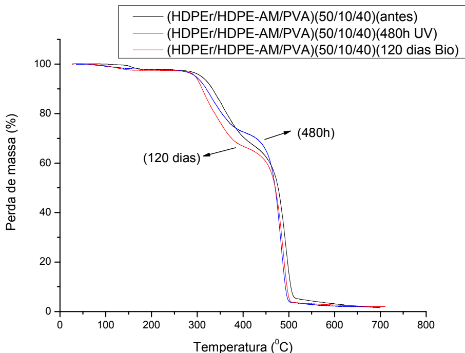
Figura 71 – Curva de perda de massa da mistura HDPEr/HDPE-AM/PVA com composição 50/10/40, antes e após processos de degradação por irradiação (480 horas UV) e biodegradação (120 dias).
