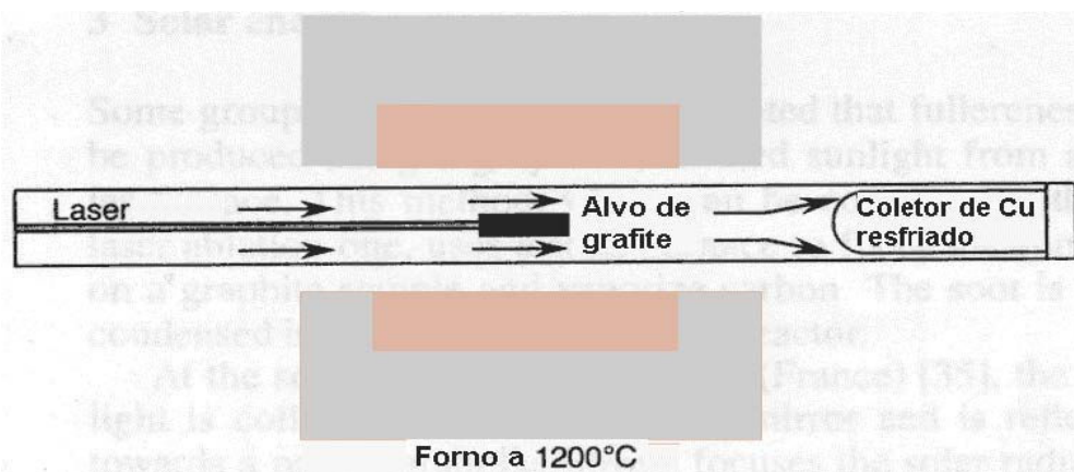
Figura 3-2 - Representação esquemática do equipamento de vaporização por laser utilizado na Rice University (Houston, Texas, USA).
