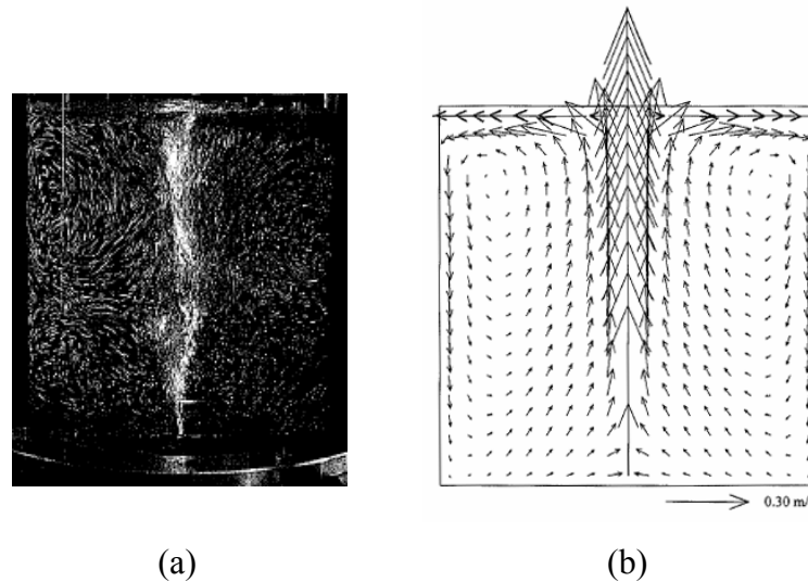
Figura 8 - (a) Visualização do escoamento através de um plano laser. (b) Campo de vetores velocidade obtidos numericamente (Zhu et al, 1995).
