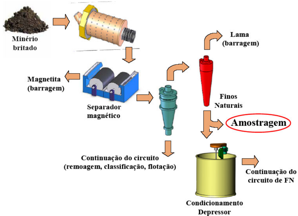
Figura 3.1. Ponto de coleta da amostra de Finos Naturais na usina de concentração.
