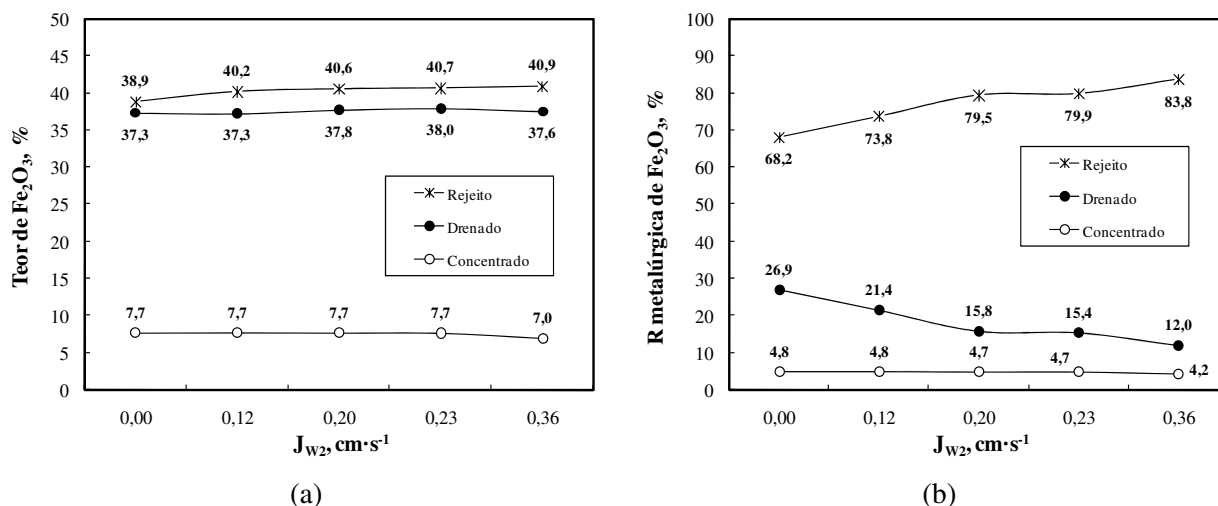
Figura 4.51. Efeito da variação de J_{w2} sobre o teor de \text{Fe}_2\text{O}_3 (a) e distribuição (b) nos fluxos do concentrado, drenado e rejeito para ensaios em C3P (média de duas amostragens). Condições: % sólidos no condicionamento = 39; % sólidos na alimentação = 25; h espuma = 70\pm 1 cm; pH no condicionamento = 11,6; Dosagem de fubá de milho gelatinizado = 1400 \text{ g}\cdot\text{t}^{-1} ; Dosagem de sabão de óleo de soja = 70 \text{ g}\cdot\text{t}^{-1} ; J_{gs} = 0,52 \text{ cm}\cdot\text{s}^{-1} ; J_w = 0,37 \text{ cm}\cdot\text{s}^{-1} ; Tempo de condicionamento com depressor = 15 min; Tempo de condicionamento com o coletor = 9 min.
