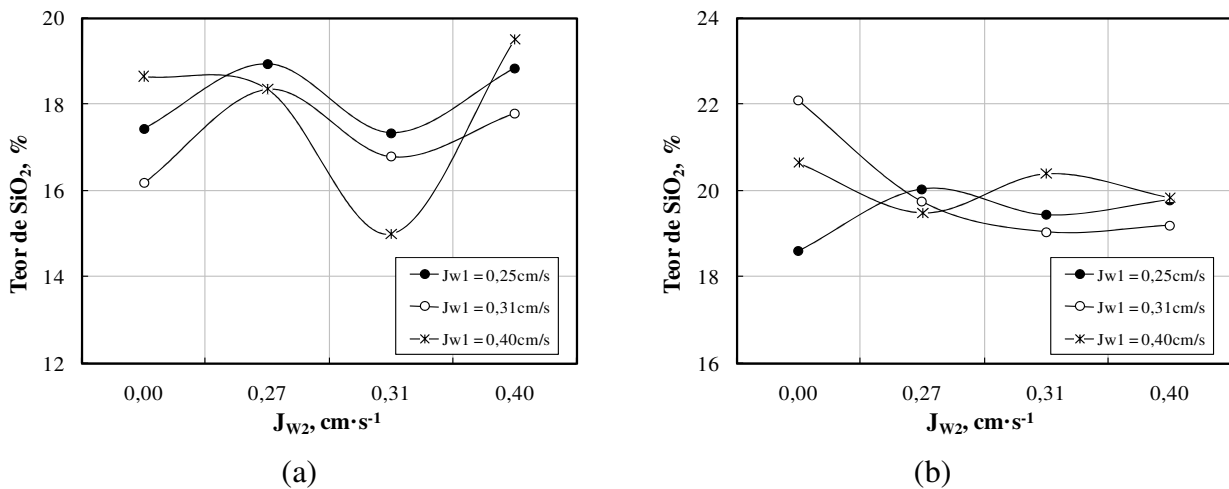
Figura 4.27. Efeito da variação de J_{W1} e J_{W2} sobre o teor de \text{SiO}_2 no drenado (a) e no rejeito (b). Condições: Altura da camada de espuma = 18 cm; Dosagem de sabão de óleo de soja = 60 \text{ g}\cdot\text{t}^{-1} , Dosagem de fubá de milho gelatinizado = 1200 \text{ g}\cdot\text{t}^{-1} , % sólidos no condicionamento = 40%; % sólidos na alimentação = 15%, J_a = 0,66 \text{ cm}\cdot\text{s}^{-1} , J_g = 0,49 \text{ cm}\cdot\text{s}^{-1} , pH de condicionamento = 12.
