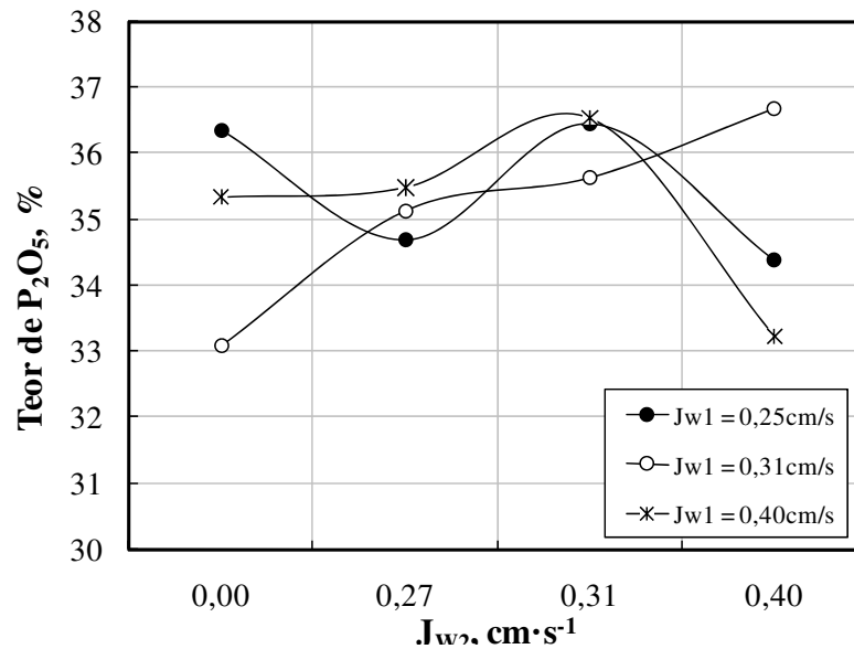
Figura 4.22. Efeito da variação de J_{w1} e J_{w2} sobre o teor de \text{P}_2\text{O}_5 na corrente do concentrado. Condições: Altura da camada de espuma = 18 cm; Dosagem de sabão de óleo de soja = 60 \text{ g}\cdot\text{t}^{-1} , Dosagem de fubá de milho gelatinizado = 1200 \text{ g}\cdot\text{t}^{-1} , % sólidos no condicionamento = 40%; % sólidos na alimentação = 15%, J_a = 0,66 \text{ cm}\cdot\text{s}^{-1} , J_g = 0,49 \text{ cm}\cdot\text{s}^{-1} , pH de condicionamento = 12.
