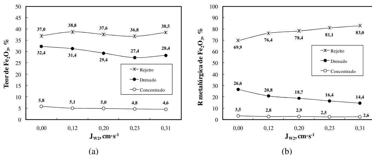
Figura 4.55. Efeito da variação de J_{w2} sobre o teor de \text{Fe}_2\text{O}_3 (a) e distribuição (b) nos fluxos do concentrado, drenado e rejeito para ensaios em C3P (média de duas amostragens). Condições: % sólidos no condicionamento = 40; % sólidos na alimentação = 25; h espuma = 70\pm 1 cm; pH no condicionamento = 12,0; Dosagem de fubá de milho gelatinizado = 1400\text{ g}\cdot\text{t}^{-1} ; Dosagem de sabão de óleo de soja = 70\text{ g}\cdot\text{t}^{-1} ; J_g = 0,52\text{ cm}\cdot\text{s}^{-1} ; J_w = 0,37\text{ cm}\cdot\text{s}^{-1} ; Tempo de condicionamento com depressor = 17 min; Tempo de condicionamento com o coletor = 10 min.
