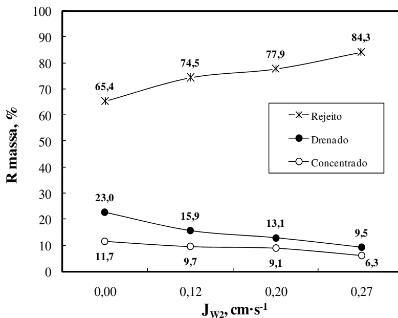
Figura 4.57. Recuperação em massa para C3P. Condições: % sólidos no condicionamento = 40; % sólidos na alimentação = 25; h espuma = 70\pm 1\text{cm} ; pH no condicionamento = 12,0; Dosagem de fubá de milho gelatinizado = 1400\text{ g}\cdot\text{t}^{-1} ; Dosagem de sabão de óleo de soja = 70\text{ g}\cdot\text{t}^{-1} ; J_g = 0,52\text{ cm}\cdot\text{s}^{-1} ; J_w = 0,37\text{ cm}\cdot\text{s}^{-1} ; Tempo de condicionamento com depressor = 17 min; Tempo de condicionamento com o coletor = 10 min.
