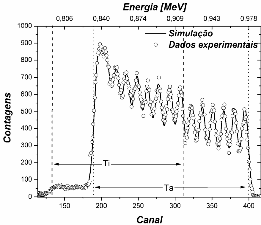
Figura 37: Espectro simulado e experimental de RBS para a amostra TaTiN H . Um \Lambda_{\text{m\u00e9dio}} \approx 23 nm foi obtido para periodicidade da amostra.
