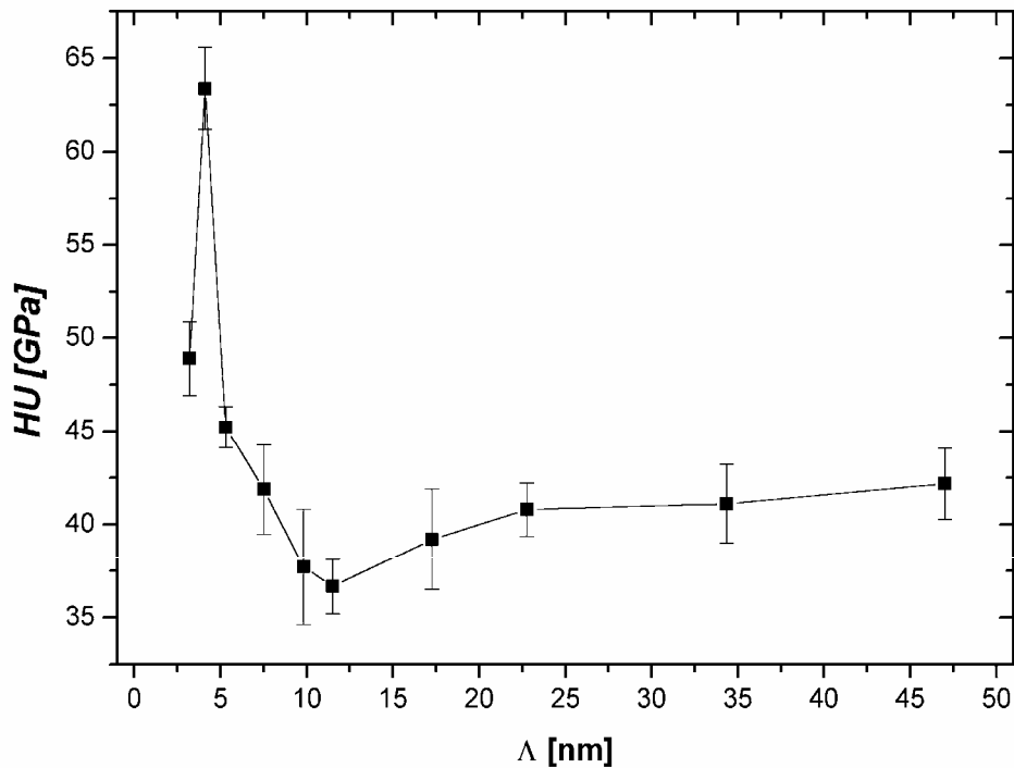
Figura 42: Valores de dureza HU obtidos para as amostras de Ta/TiN apresentados em função de \Lambda . Foi detectado um valor máximo de aproximadamente 63 GPa.
