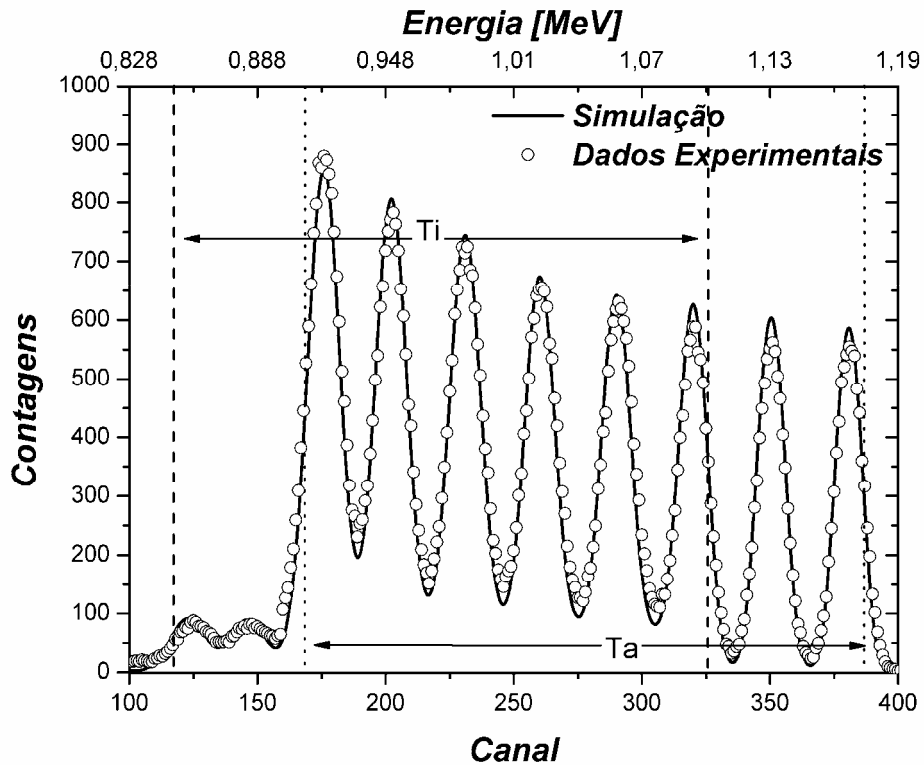
Figura 35: Espectros simulado e experimental de RBS para a amostra TaTiN_J. Foi obtido um \Lambda_{\text{médio}} = 47 nm.
