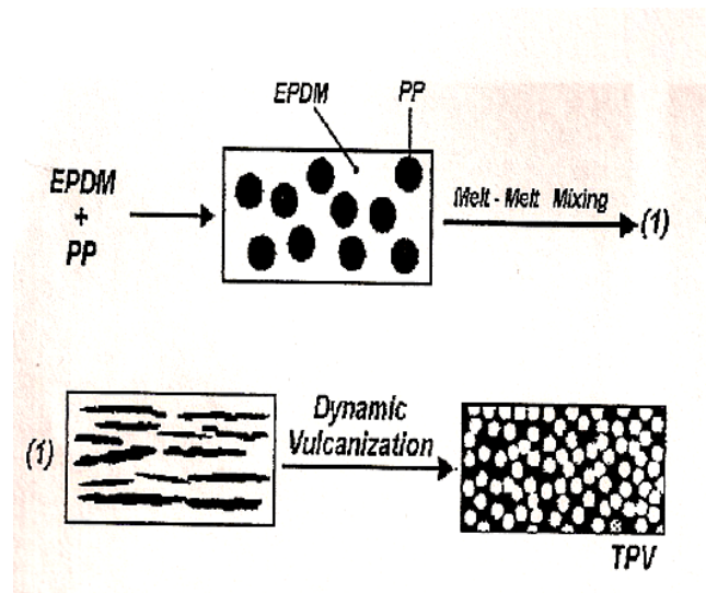
Figura 11. Partículas dispersas de elastômero na matriz contínua plástica [46]
