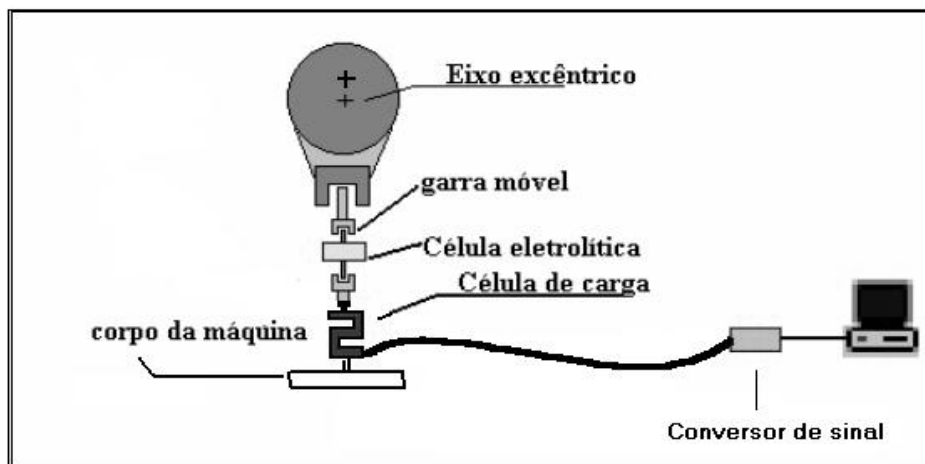
Figura 12 – Desenho esquemático da máquina de fadiga e sistema de aquisição.
