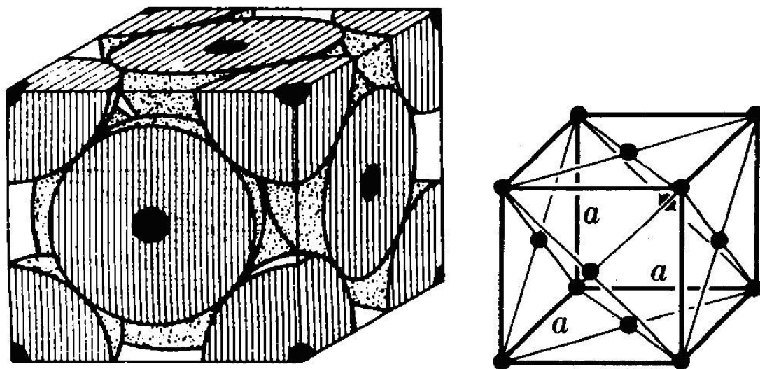
Figura 2 Sistema cristalino cúbico de face centrada (8)
