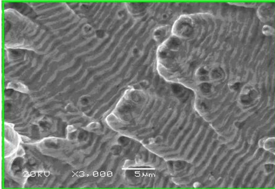
Figura 28 - Desenvolvimento de trinca típica de fadiga (reg.II -fig.7-cap.2)
