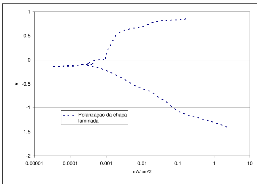
Figura 19 - Curvas potenciostáticas do Inconel 625 em forma de chapa, em solução 115000 ppm de Cl -
