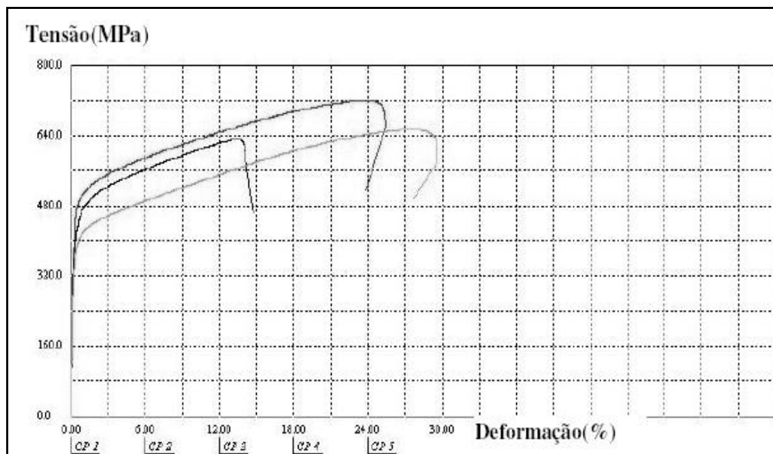
Figura 15 - Tração do material de solda (19)
