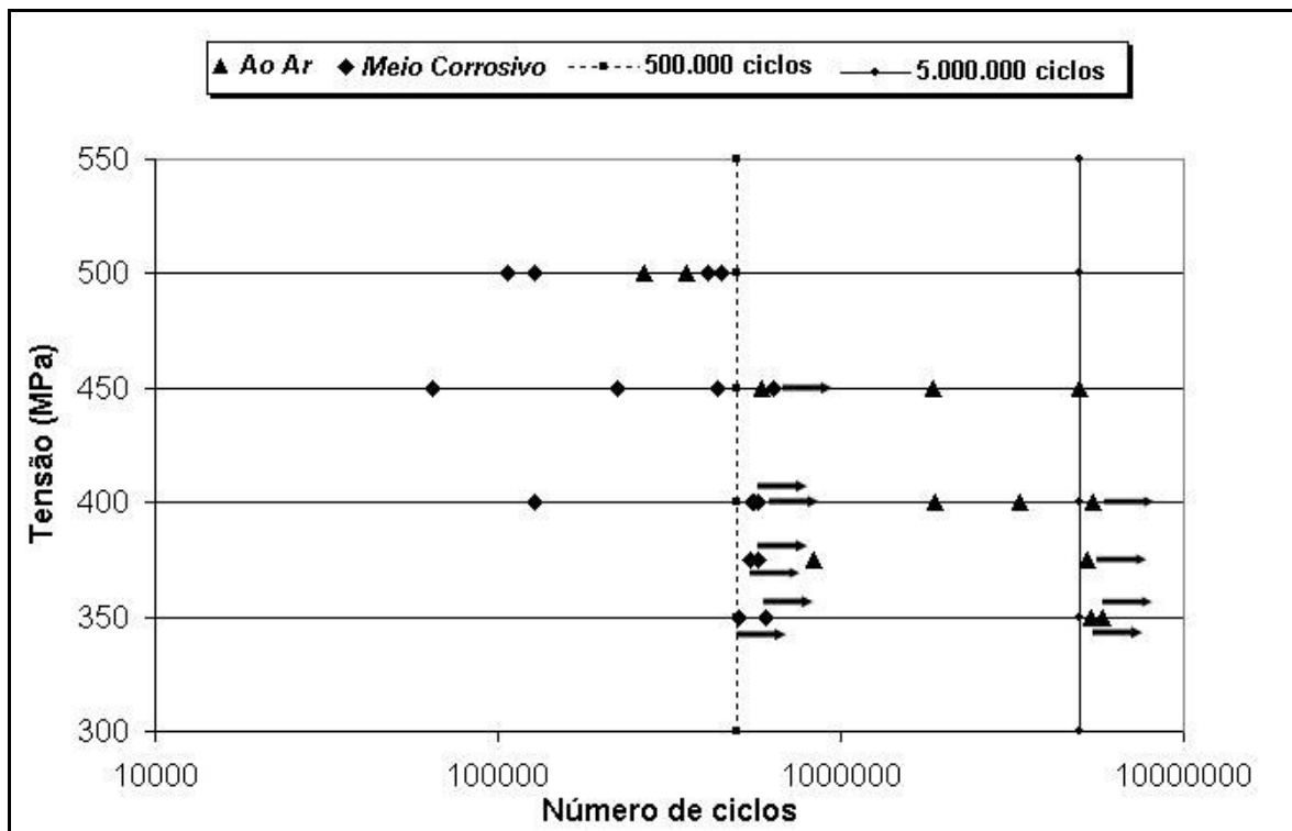
Figura 6 - SxN do depósito de solda (eletrodos revestidos) (19)
