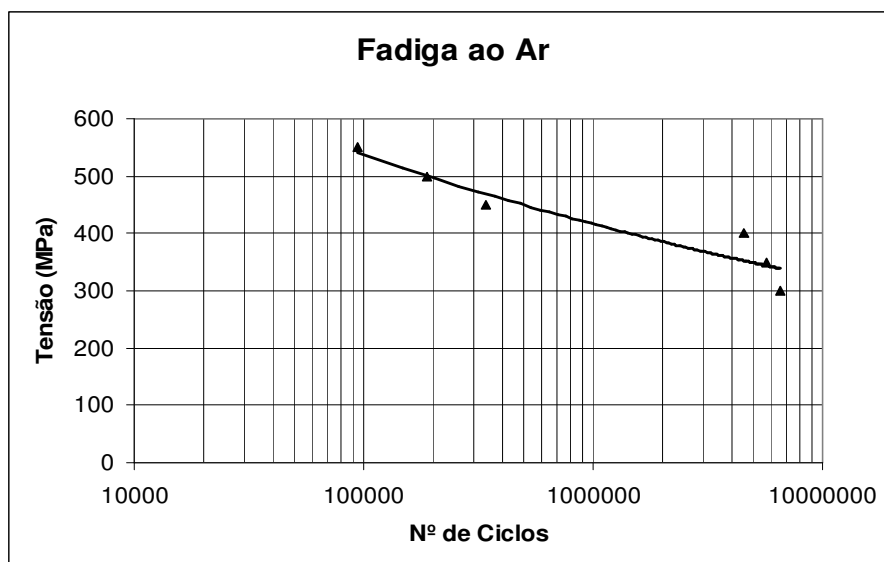
Figura 17 - Curva de fadiga ao ar da junta soldada
