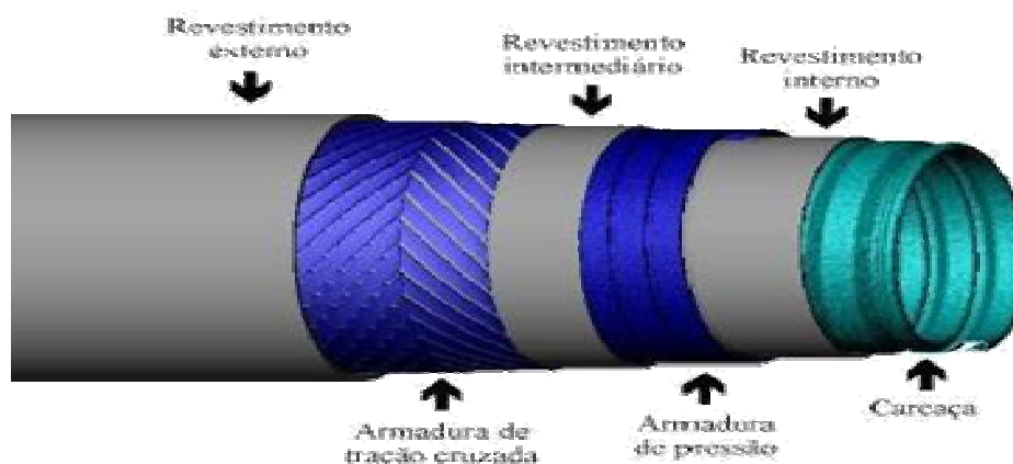
Figura 1 Riser flexível mostrando em corte a configuração de armaduras, carcaça e revestimentos poliméricos.
