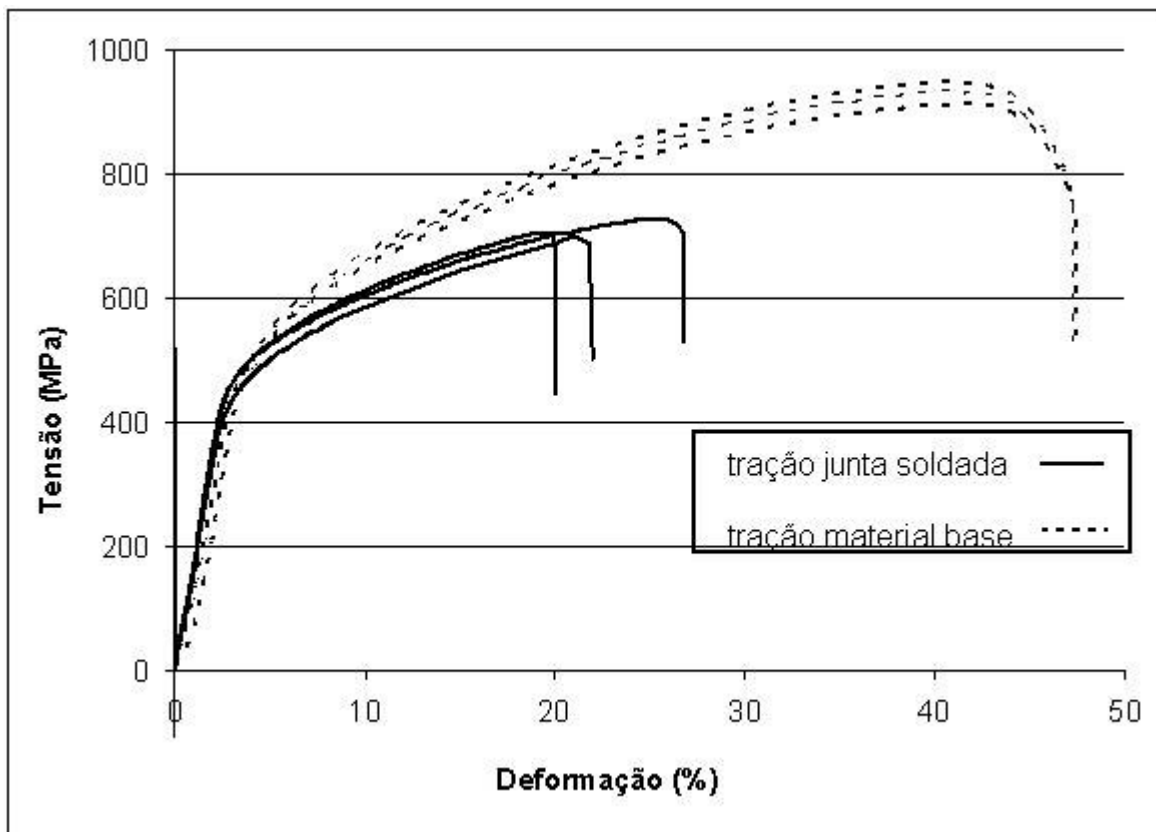
Figura 36 Comparações de Curvas de Tração
