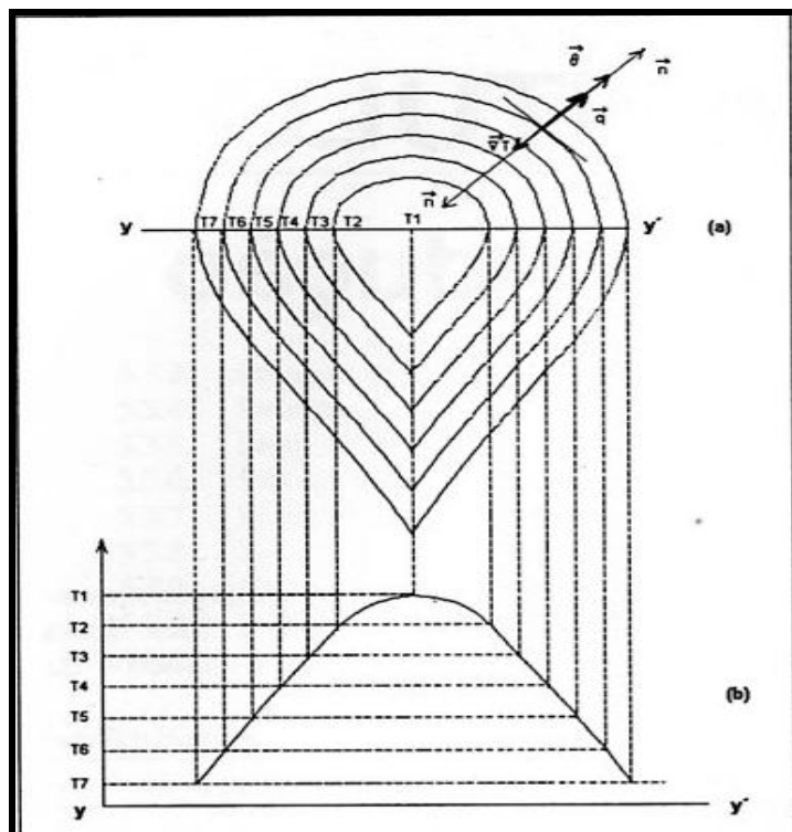
Figura 8 (a) Seções transversais de superfícies isotérmicas, (b) Gradiente de temperatura. (23)
