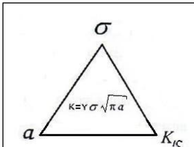
Figura 5 Triângulo da mecânica da fratura mostrando como estão correlacionados o carregamento aplicado, o tamanho crítico do defeito e a Tenacidade a fratura (fator de intensidade de tensões crítico) que é uma propriedade do material. (11)
