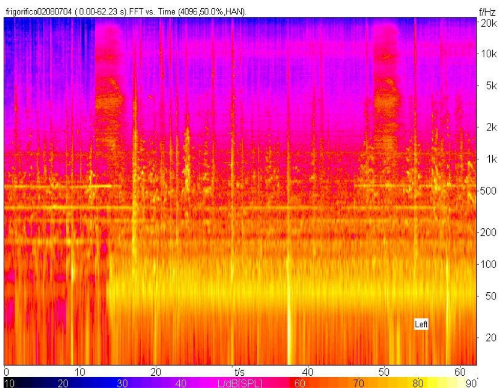
Figura 70: Espectrograma do ruído na sala de desossa, medido no ouvido externo de um trabalhador no posto de desossa (posto 4). O eixo x representa o tempo, o eixo y a frequência e as cores representam o nível de pressão sonora em função do tempo e da frequência.
