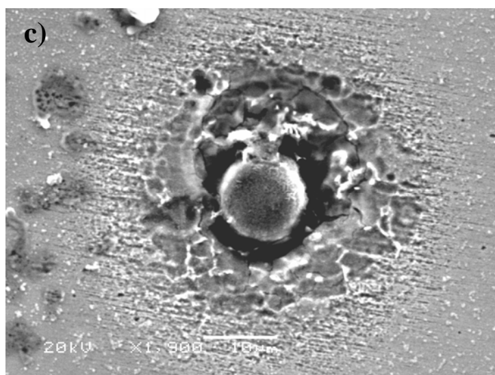
Figura 34. MEV do pite associado a inclusões do aço API 5L X56 em diferentes aumentos (a) x50, (b) x250 e (c) x1900. Amostra submetida ao extrato aquoso do solo 4 exposto a aproximadamente 3h no potencial de corrosão (imagem por elétrons secundários).
