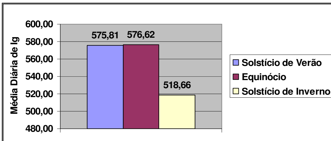
Figura 5.13 - Média diária de radiação solar, para os solstícios e equinócio – 05% Leste (W/m 2 )
