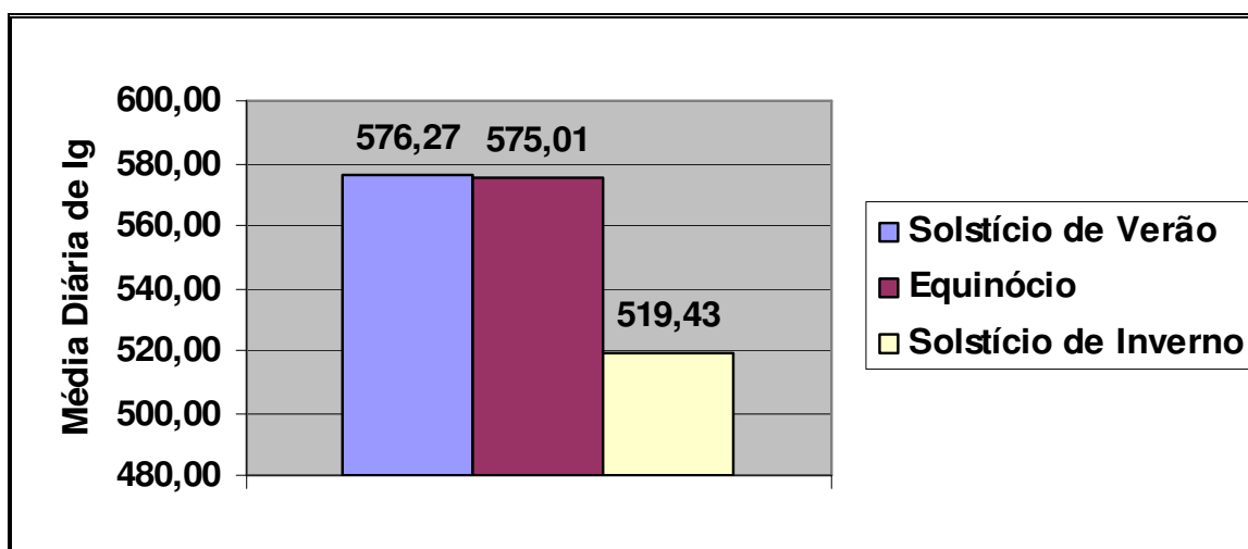
Figura 5.11 - Média diária de radiação solar, para os solstícios e equinócio – 10% Oeste (W/m 2 )
