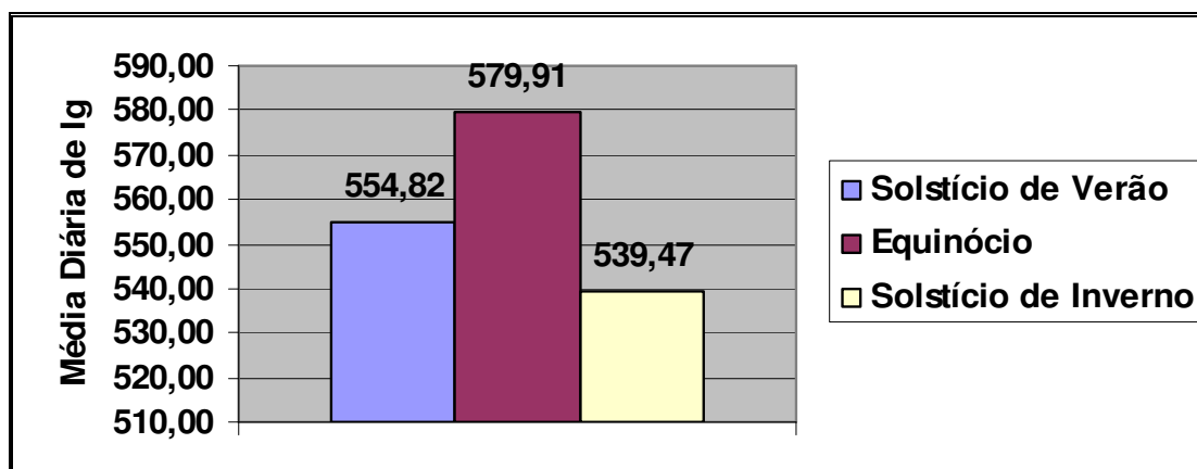
Figura 5.8 - Média diária de radiação solar, para os solstícios e equinócio – 10% Norte (W/m 2 )
