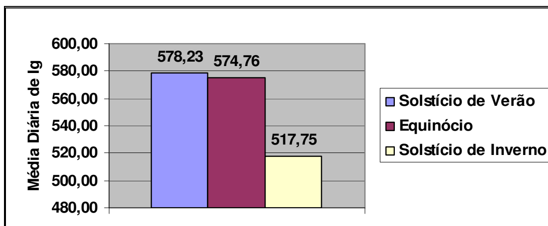
Figura 5.9 - Média diária de radiação solar, para os solstícios e equinócio – 10% Leste (W/m 2 )
