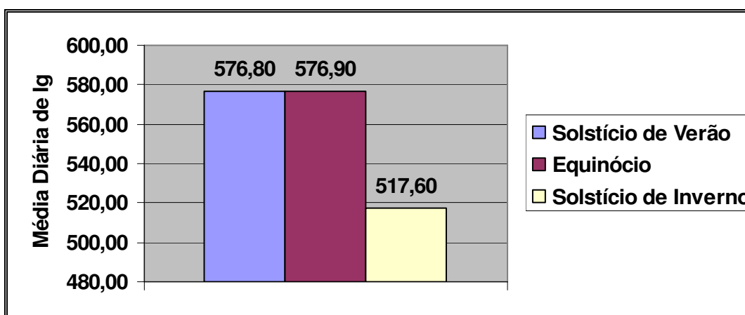
Figura 5.15 - Média diária de radiação solar, para os solstícios e equinócio – 05% Oeste (W/m 2 )
