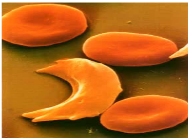
FIGURA 1 - HEMÁCIA FALCIZADA
