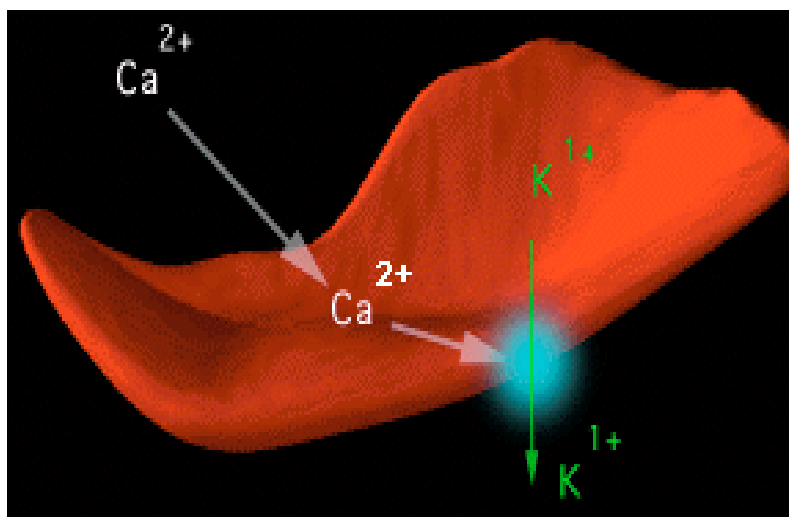
FIGURA 2 - REPRESENTAÇÃO ESQUEMÁTICA DA ATIVIDADE DO CANAL DE GARDOS NA HEMÁCIA FALCIFORME
