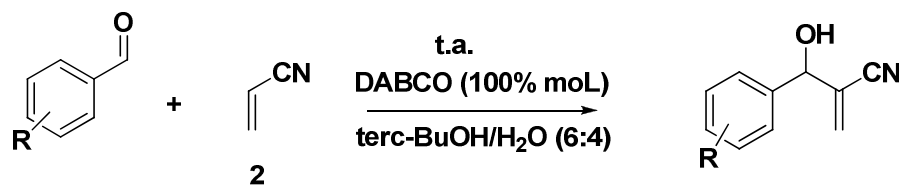
Esquema 4.1: Metodologia inicial para a síntese de 29 , 31 , 13 , 33 , 14 , 36 , 25 e 26 .
