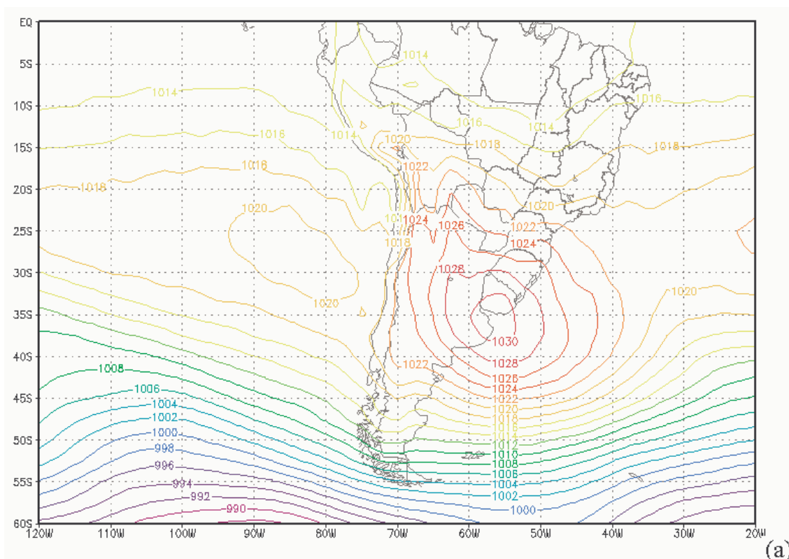
FIGURA 3.20 – (a) P (hPa), (b) Z (m) em 500 hPa, (c) CJ ( m s^{-1} ) e LC em 250 hPa, (d) UR (%) em 925 hPa e T ( ^{\circ}C ) (e) em 700 hPa e (f) em 850 hPa. Estes campos são obtidos a partir da média diária dos 4 horários sinóticos e da média de 15 casos de neve, referentes a quinta classe identificada empiricamente.
