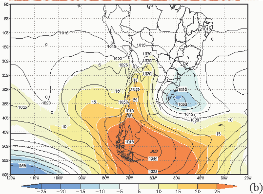
FIGURA 3.2 – (a) Imagem do satélite GOES-12 das 09:00 TMG e média diária (linha cheia) e anomalia (áreas colorida) da (b) P (hPa) e (c) de Z (mgp) em 500 hPa, para o dia 11 de julho de 2000.
