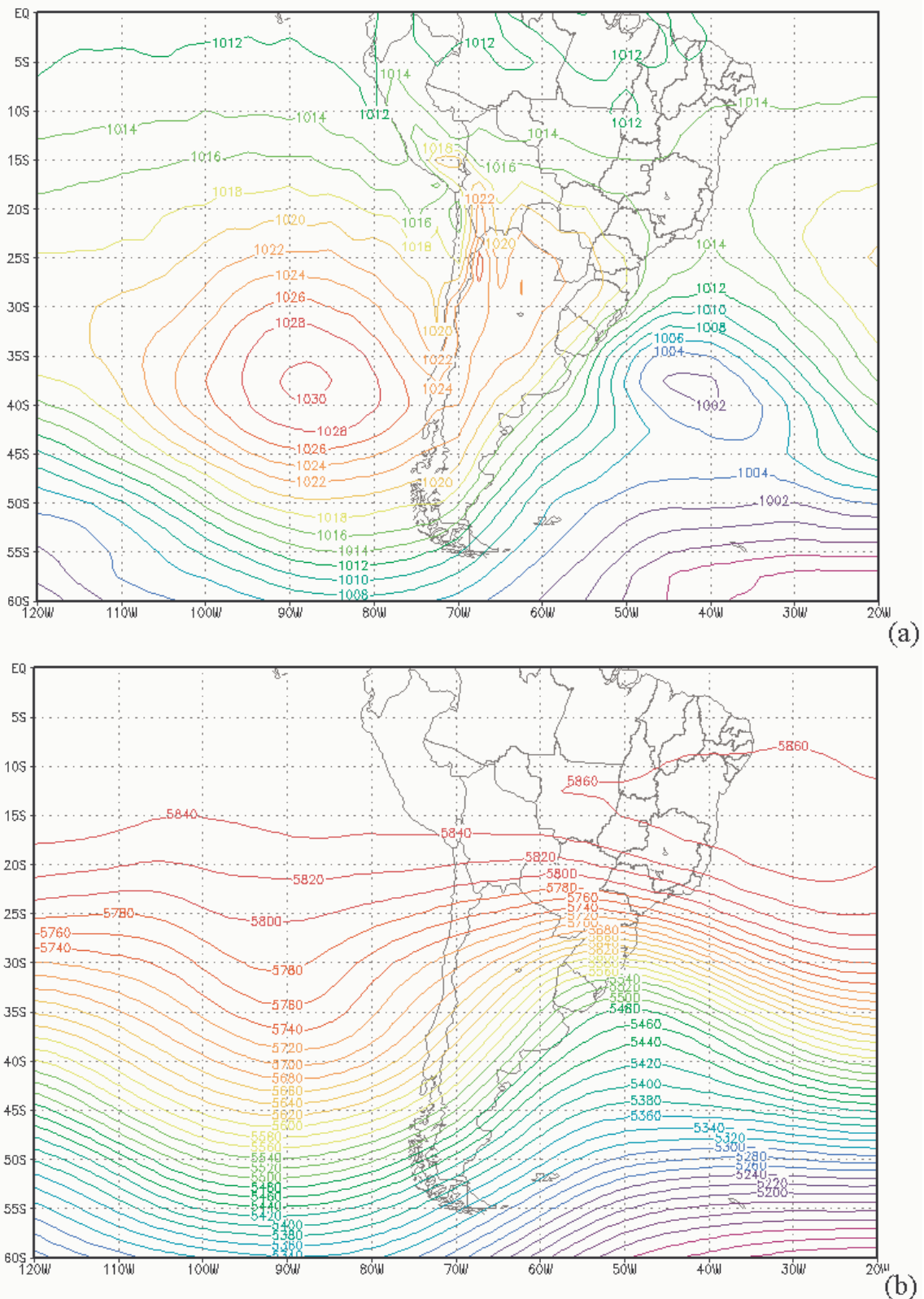
FIGURA 3.22 – (a) P (hPa), (b) Z (mgp) em 500 hPa, (c) CJ ( m s^{-1} ) e LC em 250 hPa, (d) UR (%) em 925 hPa e T ( ^{\circ}C ) (e) em 700 hPa e (f) em 850 hPa. Estes campos são obtidos a partir da média diária dos 4 horários sinóticos e da média dos 12 casos de neve, referentes a sétima classe identificada empiricamente.
