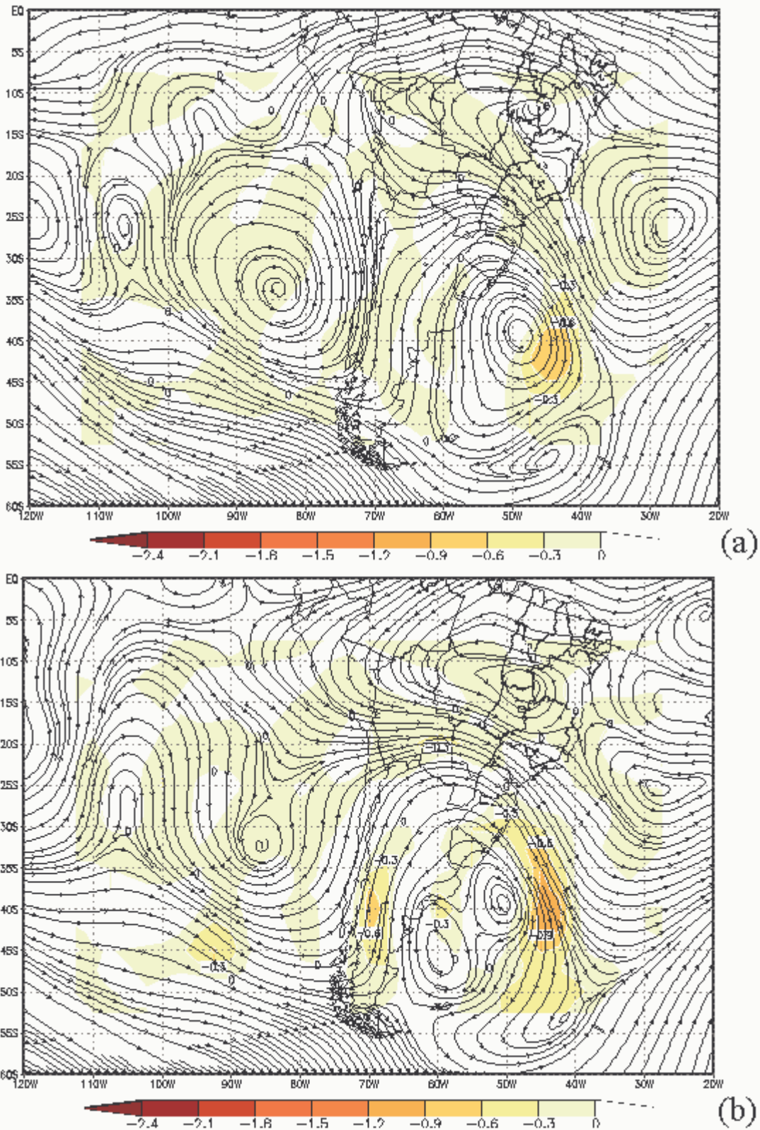
FIGURA 3.7 – Média diária da DVQ (áreas coloridas) e LC em (a) 700 hPa e (b) 500 hPa, e (c) CJ (áreas coloridas) e LC em 200 hPa para o dia 12 de julho de 2000. Os valores nas legendas de (a) e (b) estão em \times 10^{-17} \text{ m s}^{-1} \text{ kg}^{-1} e de (c) estão em \text{m s}^{-1} .
