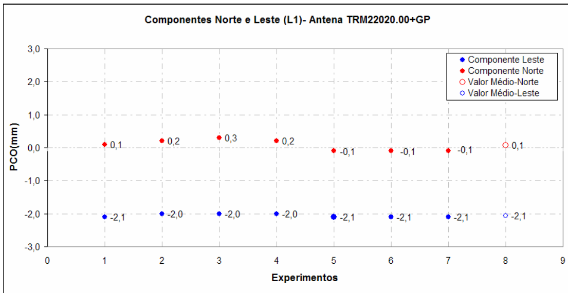
FIGURA 62 - COMPONENTE NORTE E LESTE (L1)
