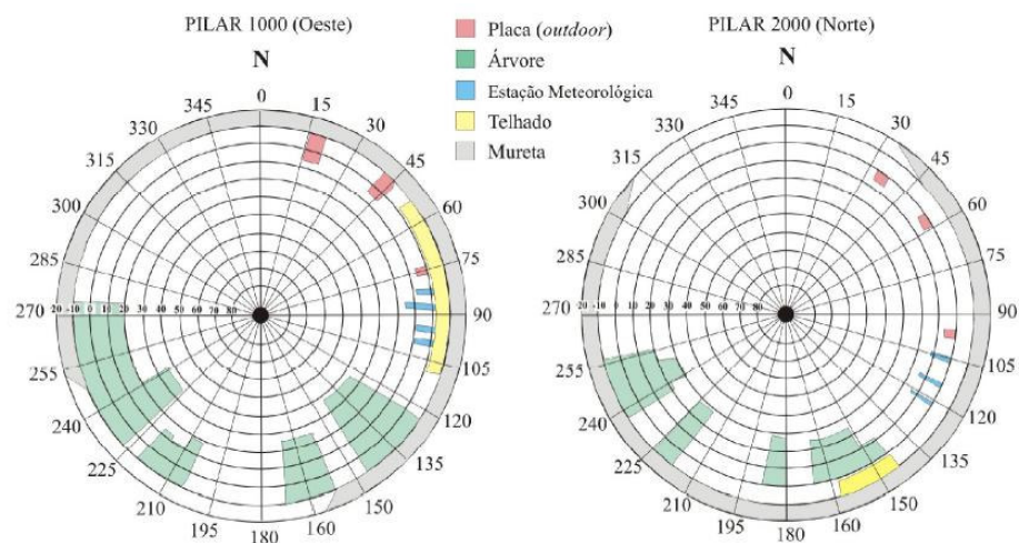
FIGURA 37 - LEVANTAMENTO DE OBSTRUÇÃO PILAR 1000 (OESTE) E PILAR 2000 (NORTE) FONTE: FREIBERGER JUNIOR (2007)
