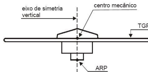
FIGURA 13-ARP, CENTRO MECÂNICO, TGP FONTE: FREIBERGER JUNIOR (2004)
