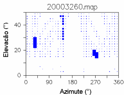
FIGURA 58 - PILAR 2000 (NORTE) – ANTENA AT 504 - DIA GPS 326-08 FONTE: A autora (2009)
