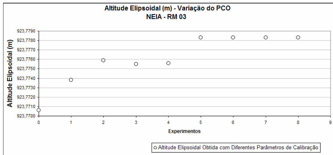
FIGURA 85 - VALORES DAS ALTITUDES ELIPSOIDAIAS EM METROS (RM03-NEIA)
