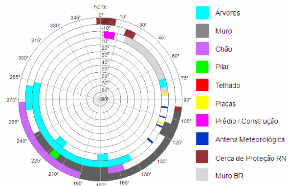
FIGURA 59 - DIAGRAMA DE OBSTRUÇÃO PILAR 2000 (NORTE) FONTE: A autora (2009)
