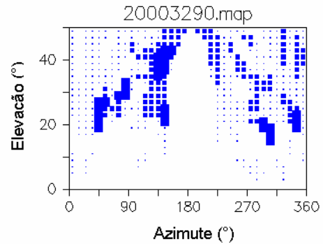
FIGURA 45 - PILAR 2000 (NORTE) - ANTENA TRM22020.00+GP - DIA GPS 329-08 FONTE: KRUEGER (2009)
