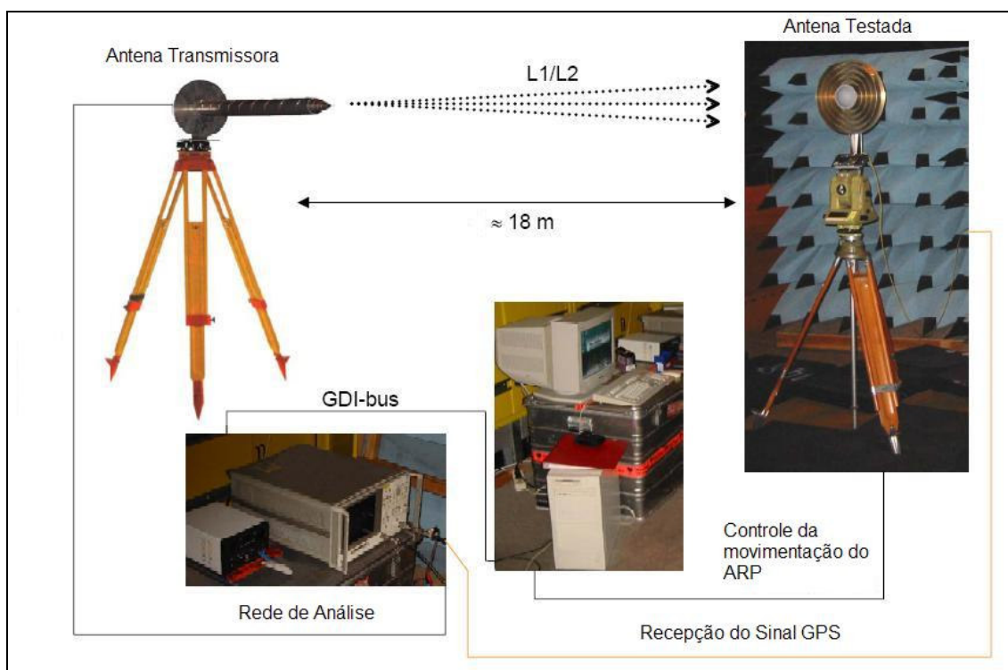
FIGURA 18 - CALIBRAÇÃO ABSOLUTA EM CÂMARA ANECÓICA FONTE: ADAPTADO DE GÓRRES ET AL., (2006)
