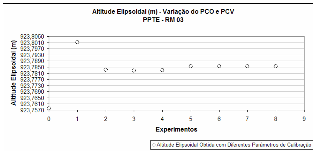
FIGURA 86 - VALORES DAS ALTITUDES ELIPSOIDAIAS EM METROS (RM03-PPTE)
