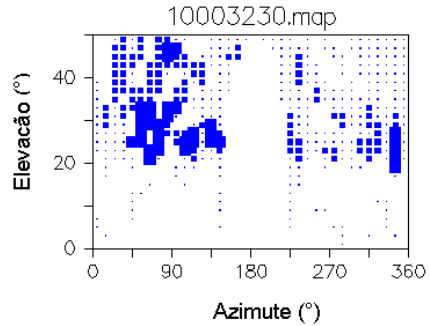
FIGURA 39 - PILAR 1000 (OESTE) - ANTENA TRM22020.00+GP- DIA GPS 323-08 FONTE: KRUEGER (2009)
