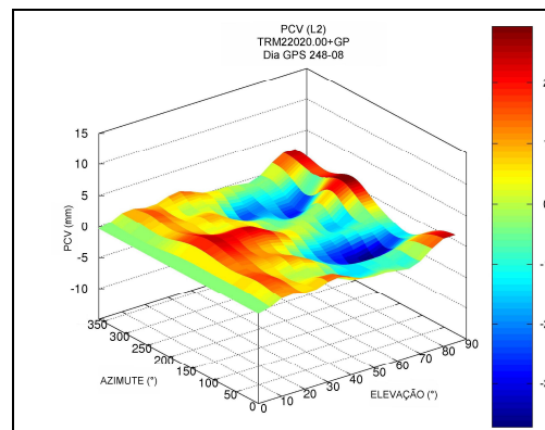
FIGURA 72 - PCV (mm) - DEPENDENTE DA ELEVAÇÃO E AZIMUTE PARA A PORTADORA L2, ANTENA TRM22020.00+GP, DIA GPS 248. FONTE: A autora (2009)
