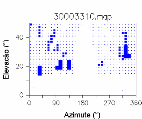
FIGURA 60 - PILAR 3000 (SUL) - ANTENA AT 504 - DIA GPS 331-08 FONTE: A autora (2009)
