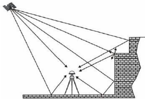
FIGURA 2 - EFEITO DE MULTICAMINHO FONTE: SOUZA et al., (2006)
