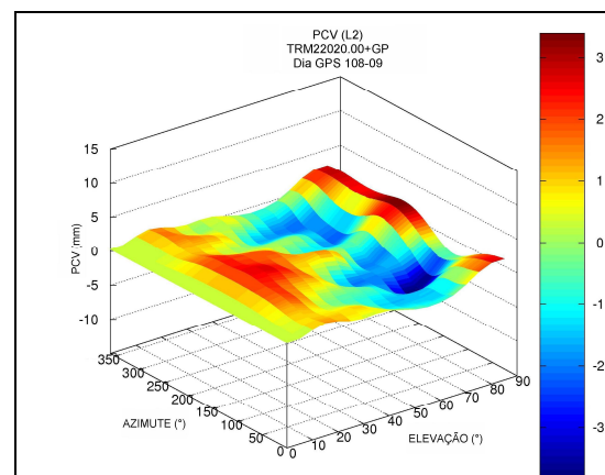
FIGURA 79 - PCV (mm) - DEPENDENTE DA ELEVAÇÃO E AZIMUTE PARA A PORTADORA L2, ANTENA TRM22020.00+GP, DIA GPS 108 FONTE: A autora (2009)
