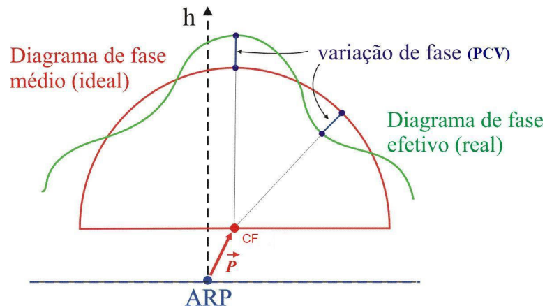
FIGURA 16-INTERPLETAÇÃO DO PCV EM FUNÇÃO DO PCO FONTE: ADAPTADO DE FREIBERGER JUNIOR (2007)
