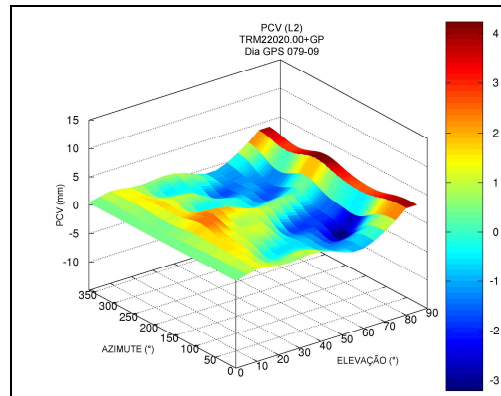
FIGURA 74 - PCV (mm) - DEPENDENTE DA ELEVÇÃO E AZIMUTE PARA A PORTADORA L2, ANTENA TRM22020.00+GP, DIA GPS 79
