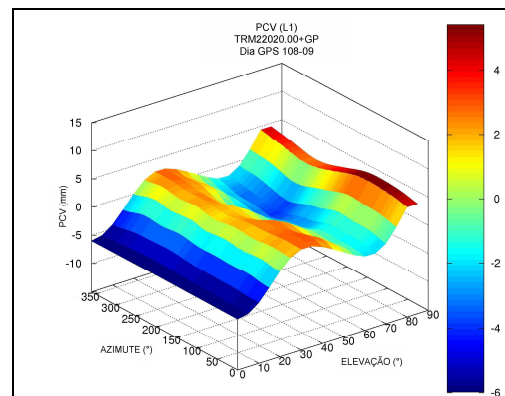
FIGURA 76 - PCV (mm) - DEPENDENTE DA ELEVÇÃO E AZIMUTE PARA A PORTADORA L1, ANTENA TRM22020.00+GP, DIA GPS 108
