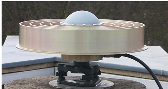
FIGURA 23 - ANTENA AOAD/M-T FONTE: GEOPP. DE (2008)
