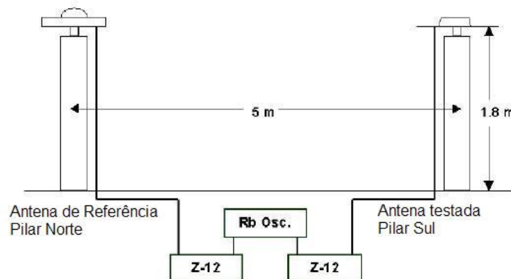
FIGURA 24 - PROCEDIMENTO DE CAMPO PARA REALIZAÇÃO DA CALIBRAÇÃO RELATIVA DE ANTENAS NO NGS
