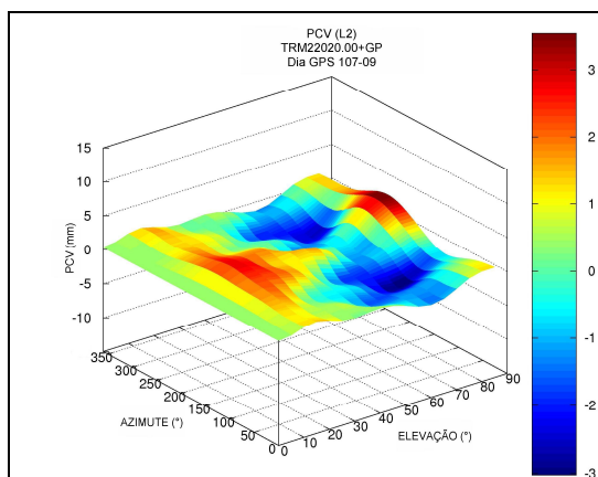
FIGURA 78 - PCV (mm) - DEPENDENTE DA ELEVAÇÃO E AZIMUTE PARA A PORTADORA L2, ANTENA TRM22020.00+GP, DIA GPS 107 FONTE: A autora (2009)
