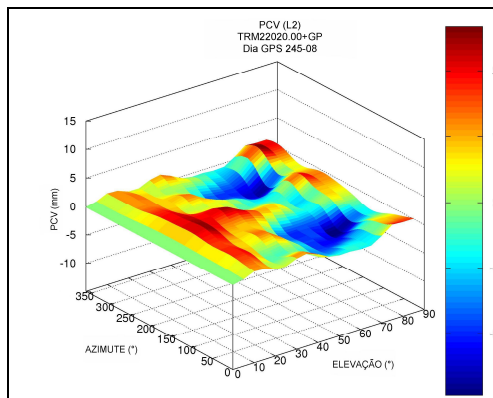
FIGURA 70 - PCV (mm) - DEPENDENTE DA ELEVAÇÃO E AZIMUTE PARA A PORTADORA L2, ANTENA TRM22020.00+GP, DIA GPS 245 FONTE: A autora (2009)
