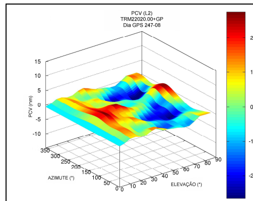
FIGURA 71 - PCV (mm) - DEPENDENTE DA ELEVAÇÃO E AZIMUTE PARA A PORTADORA L2, ANTENA TRM22020.00+GP, DIA GPS 247 FONTE: A autora (2009)
