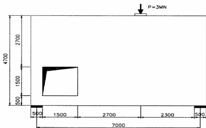
Figura 5.4.17 – Viga biapoçada com um buraco
