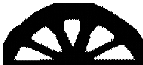
Figura 5.7 - RR= 5,5%, RRI=1%, ER=1,1%, VRI=5%,7680 elementos triangulares, Iteração 69 - malha (96x40) - SESO
