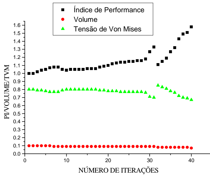
Figura 5.5.7 – Processo Evolucionário SESO
