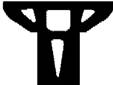
Figura 5.6.36 – RR=12,0%, RRI=1%,ER=1,5%, VRI=5%,12040 elementos triangulares, Iteração 136 – malha (170x60) - SESO
