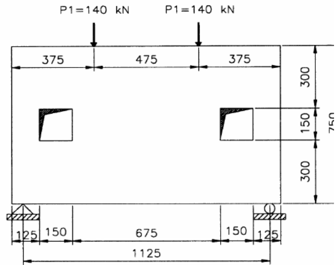
Figura 5.4.9 – Viga biapoiada com dois buracos
