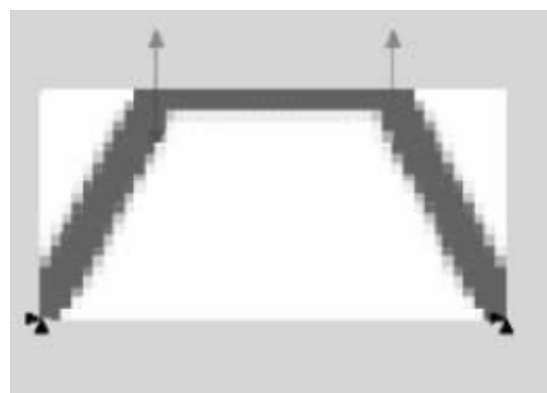
Figura 5.4.41 – Chapa biapoiada com buraco central D. Tcherniak e O. Sigmund (2001)
