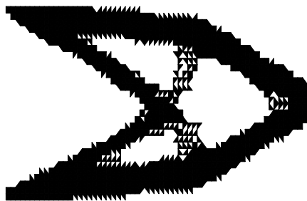
Figura 3.18 - RR= 6,5\% , ER=0,5\% , VI=40\% , VRI=1,75\% , 4798 elementos triangulares, Iteração 152 - malha (64x30) - ESO
