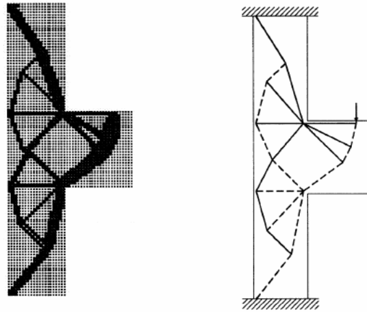
Figura 5.6.39 – Modelo de Strut-and-Tie
