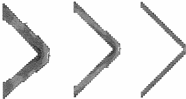
Figura 3.13 – Problema de duas barras Silva (2001).
