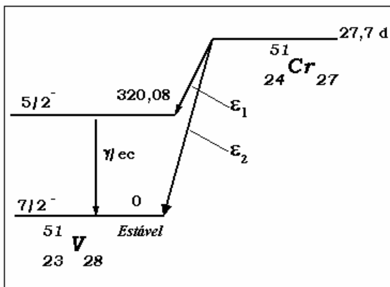
Figura 15. Esquema de decaimento do ^{51}\text{Cr} [30].
