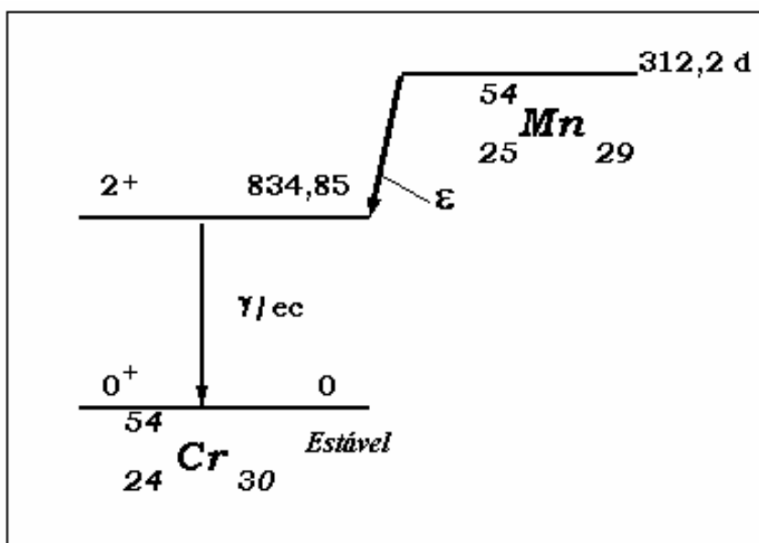
Figura 16. Esquema de decaimento do ^{54}\text{Mn} [30] .
