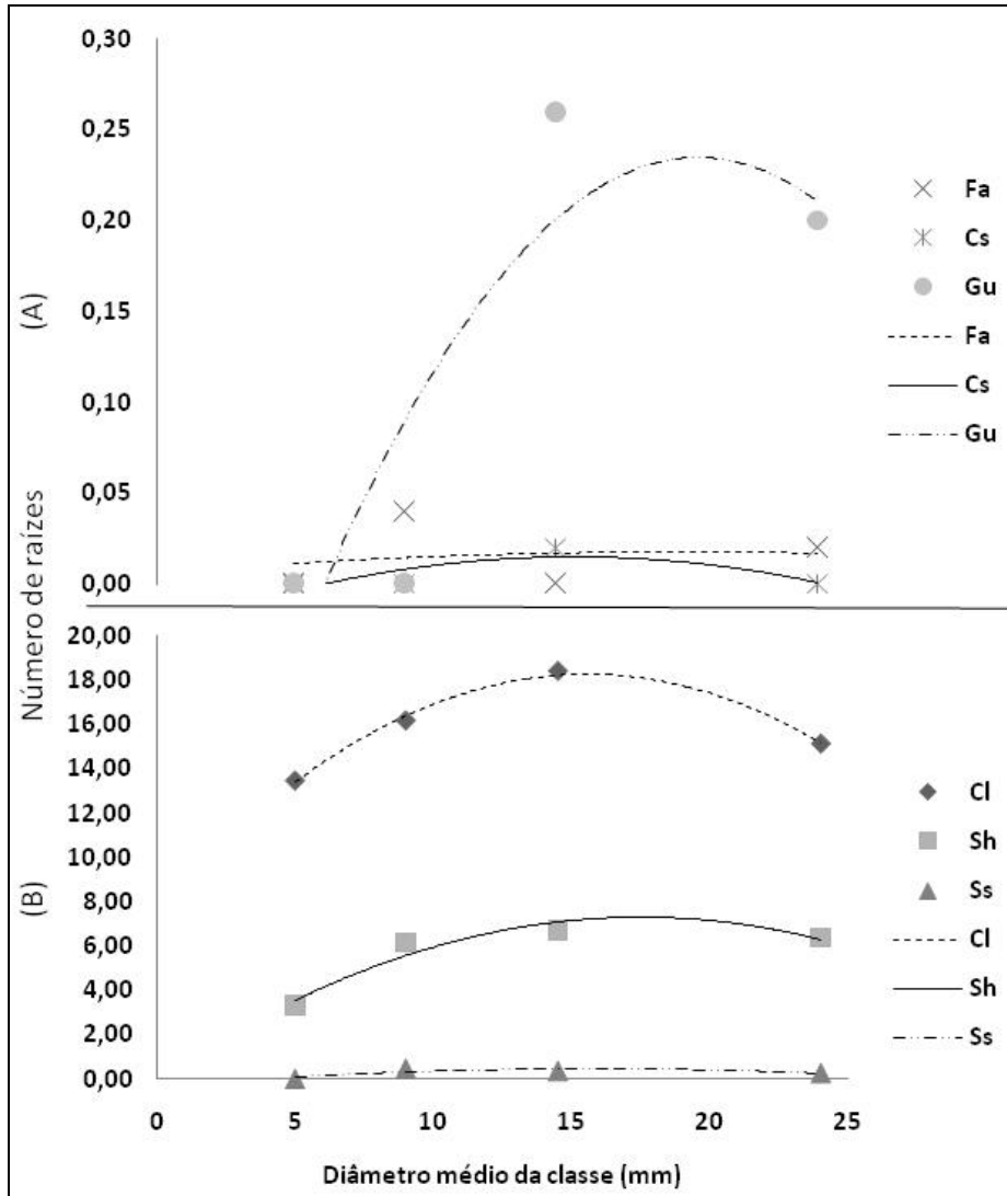
FIGURA 4 Curva do número de raízes em função do diâmetro médio das estacas. Em (A) para as espécies F. adhatodigifolia (Fa), C. silvestris (Cs) e G. ulmifolia (Gu), em (B) para as espécies C. laevigatum (Cl), S. humboldtiana (Sh) e S. scottiana (Ss).
