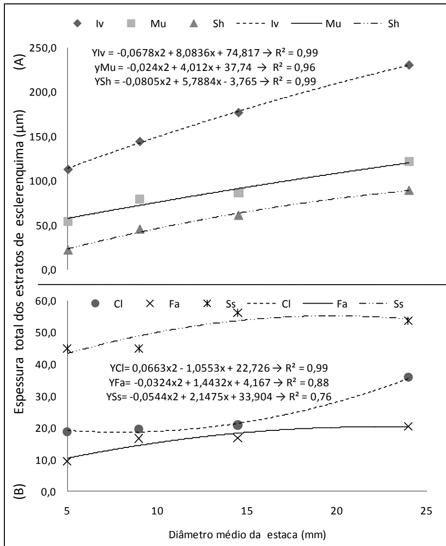
FIGURA 11 Espessura do(s) estrato(s) de tecido esclerenquimático em estacas lenhosas das espécies estudadas em função do diâmetro médio da secção analisada. Em (A) para as espécies I. vera (Iv), M. umbellata (Mu) e S. humboldtiana (Sh). Em (B) para as C. laevigatum (Cl), F. adhatodigifolia (Fa) e S. scottiana (Ss).
