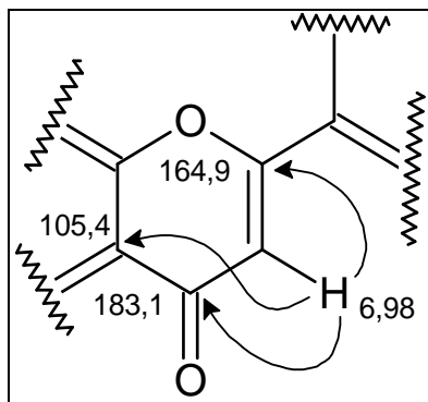
Figura 5 - Sub-estrutura I para SS1.
