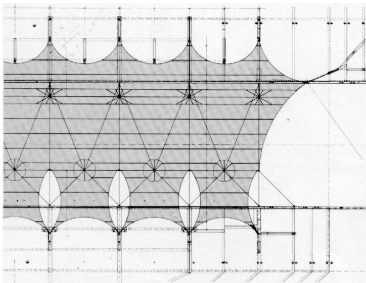
Figura 2-11 –Anexo do Schulberger Facility - Renzo Piano.
