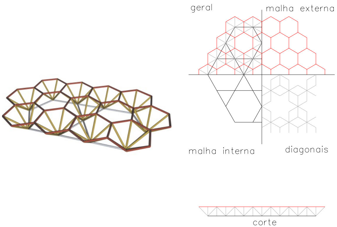
Treliça proposta.
