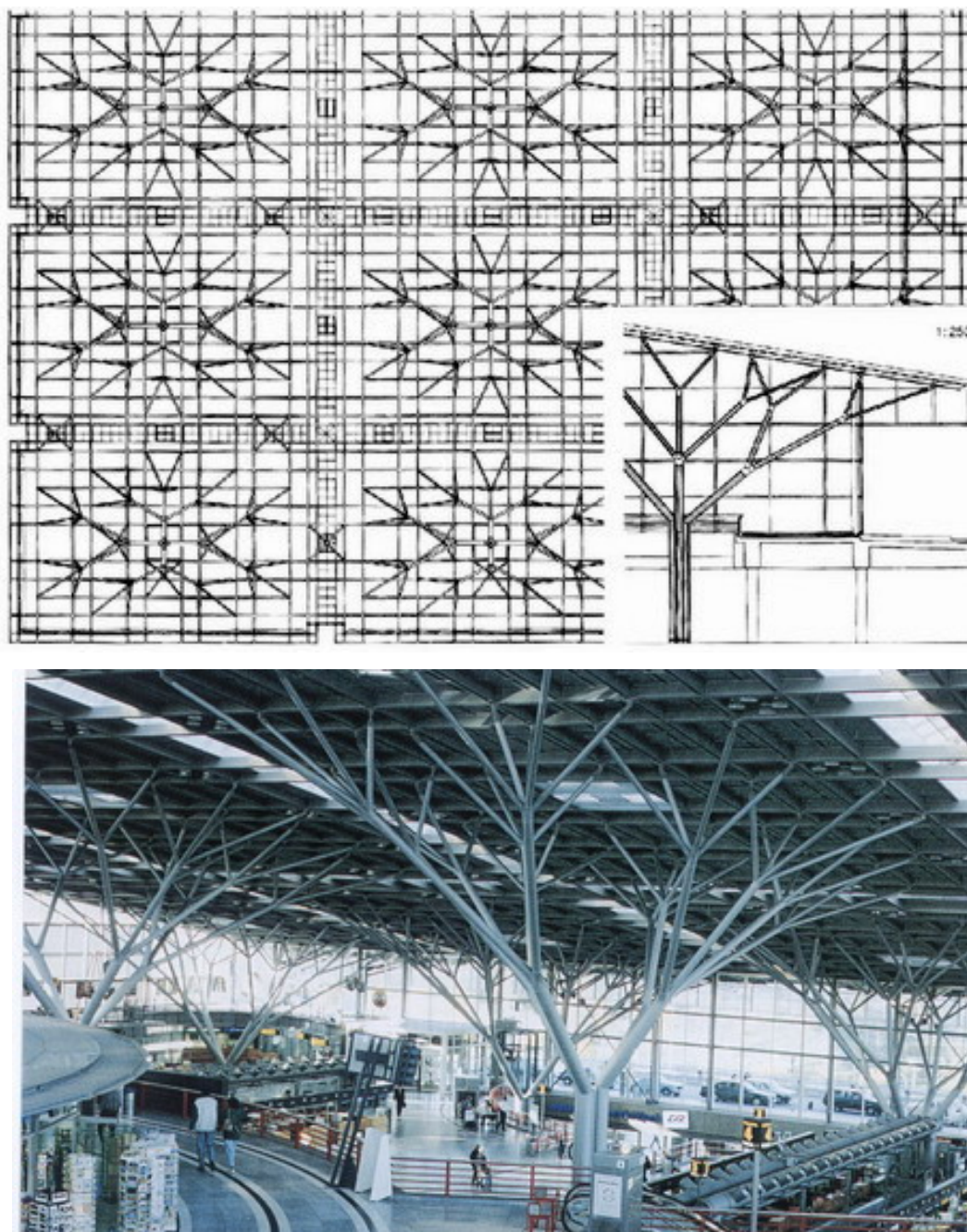
Figura 3-23 – Aeroporto de Stutgard.
