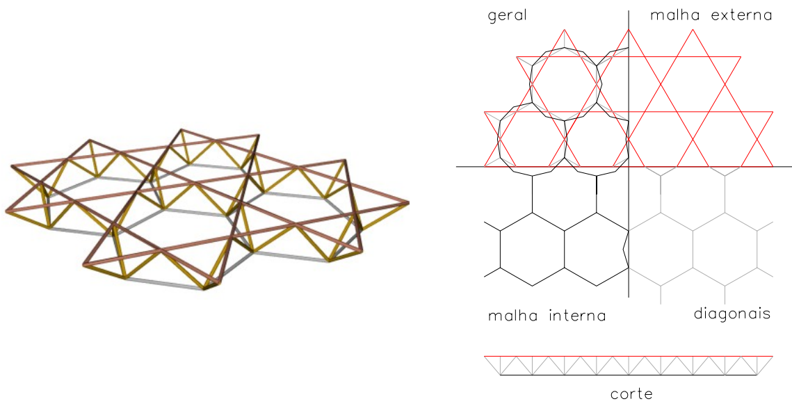
Treliça proposta.
