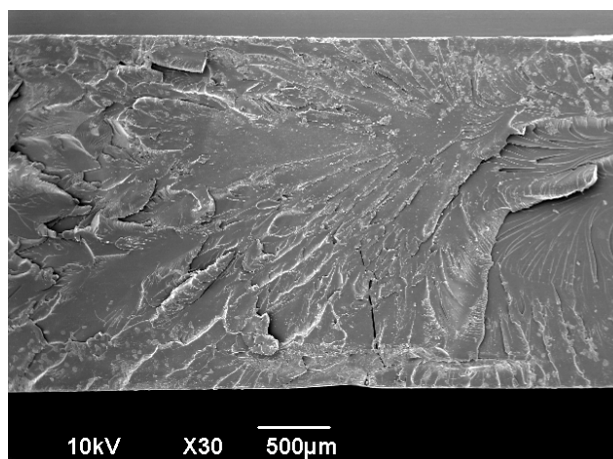
Figura 37 – Micrografia de um corpo-de-prova de resina epóxi fraturado em ensaio de tração.
