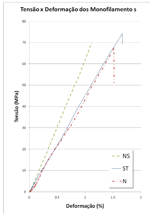
Figura 33 – Curvas representativas de resistência à tração dos monofilamentos.
