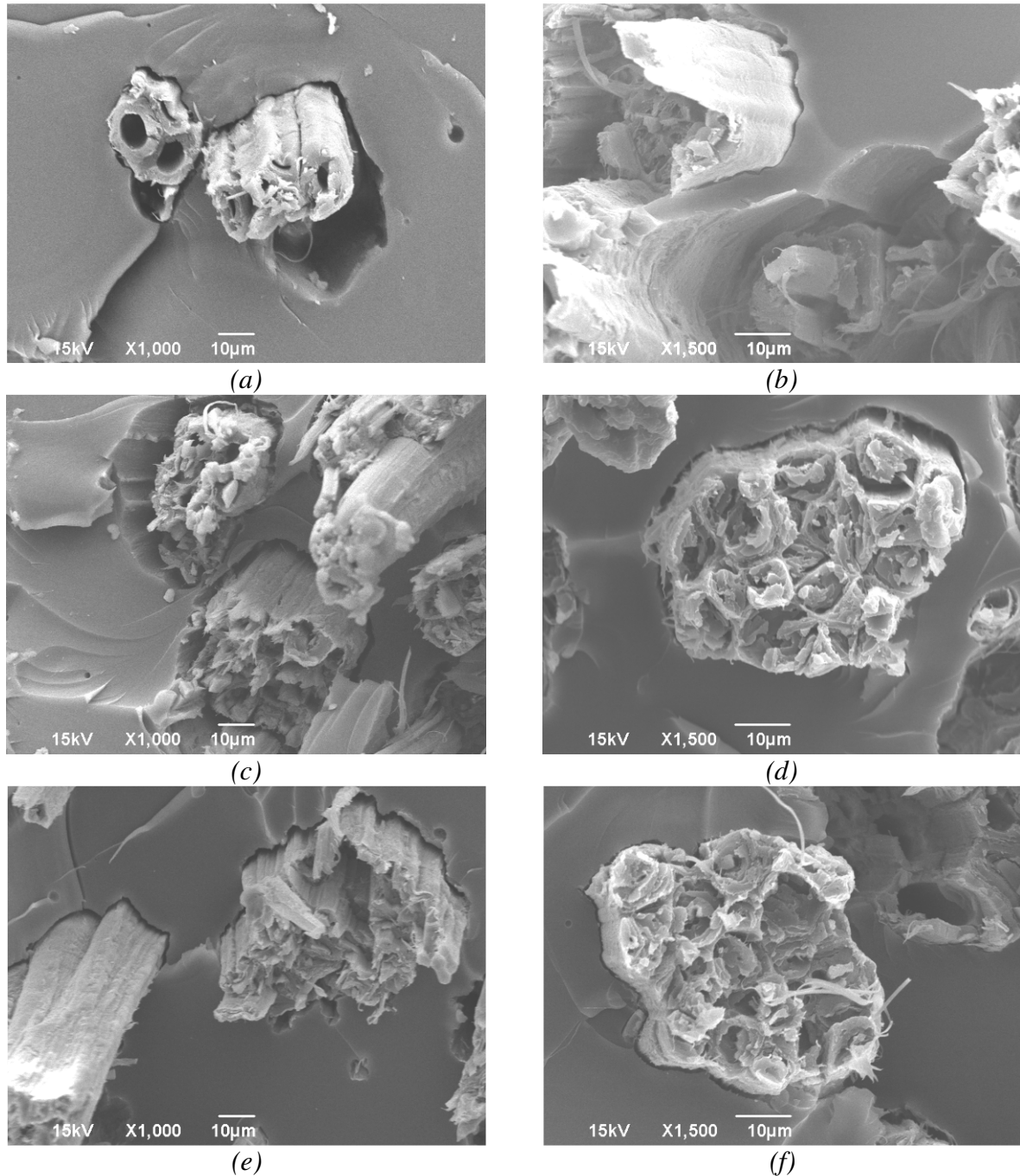
Figura 41 – MEV dos compósitos juta/epóxi do ensaio de flexão – análise da interface fibra/matriz. Compósito com fibras sem tratamento (a) e (b), com fibras tratadas com hidróxido de sódio (c) e (d) e com fibras tratadas via NaOH e agente silano (d) e (f).
