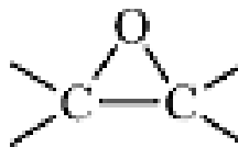
Figura 8 – Grupo epóxi.
