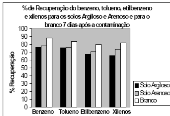
Figura 6 - Recuperação (%) de benzeno, tolueno, etilbenzeno e xilenos nos solos argiloso e arenoso e para o branco, após sete dias de contaminação (MELQUIADES et al., 2006).
