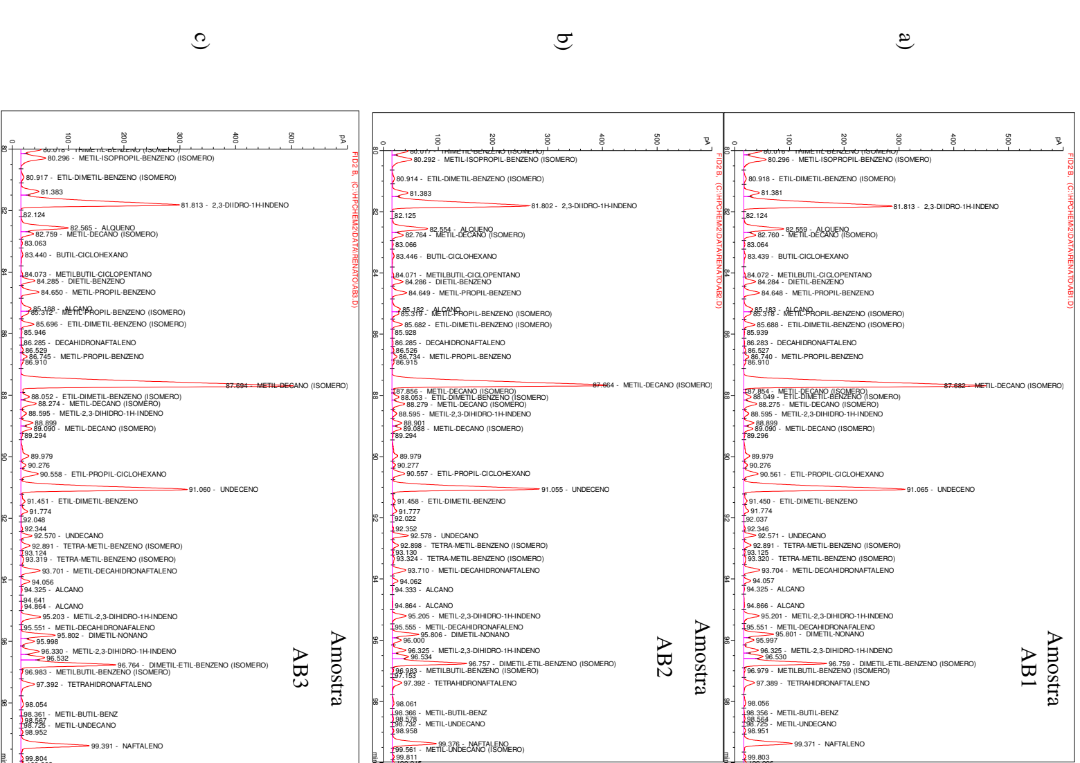
Figura 13 – Faixa de 80 a 100 minutos do cromatograma da amostra AB1 (a); AB2 (b) e AB3 (c)
