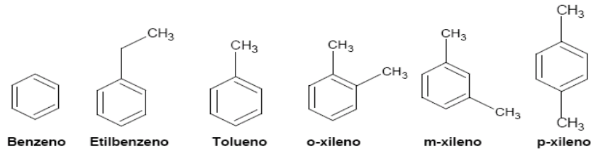
Figura 2 - Estrutura química dos contaminantes aromáticos da gasolina, denominados de BTEX (CARDOSO, 2007)
