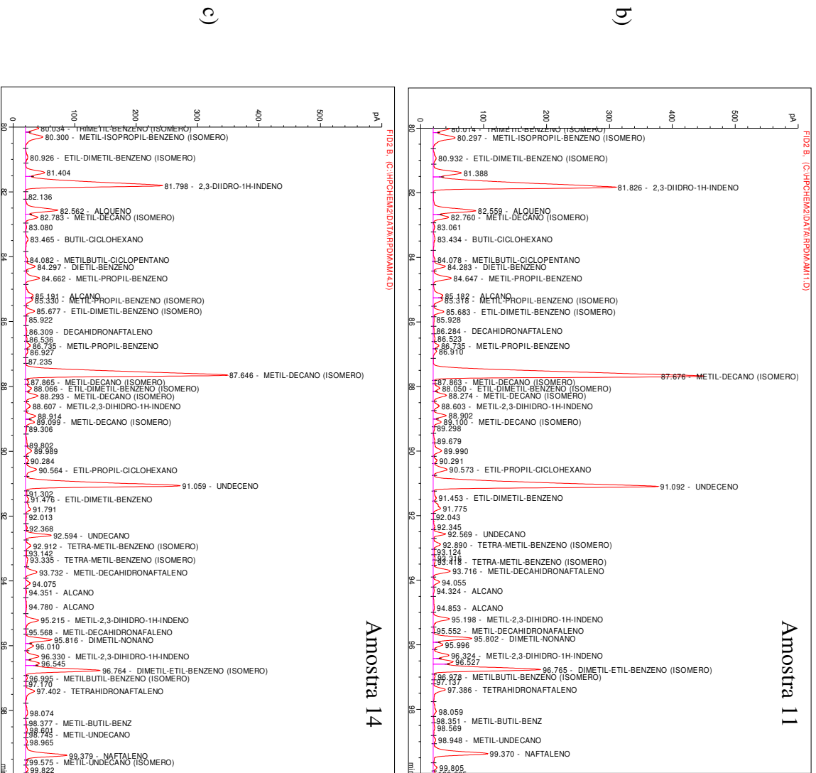
Figura 15 – Faixa de 80 a 100 minutos do cromatograma da amostra 7 (a); 11 (b) e 14 (c)
