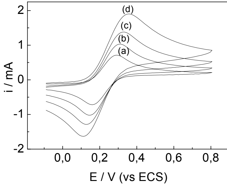
Figura 1.13: Voltamogramas cíclicos do CPV em solução 0,04 \text{ mol L}^{-1} de \text{K}_3[\text{Fe}(\text{CN})_6] e 1,0 \text{ mol L}^{-1} de \text{KCl} , v = 20 (a) , 50 (b) , 100 (c) e 200 \text{ mV s}^{-1} (d).
