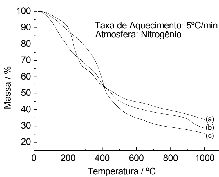
Figura 2.1: Curvas das análises termogravimétricas de: Resina-Fe (a); Resina-Cr (b); Resina-Ce (c).
