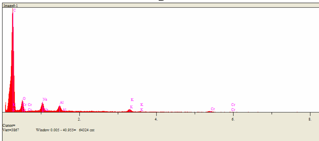
Figura 2.6: Espectro de energia dispersiva de Raios-X do: CPV-Fe (A), CPV-Ce (B) e CPV-Cr (C).
