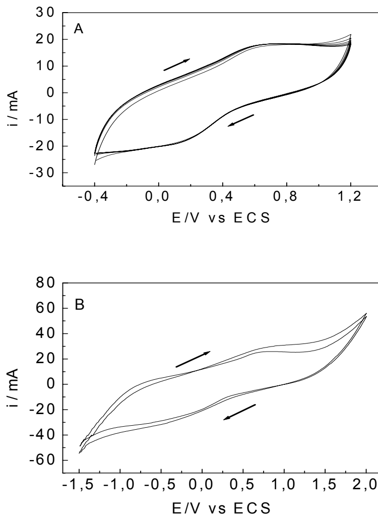
Figura 2.10: Voltamogramas cíclicos do CPV-Fe: ativado em 90s a 2,25V vs ECS, 15 ciclos em \text{H}_2\text{SO}_4 0,5\text{mol.L}^{-1} (A), em \text{H}_2\text{SO}_4 0,5\text{mol.L}^{-1} (B) a v = 100 \text{ mV s}^{-1} .
