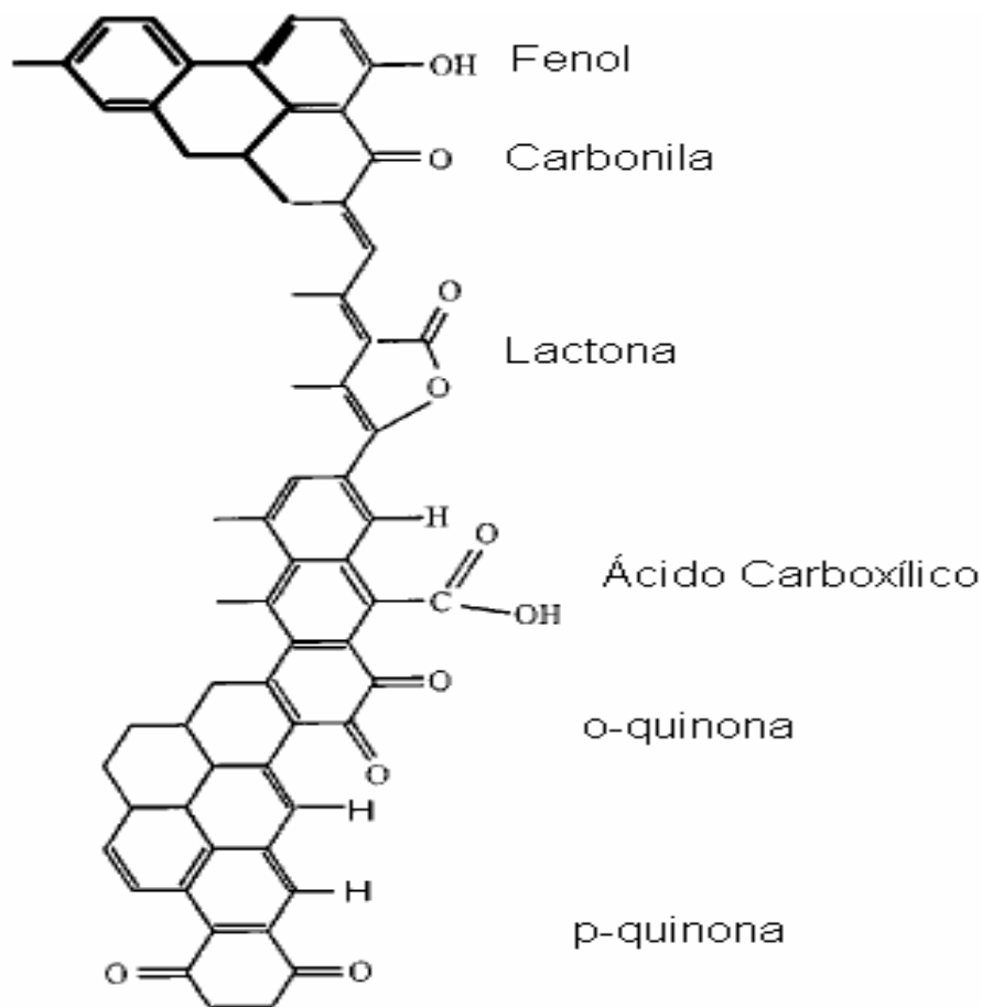
Figura 1.5: Várias possibilidades de grupos funcionais contendo oxigênio que podem estar presentes sobre a superfície de materiais de carbono [4].
