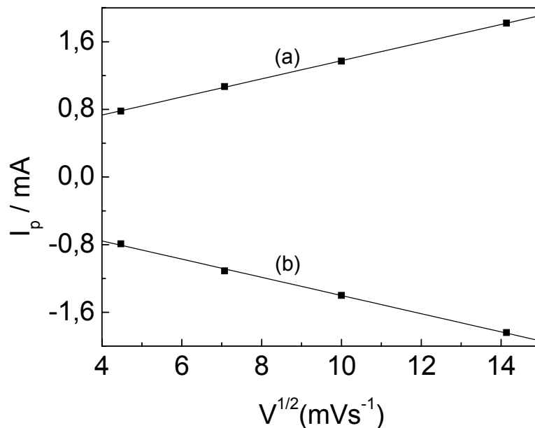
Figura 1.14: Relação entre i_{p_c} e i_{p_a} com a velocidade de varredura nos voltamogramas da Figura 1.14: i_{p_c} (a); i_{p_a} (b).
