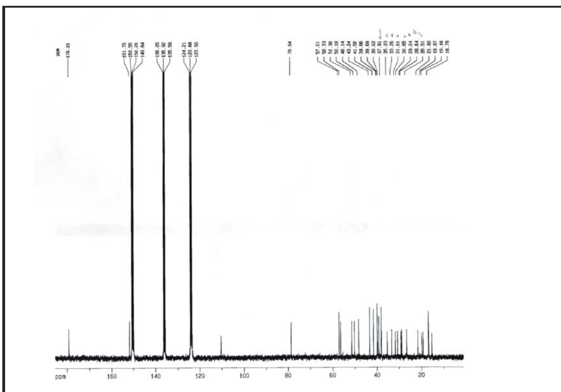
Figura 77: Espectro de RMN ^{13}\text{C} de LA-SU-09.
