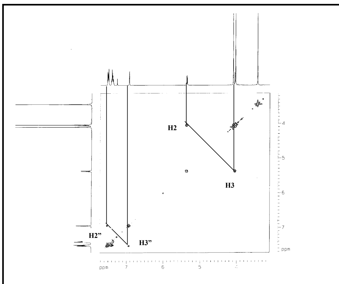
Figura 42: Espectro RMN COSY de LA-SU-05.
