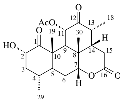
11-Acetilamarolida
