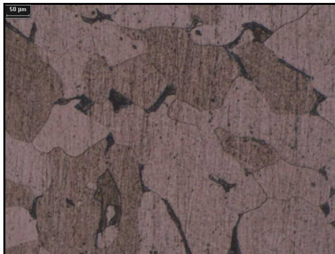
Figura 9. Micrografias ópticas da microestrutura do aço carbono 1008 após revelação da estrutura com reagente de Nital 2%. Aumento de 200X.
