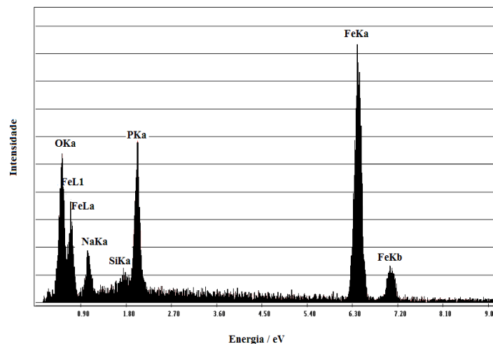
Figura 17. Espectro de EDS para o ponto branco no aço 1008 contendo PFe/BTAH.
