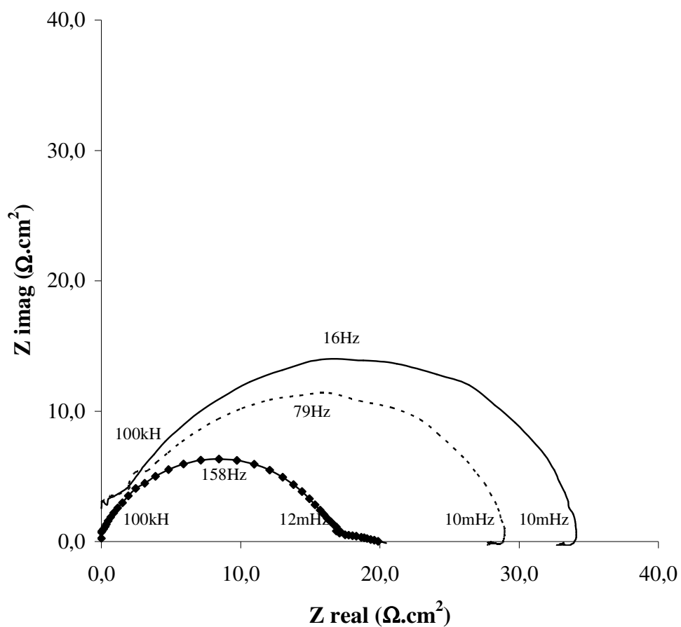
Figura 33. Diagramas de Nyquist do aço carbono 1008: (—◆—) polido, (---) com PFe, (—) com PFe/BTAH, em meio de H_2SO_4 0,1 \text{ mol L}^{-1} .
