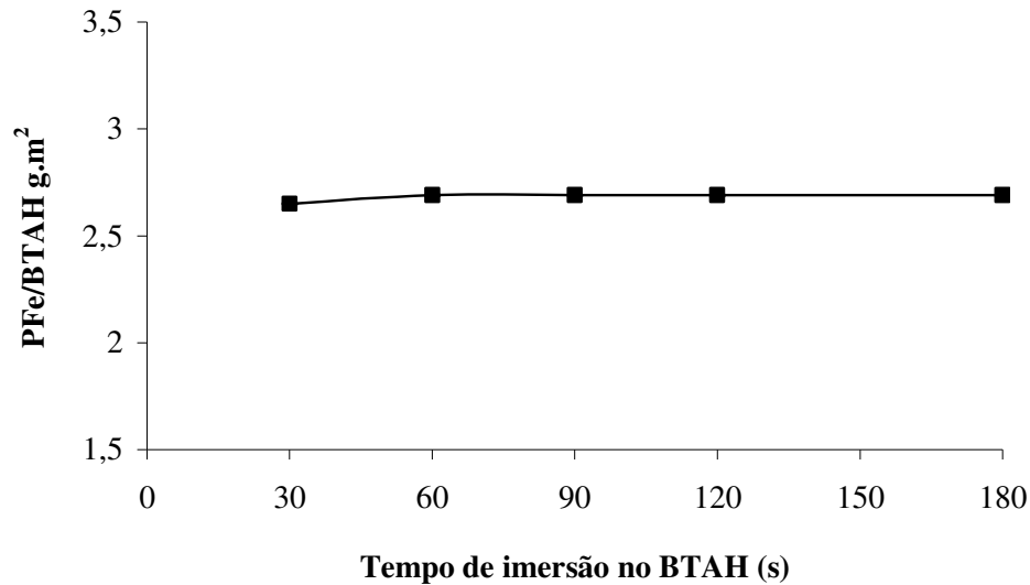
Figura 12. Variação média da massa de PFe/BTAH na superfície do aço carbono 1008 em função do tempo de imersão no banho inibidor de BTAH.
