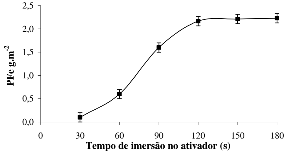
Figura 10. Variação média da massa de PFe na superfície do aço carbono 1008 em função do tempo de imersão no ativador.
