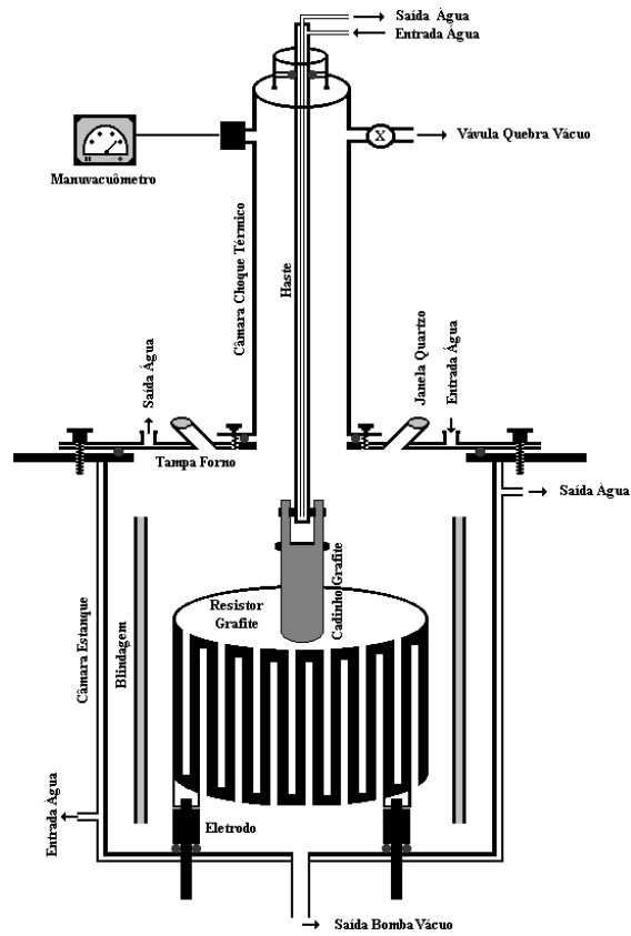
Figura 5.2. Diagrama esquemático da câmara de fusão do forno a vácuo.
