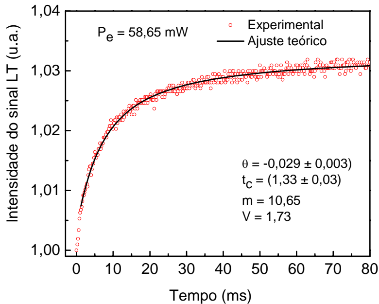
Figura 6.9: Transiente de LT para o vidro dopado com 2% de \text{Yb}_2\text{O}_3 determinado com a amostra em temperatura ambiente. P_e = 58,65 mW e \lambda_{\text{ex}} = 976 nm.
