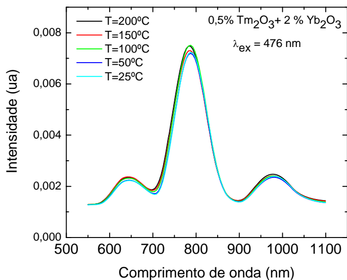
Figura 6.21. Espectro de emissão em função da temperatura da amostra dopada com 2% de \text{Yb}_2\text{O}_3 e 0,5% \text{Tm}_2\text{O}_3 com excitação em \lambda_{\text{ex}} = 476 nm.
