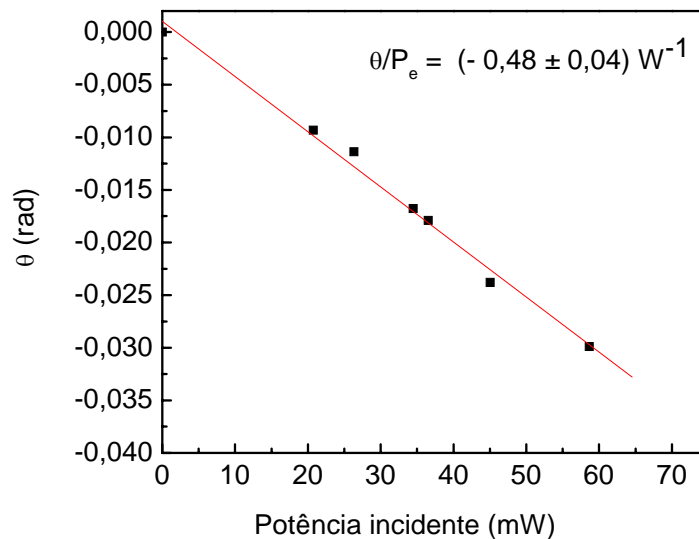
Figura 6.10. Valores do parâmetro \theta em função da potência do laser de excitação em \lambda=976 nm para amostra de LSCAS dopada com 2% \text{Yb}_2\text{O}_3 .
