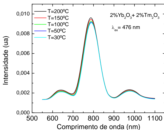
Figura 6.22. Espectro de emissão em função da temperatura da amostra dopada com 2% \text{Yb}_2\text{O}_3 e 2,0% \text{Tm}_2\text{O}_3 com excitação em \lambda_{\text{ex}} = 476 nm.
