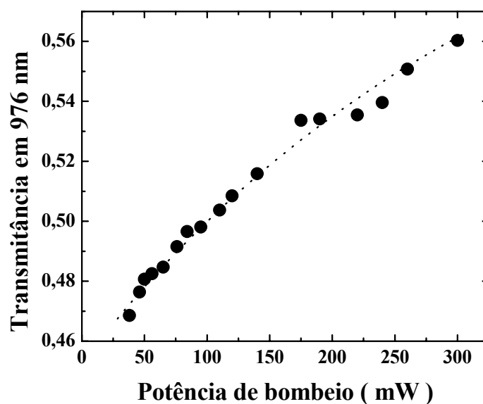
Figura 8.4 : Transmitância em função da potência de bombeio para a amostra co-dopada com 2% de \text{Yb}_2\text{O}_3 e 0,5% de \text{Tm}_2\text{O}_3 .
