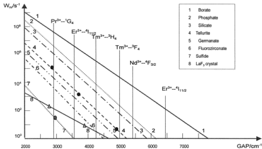
Figura 7.4. Taxa de relaxação por multifonons de níveis excitados de íons terras raras em várias matrizes vítreas em função do intervalo dos níveis de energia [1].
