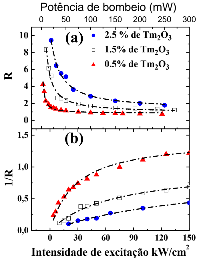
Figura 8.6 - Razão das emissões devido à conversão ascendente de energia. (a) R = \frac{I(800\text{nm})}{I(480\text{nm})} e (b) \frac{1}{R} , ambas em função da potência de bombeio.
