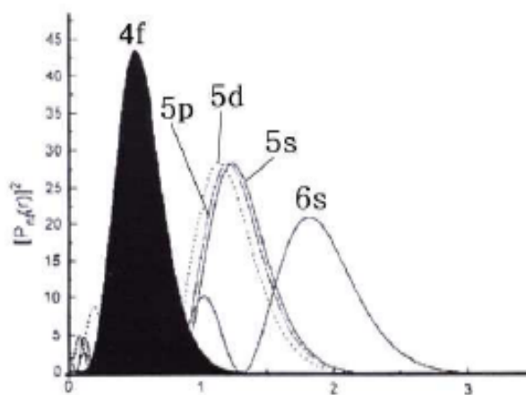
Figura 3.7 Distribuição de probabilidade radial dos elétrons em função da distancia ao núcleo do átomo de Yb para os orbitais 4f, 5d, 5p e 6s. [21]
