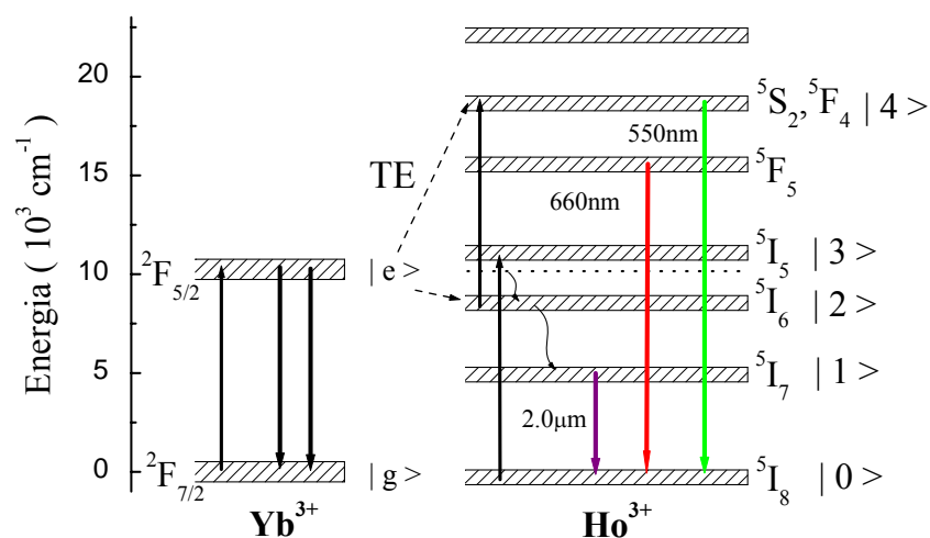
Figura 9.2 diagrama simplificado de níveis do sistema Yb^{3+} - Ho^{3+} .
