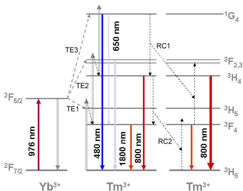
Figura 8.2. Diagrama de níveis simplificado para o sistema \text{Yb}^{3+}/\text{Tm}^{3+} mostrando o processo de transferência de energia, as emissões e o processo de relaxação cruzada de energia, com bombeio no comprimento de onda de 976 nm.
