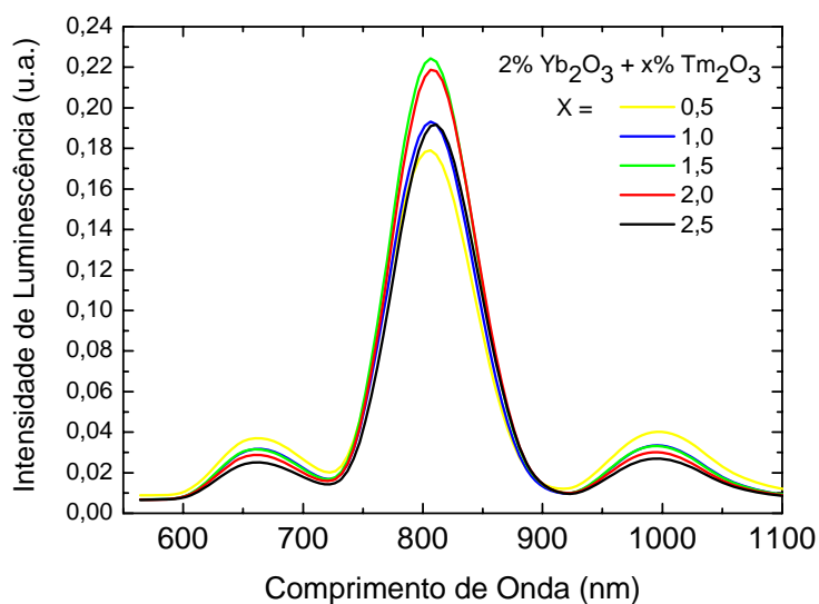
Figura 6.16. Intensidade de luminescência normalizada pela espessura das amostras co-dopadas com 2% de Yb_2O_3 e diferentes concentrações de Tm_2O_3 com excitação em 476 nm.
