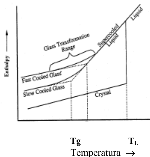
Figura 3.3 Processos de cristalização e vitrificação em função da temperatura [11].
