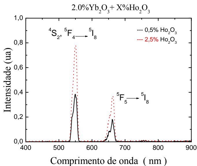
Figura 9.3 Espectro de emissão no visível do íon Ho 3+ com excitação em \lambda=976 nm.
