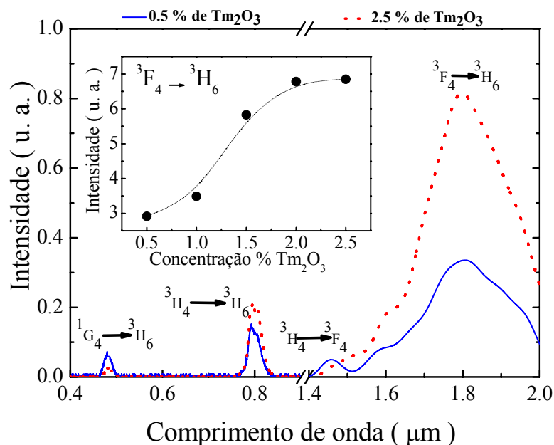
Figura 7.3 – espectro de emissão luminescente do íon Tm^{3+} nas amostras co-dopadas com 2% de Yb_2O_3 e 0,5 e 2,5 % de Tm_2O_3 . O bombeio foi em \lambda = 976 nm e a intensidade de emissão no comprimento de onda de \lambda = 1,8 \mu m , devido à transição {}^3F_4(Tm^{3+}) \rightarrow {}^3H_6(Tm^{3+}) . O diagrama interno mostra o aumento dessa emissão em função da concentração Tm_2O_3 .
