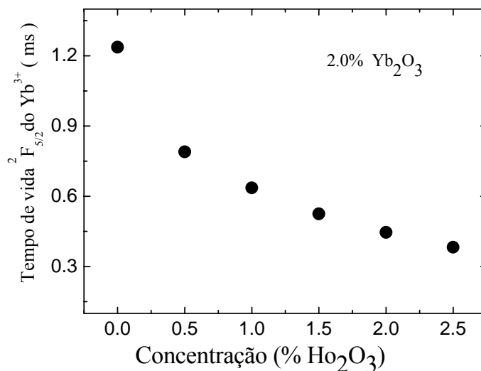
Figura 9.4 Tempos de vida do nível ^2F_{5/2}(Yb^{3+}) em função da concentração de Ho 2 O 3 .
