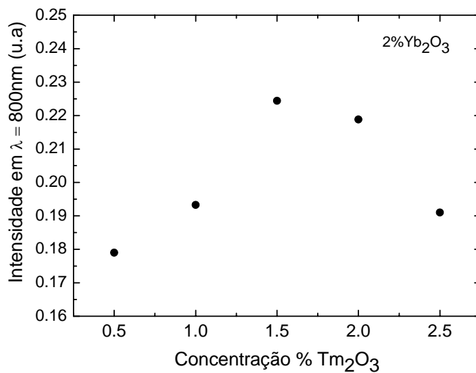
Figura 6.17. Intensidade de luminescência em \lambda=800nm normalizada pela espessura das amostras dopadas com 2% Yb_2O_3 e diferentes concentrações de Tm_2O_3 , excitado em 476 nm.
