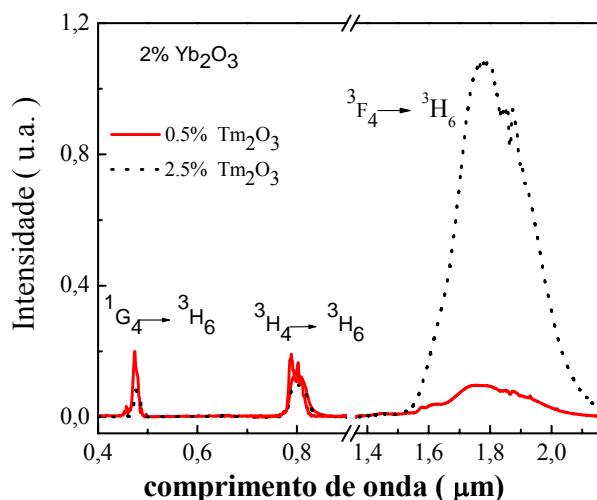
Figura 7.1, Espectro de luminescência das amostras dopadas com 2,0% de \text{Yb}_2\text{O}_3 e com 0,5 e 2,5 % de \text{Tm}_2\text{O}_3 com excitação em \lambda = 976 \text{ nm} .
