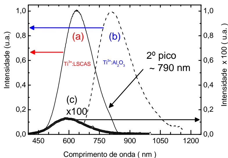
Figura 9.8 Comparação entre as bandas de emissão do cristal \text{Ti}^{3+}:\text{Al}_2\text{O}_3 e do vidro \text{Ti}^{3+}:\text{LSCAS} .
