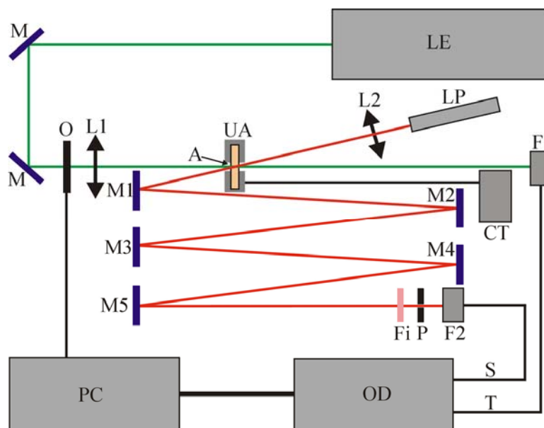
Figura 5.6. Configuração experimental. Em que: LE é o laser de excitação; LP é o laser de prova; M_i são espelhos; O é o obturador; L1 e L2 são lentes convergentes; A é a amostra; F1 é um filtro que permite a passagem da luz do laser de prova; P é um orifício com aproximadamente 2,0 mm de diâmetro; F1 e F2 são fotodiodos; S é o cabo do sinal de lente térmica; T é o cabo do sincronizador de sinal; OD é o osciloscópio; PC é um microcomputador; CT é o controlador de temperatura e UA a unidade de aquecimento.
