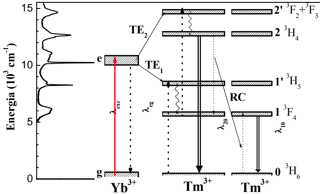
Figura 7. 6 diagrama de níveis de energia simplificado do sistema \text{Yb}^{3+}/\text{Tm}^{3+}
