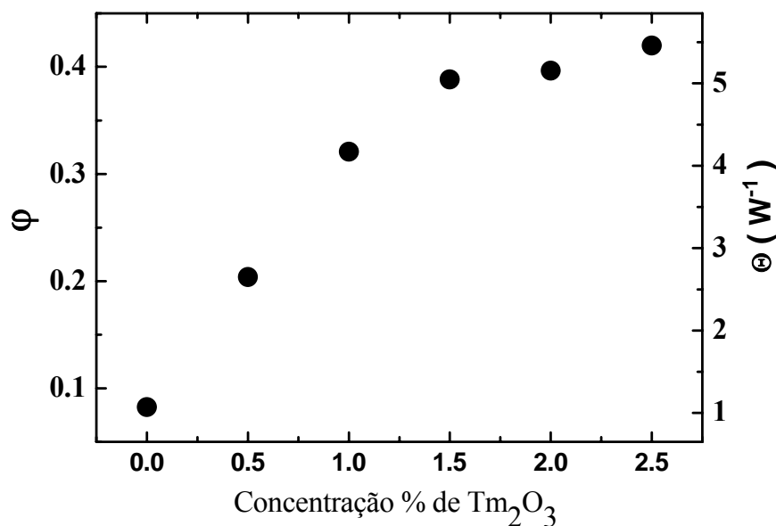
Figura 7.5 Carga térmica \phi experimental
