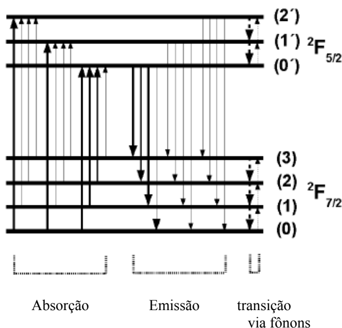
Figura 3.6. Diagrama de níveis de energia do íon \text{Yb}^{3+} .
